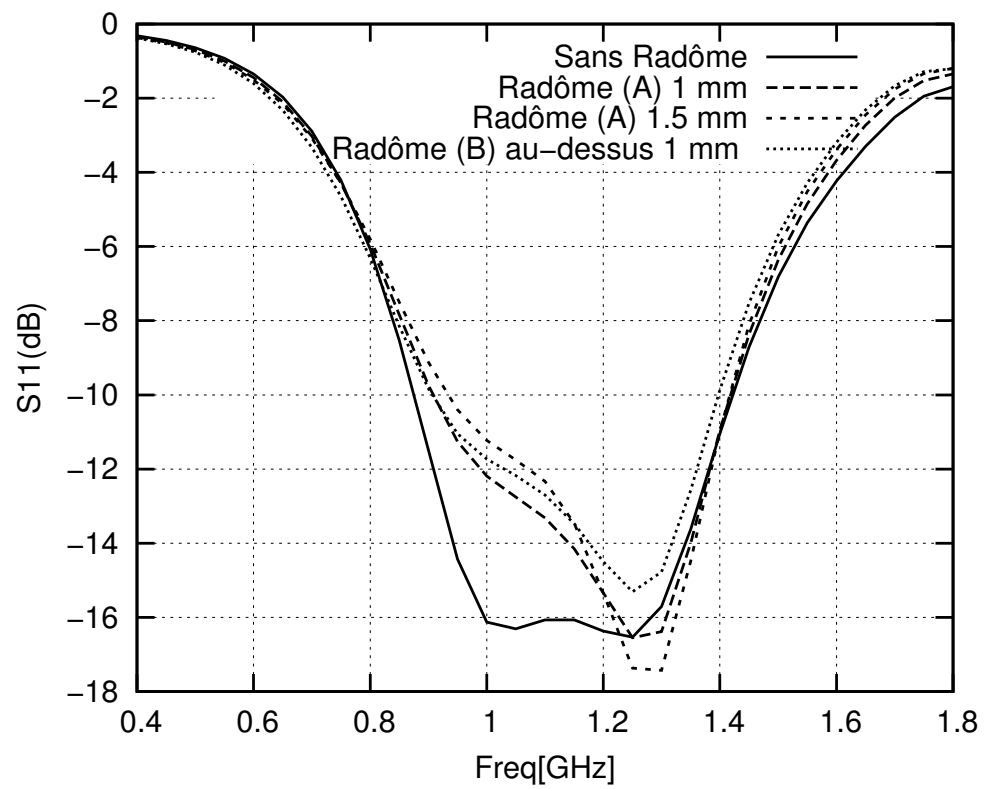
Figure 4.17 S_{11} pour différentes épaisseurs de radôme
