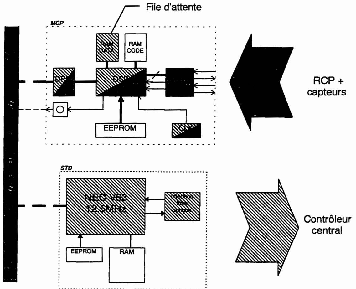
Figure 5.10: Combinaison du STD et MCP
