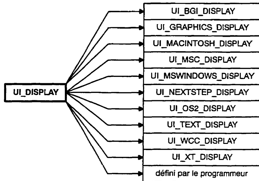
Figure 7.25: Définition de la classe abstraite UI_DISPLAY
