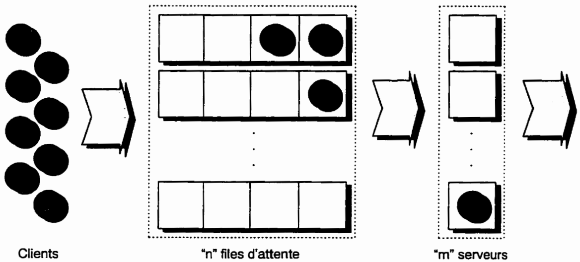
Figure I.3: Fonctionnement général d'un système temps réel à contraintes douces
