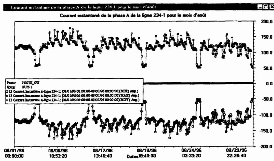
Figure 7.14: Graphique avec légende
