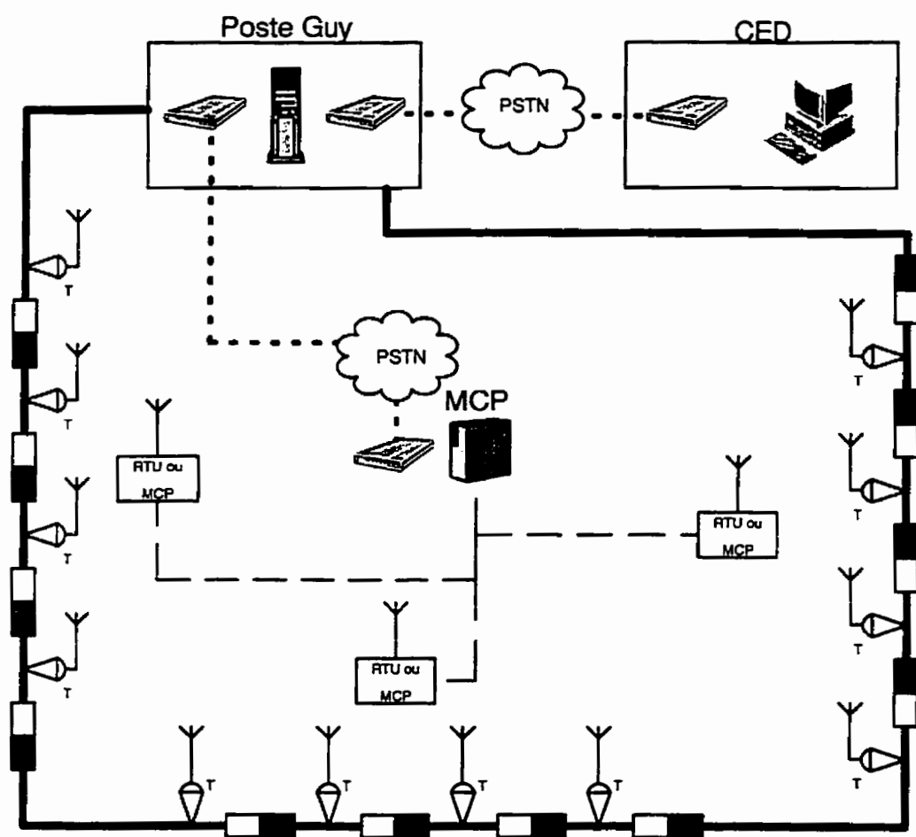
Figure 4.4: Implantation de la seconde phase du projet avec indicateurs radio
