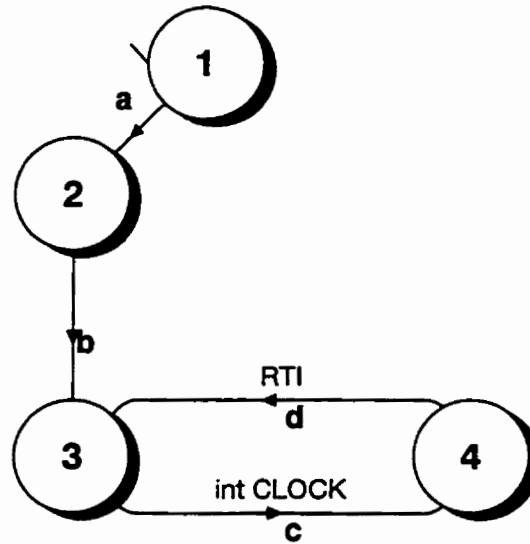
Figure 5.3: Diagramme de transition d'états du processeur MCP
