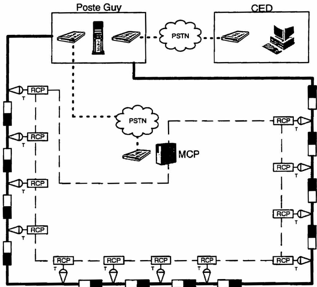
Figure 4.3: Implantation de la seconde phase du projet avec fibres optiques
