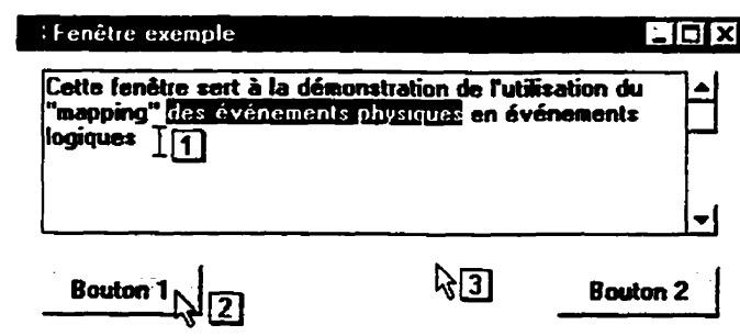
Figure 7.23: Mappage des événements physiques en événements logiques
