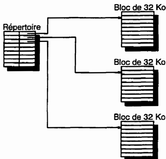
Figure 7.34: Solution au problème de mémoire sous Windows 16 bits
