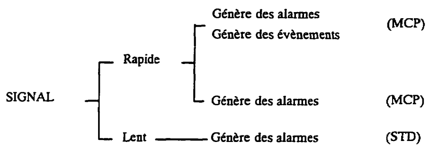
Figure 3.2: Hiérarchie des données dans le système de télésignalisation
