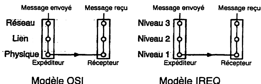
Figure 6.2: Comparaison de l'architecture du protocole avec le protocole OSI
