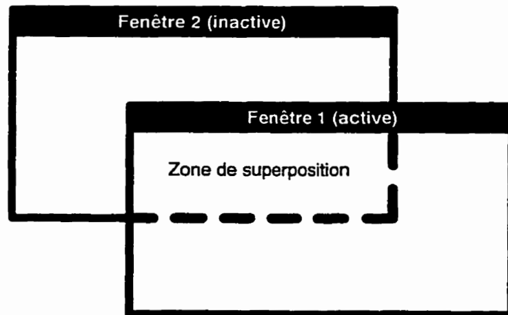
Figure 7.24: Passage de message aux fenêtres selon leur priorité
