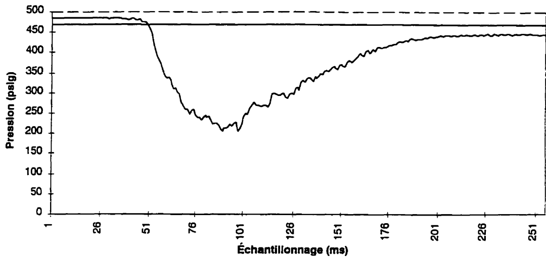
Figure 3.1: Courbe de pression d'ouverture d'une tête de disjoncteur à air
