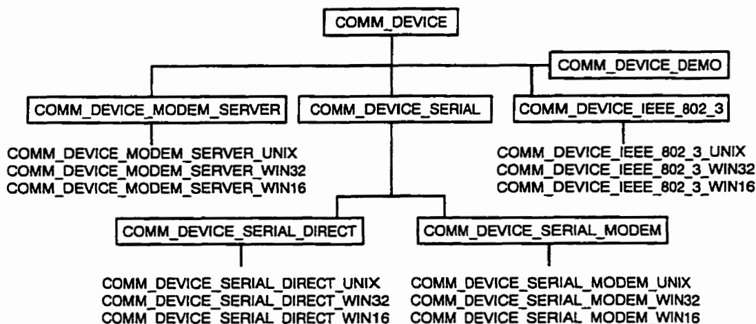
Figure 7.32: Hiérarchie des classes utilisées pour la communication
