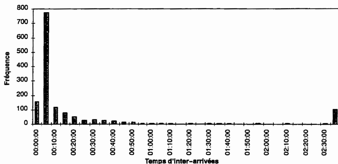
Figure I.1: Temps d'inter-arrivée des données originelles
