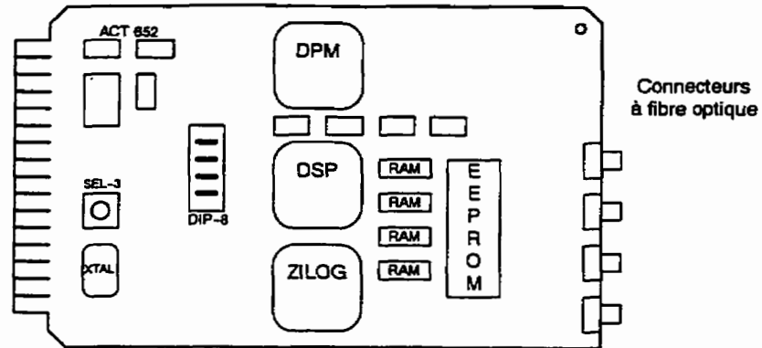
Figure 5.1: Carte MCP - disposition du DSP et de ses composants
