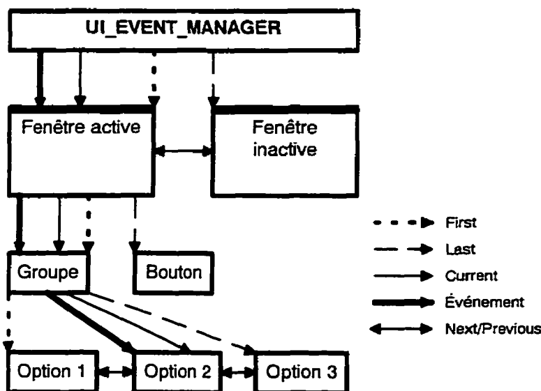
Figure 7.27: Traitement de l'exemple de l'architecture descendante
