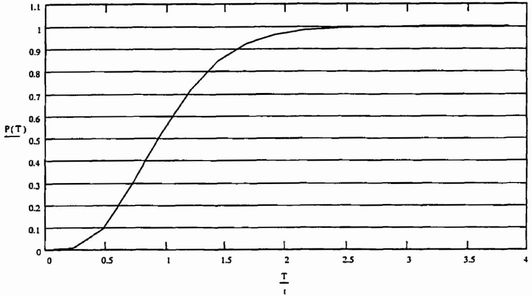
Figure I.6: Distribution Erlang 5 pour le système de surveillance
