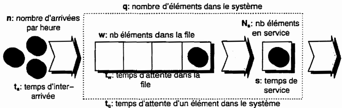
Figure I.4: Configuration du système temps réel étudié
