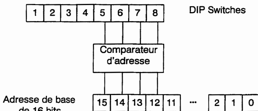
Figure 5.9: Utilisation des “DIP Switches” pour la mémoire à 2 ports
