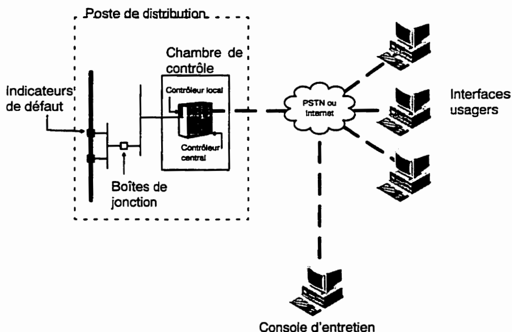
Figure 2.1: Architecture globale du système de télésignalisation
