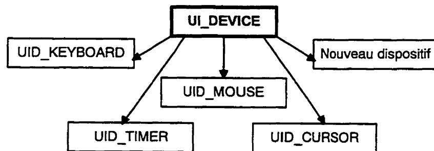
Figure 7.22: Définition de la classe abstraite UI_DEVICE
