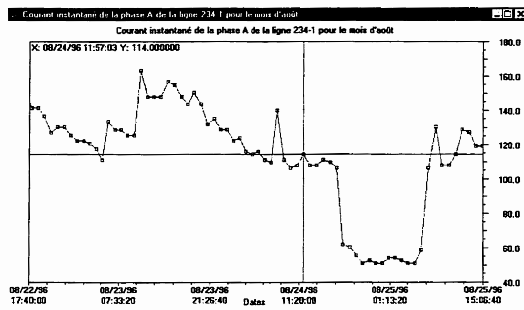
Figure 7.16: Extrapolation des graphiques de tendances
