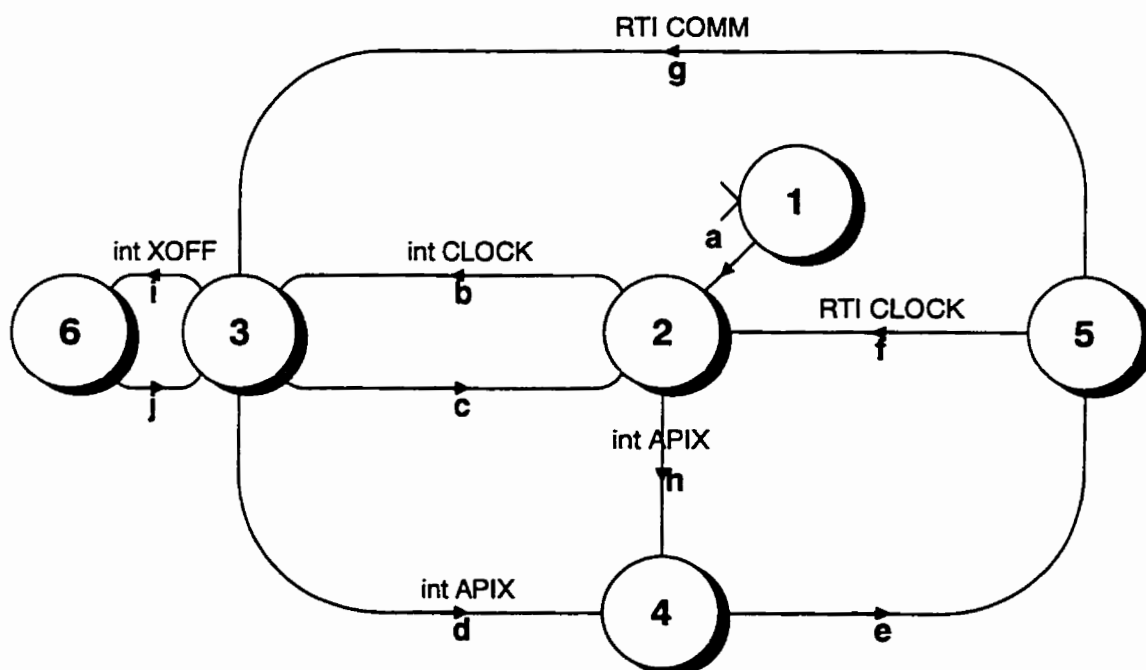
Figure 5.6: Diagramme de transition d'états du processeur STD
