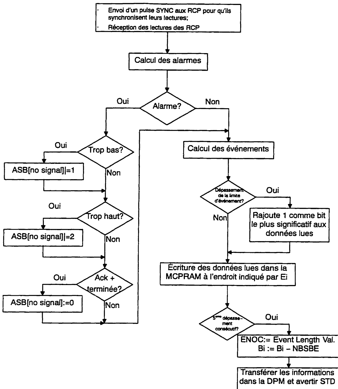
Figure 5.4: Gestion de l'interruption interne du processeur MCP
