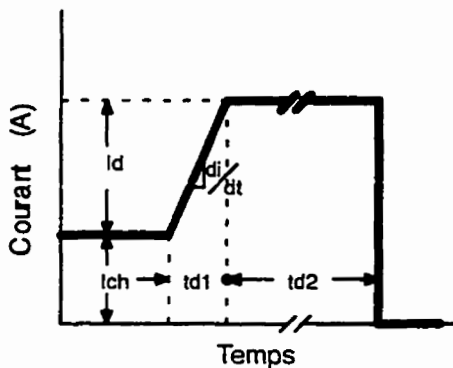
Figure 4.2: Conditions de détection de défaut
