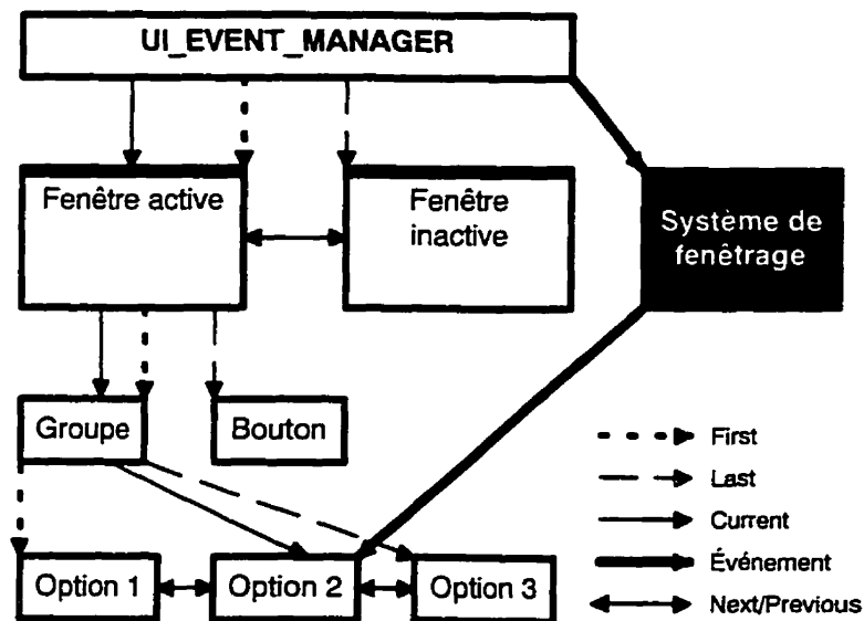
Figure 7.28: Traitement de l'exemple de l'architecture ascendante
