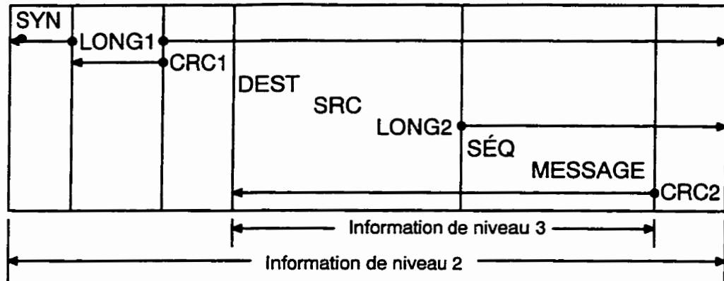
Figure 6.3: Niveau 1 du protocole de communications
