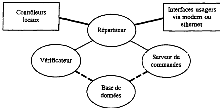
Figure 2.4: Diagramme d'interaction des logiciels du contrôleur central
