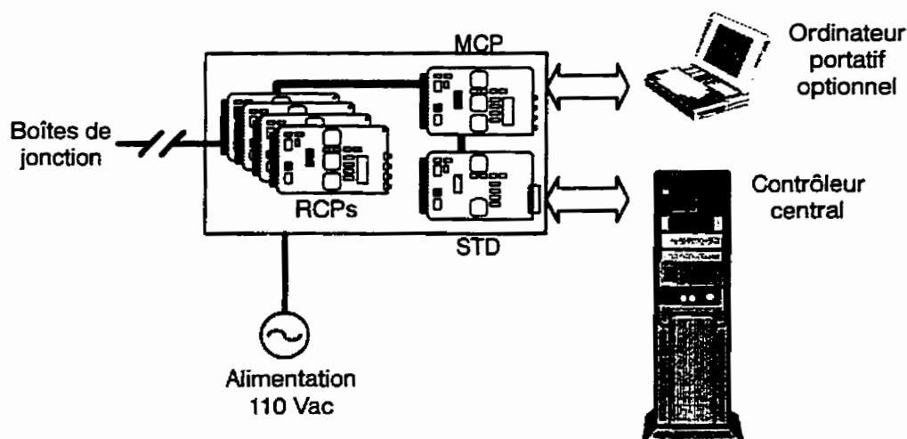
Figure 2.3: Diagramme fonctionnel d'un contrôleur local
