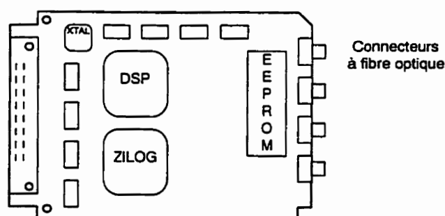
Figure 5.8: Carte RCP – disposition du processeur et de ses composantes
