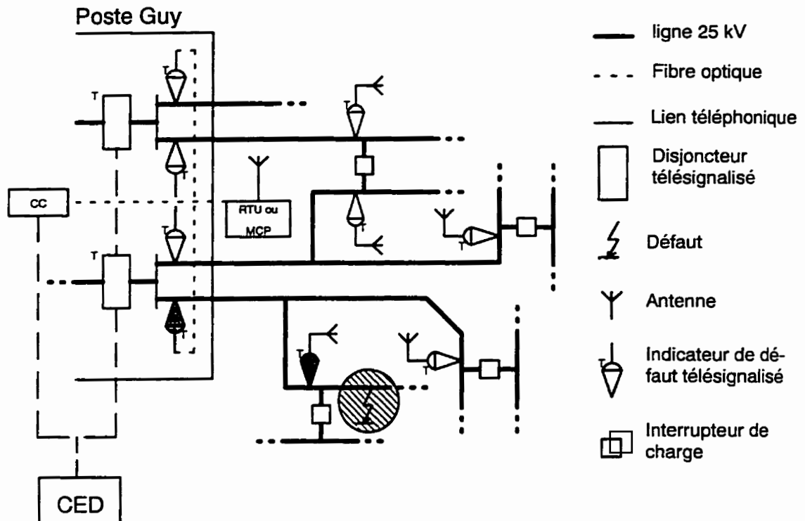
Figure 1.1: Exemple d'utilisation du système de télésignalisation en réseau
