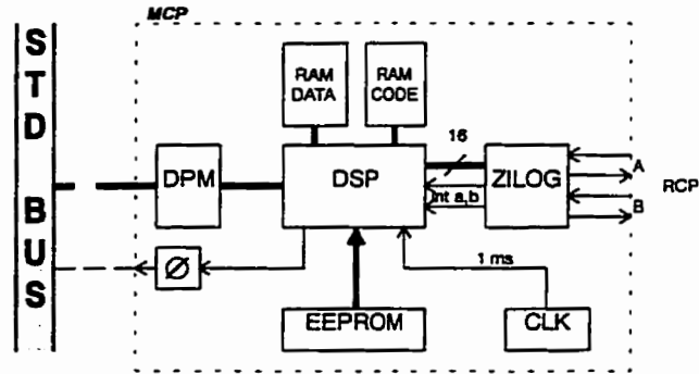
Figure 5.2: Architecture générale du MCP
