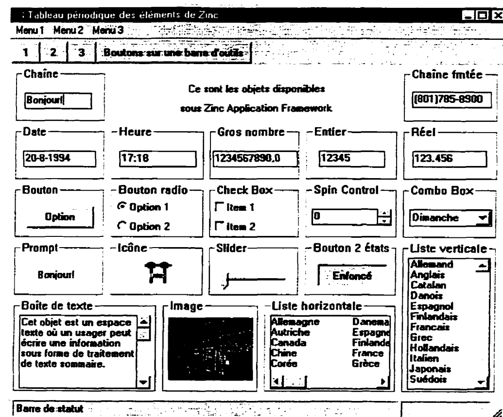
Figure 7.30: Objets dans la bibliothèque Zinc Application Framework
