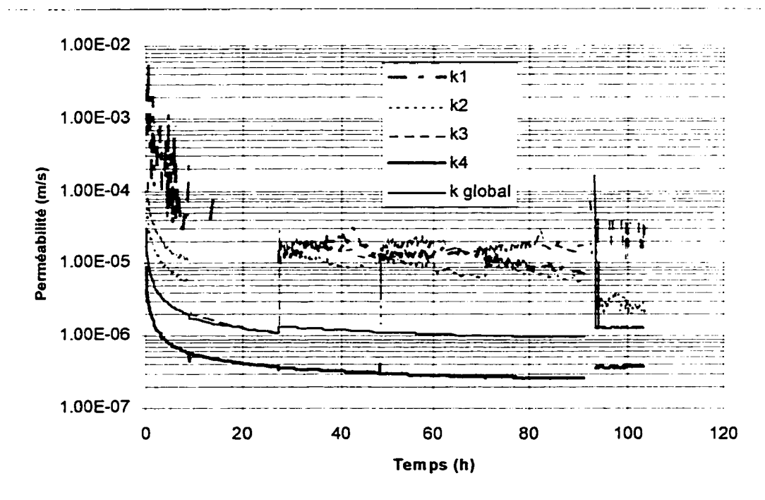
Figure 5.2 Perméabilités locales en fonction du temps pour l'essai 0
