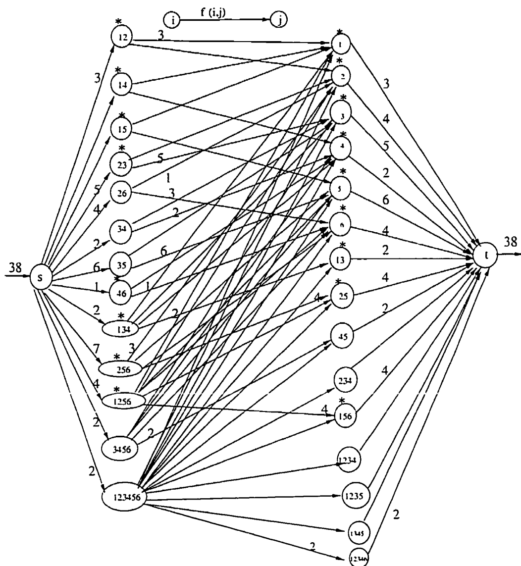
Figure 3.5 Les résultats du flot maximum avec le flot > 0 à côté de chaque arc.
