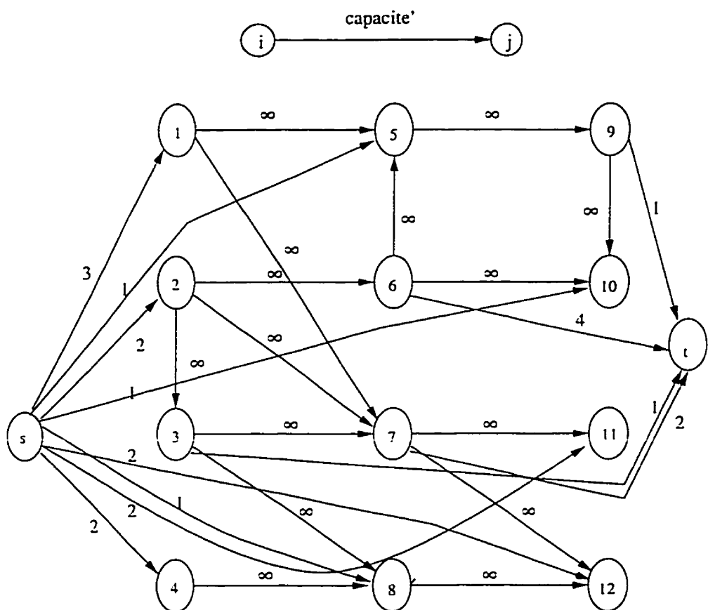
Figure 2.2 Réseau associé au graphe de la Figure 2.1.
