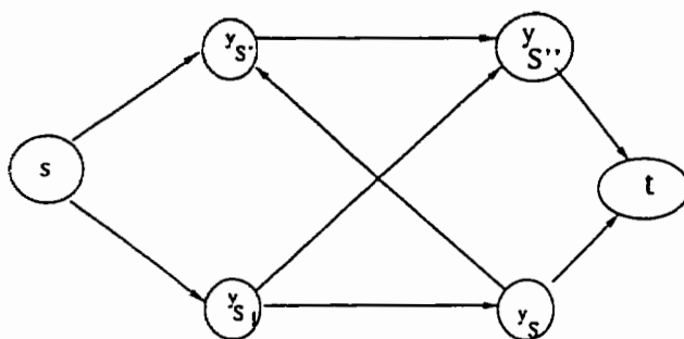
Figure 3.3 L'arc (y_s, y_{s'}) peut être éliminé.
