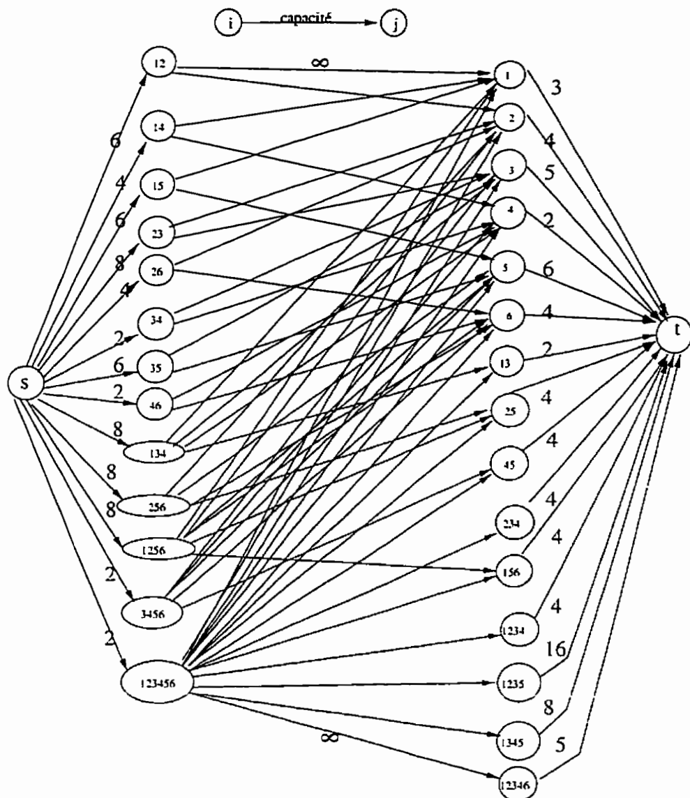
Figure 3.4 Le réseau associé au graphe construit à partir de f(X,Y) .
