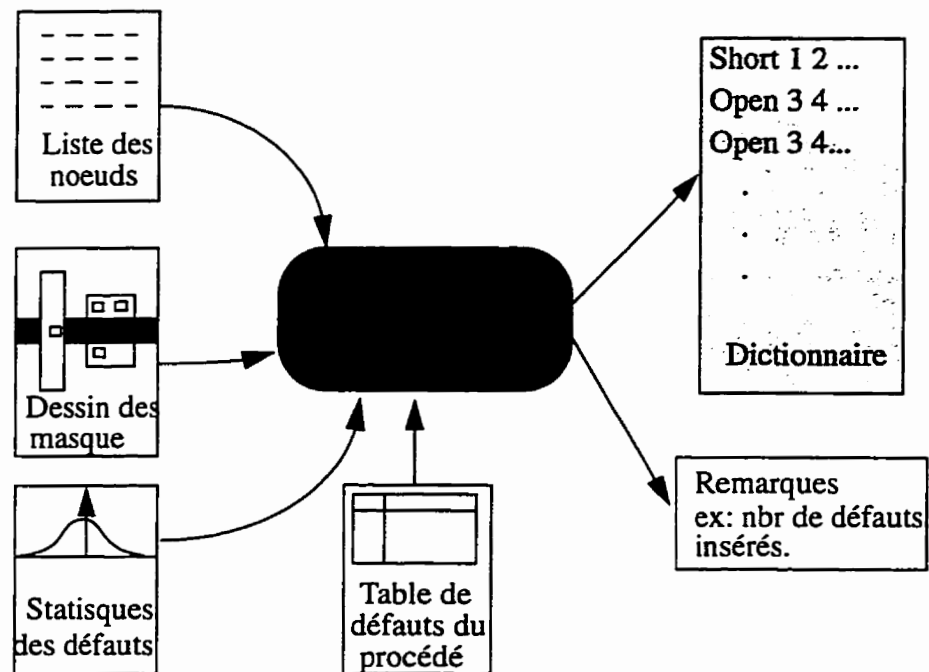
FIGURE 2.4 Entrées et sorties des générateur de dictionnaires de pannes
