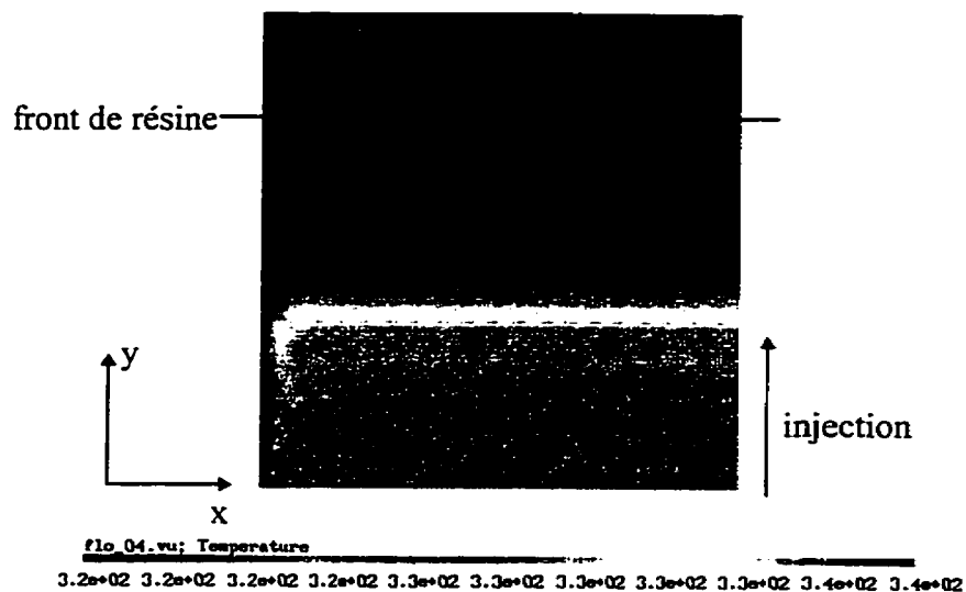
Figure 7.4 Température à 235 s. ( z=0,02 )
