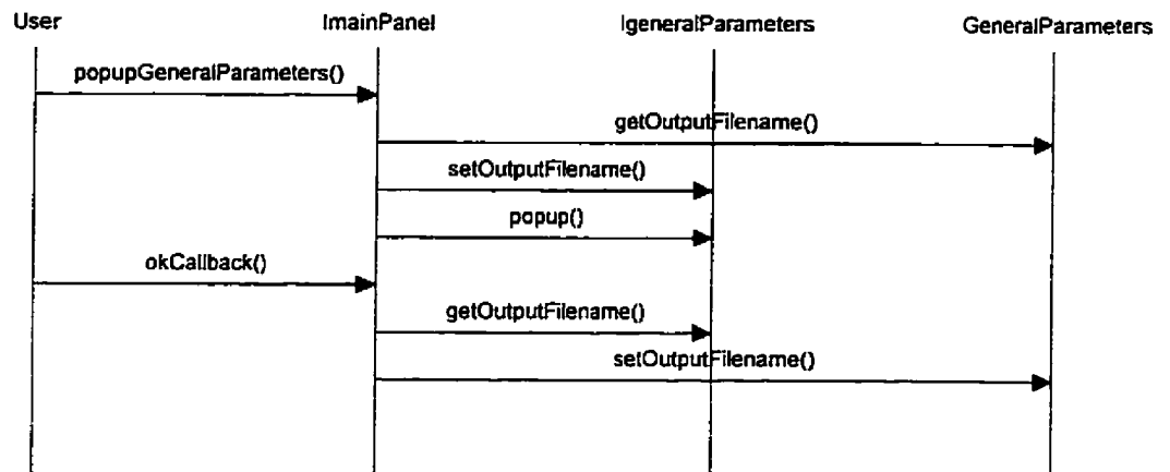
Figure 6.4 Modification proposée à l'échange de messages lors de l'ouverture et de l'enregistrement du contenu d'un panneau
