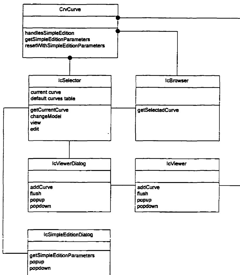
Figure 6.5 Classes impliquées dans le système d'association interactive d'une courbe à un paramètre de simulation
