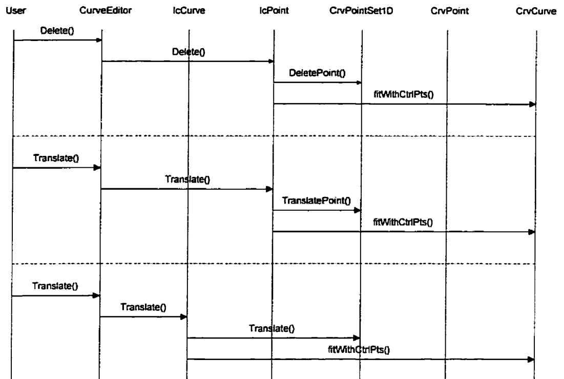
Figure 4.7 Diagramme d'événements pour la translation et la destruction d'un point de contrôle dans l'éditeur de courbes
