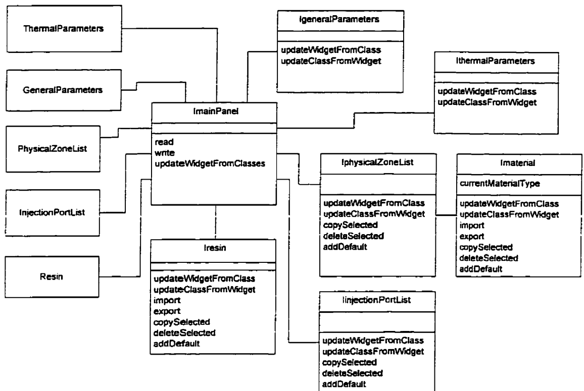
Figure 6.2 Modèle objet de Dataflot
