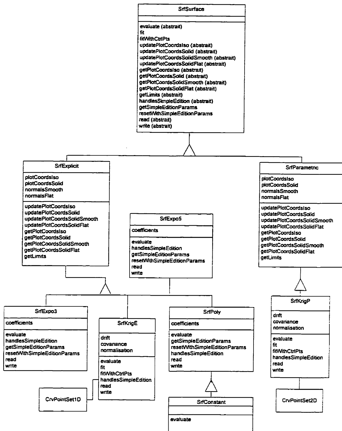
Figure 2.10 Modèle objet de la bibliothèque de surfaces
