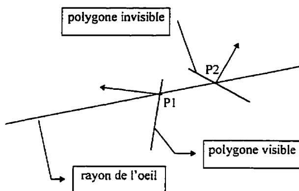
Figure 3.6 Élimination de primitives par l'algorithme de la normale
