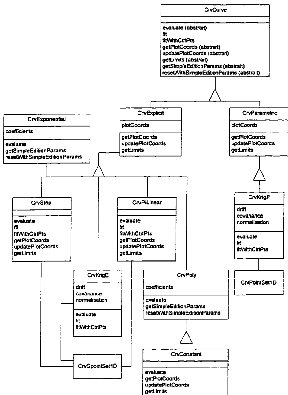
Figure 2.6 Modèle objet de la bibliothèque de courbes
