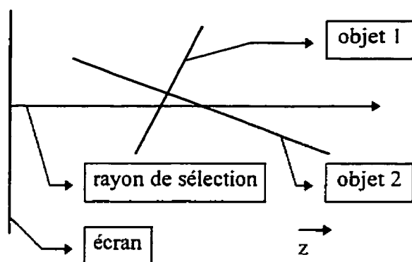
Figure 3.4 Sélection ponctuelle en 3D menant à la sélection d'un objet caché
