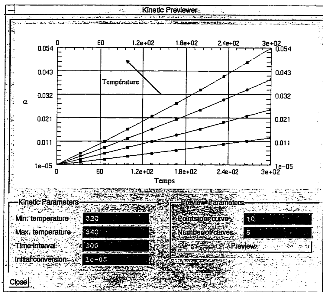
Figure 7.11 Cinétique chimique pendant la phase de remplissage
