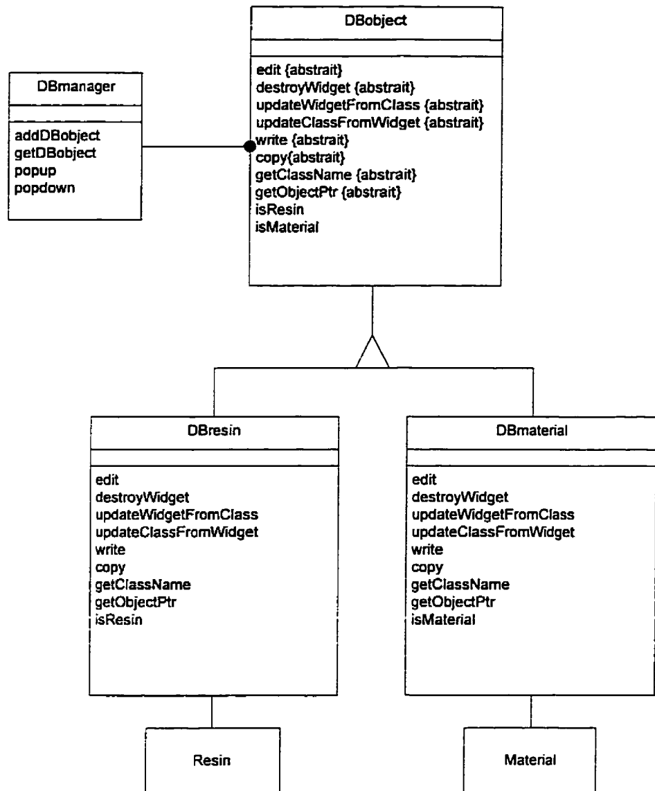
Figure 6.9 Architecture proposée pour la généralisation du gestionnaire de base de données
