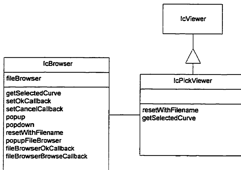
Figure 4.5 Sous-système de chargement d'une courbe contenue dans un fichier
