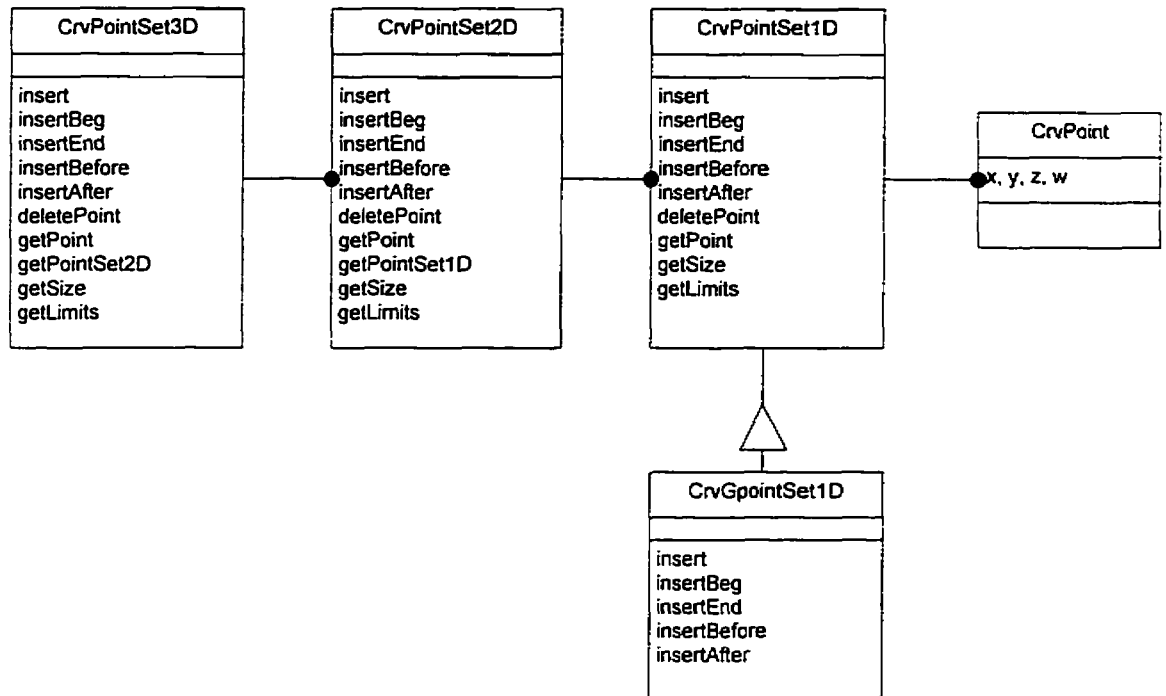
Figure 2.5 Diagramme d'objets décrivant les ensembles de points de contrôle
