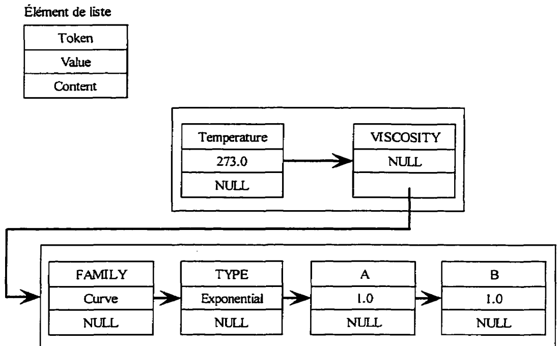
Figure 2.4 Arbre de jetons en mémoire
