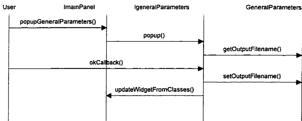
Figure 6.3 Échange de messages lors de l'ouverture d'un panneau et de l'enregistrement des modifications
