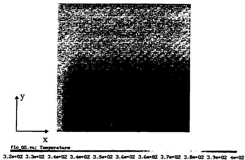
Figure 7.6 Température à t=1020 s. ( z=0,02 )
