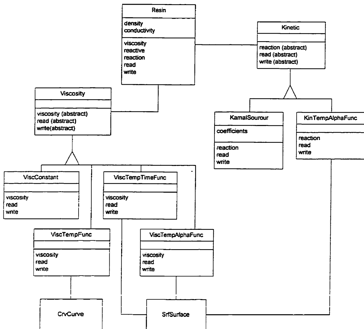
Figure 6.1 Classes impliquées dans la définition d'une résine
