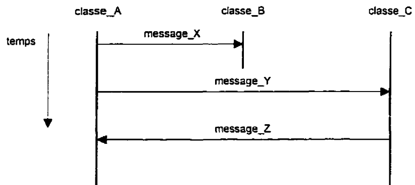
Figure 2.3 Diagramme d'événements
