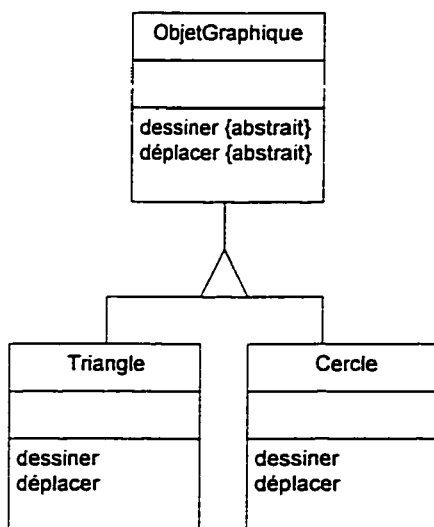
Figure 2.1 Diagramme de classes vs diagramme d'instances
