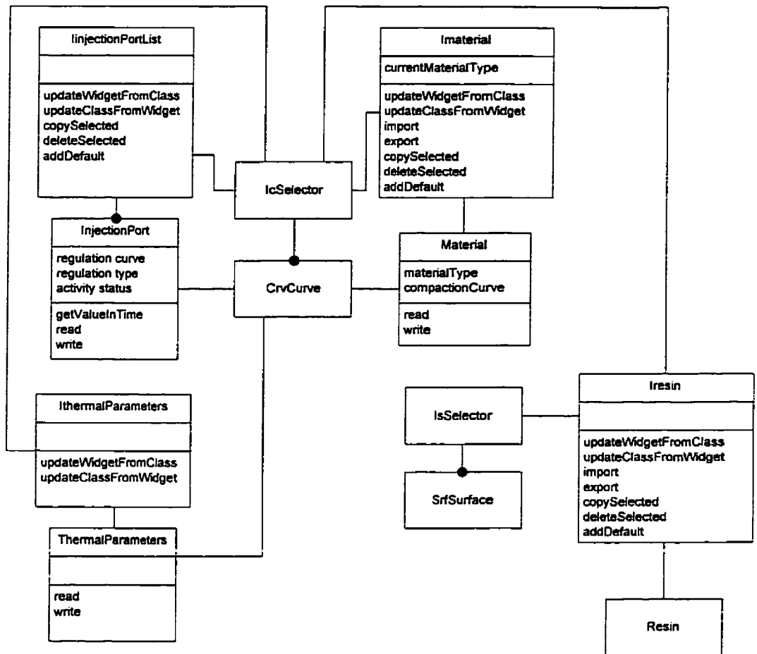
Figure 6.8 Vue d'ensemble de l'utilisation présente des courbes et des surfaces par Dataflot et Flot
