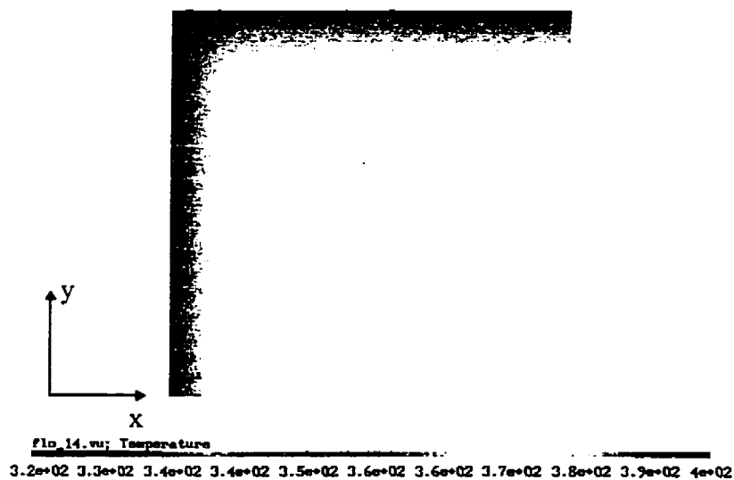
Figure 7.7 Température à t=2820 s. ( z=0,02 )
