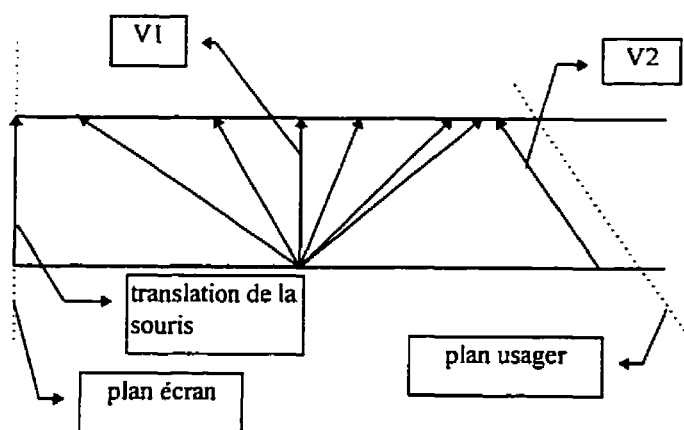
Figure 4.8 Interprétation d'une translation de la souris sur l'écran
