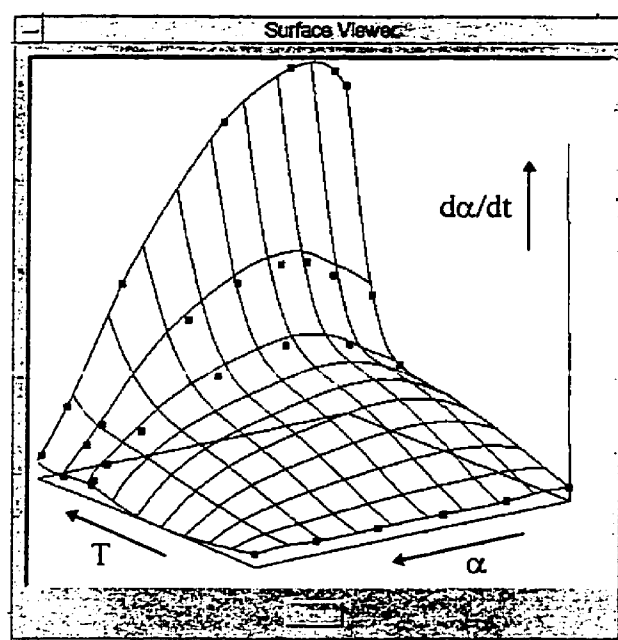
Figure 7.10 Cinétique krigée
