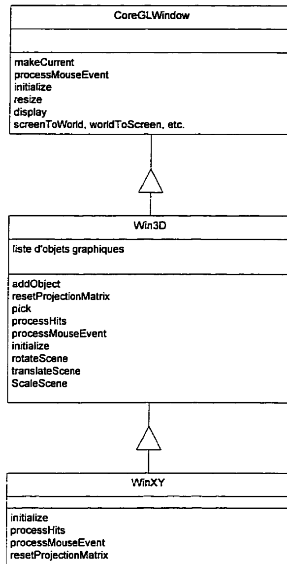
Figure 3.1 Hiérarchie des classes de visualisation
