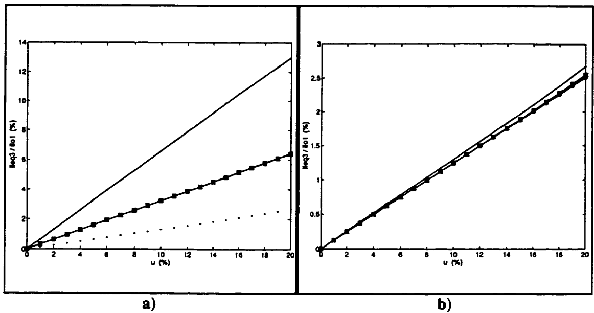
Figure 1.23 - Harmonique de courant équivalent de rang trois en fonction du taux de déséquilibre u avec \beta = 75^\circ et \alpha = 40^\circ ; convertisseurs: --- 6; --o-- 12; --*-- 18; ---+--- 24 pulsations; a) commande individuelle; b) commande équidistante
