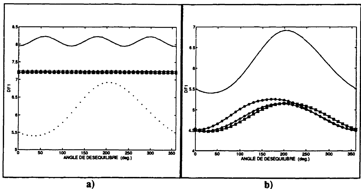
Figure 1.20 - DF_1 en fonction de l'angle de déséquilibre \beta avec u = 10\% et \alpha = 40^\circ ; convertisseurs: --- 6; --o-- 12; --*-- 18; --- 24 pulsations; a) commande individuelle; b) commande équidistante
