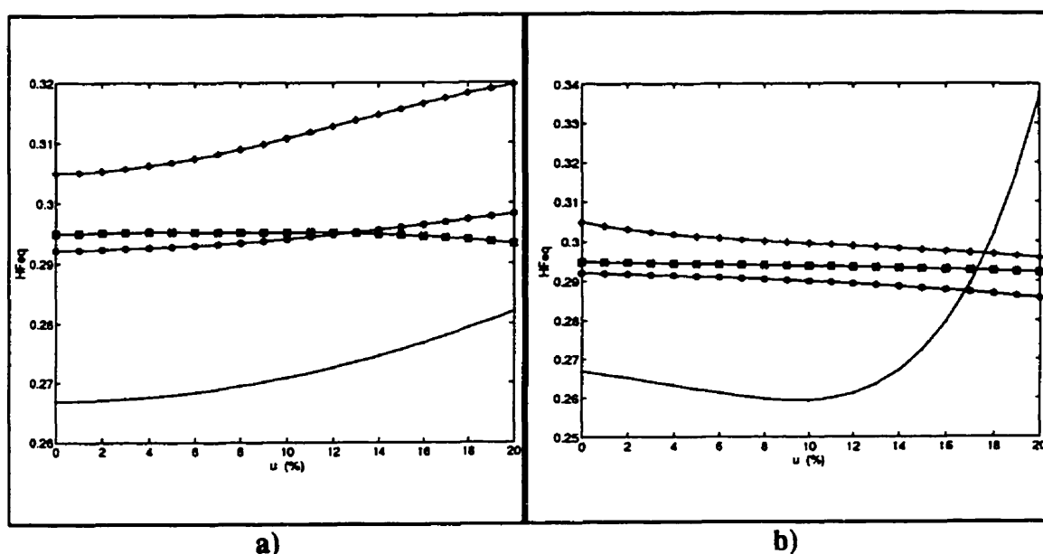
Figure 1.13 - Taux d'harmoniques équivalent en fonction du taux de déséquilibre u avec \beta = 75^\circ ; \alpha : --- 10°; --o-- 40°; --*-- 60°; --+-- 80°; a) commande individuelle; b) commande équidistante
