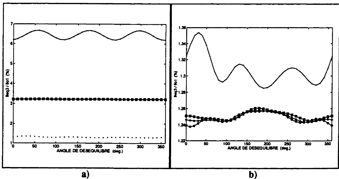
Figure 1.24 - Harmonique de courant équivalent de rang trois en fonction de l'angle de déséquilibre \beta avec u=10 et \alpha=40^\circ ; convertisseurs: --- 6; --o-- 12; --*-- 18; ---+--- 24 pulsations; a) commande individuelle; b) commande équidistante
