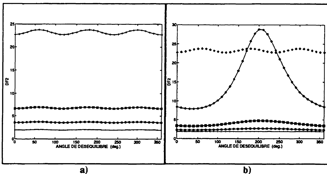
Figure 1.9 - DF_2 en fonction de l'angle de déséquilibre \beta avec u=10\% ; \alpha : --- 10^\circ ; -o- 40^\circ ; -*-- 60^\circ ; ---+-- 80^\circ ; a) commande individuelle; b) commande équidistante
