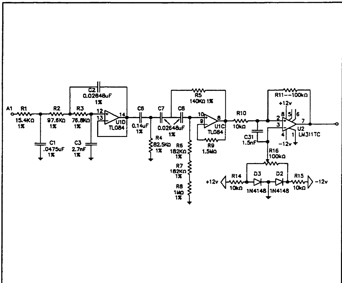
Figure V.2 - Détecteur de passage par zéro
