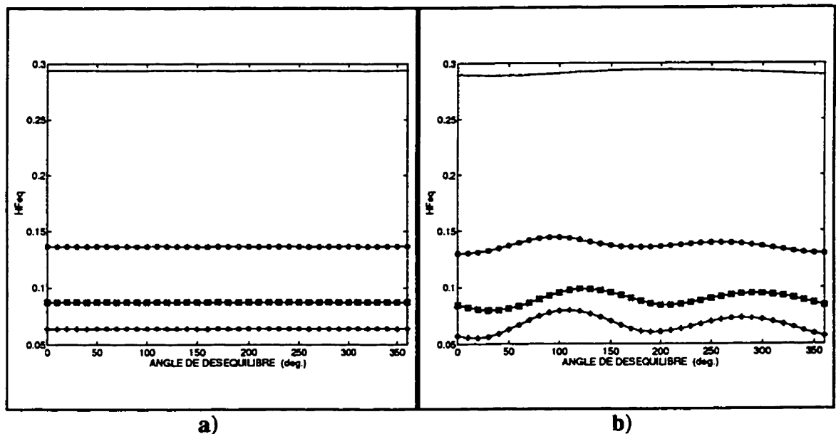
Figure 1.26 - Taux d'harmoniques de courants alternatifs en fonction de l'angle de déséquilibre \beta avec u=10\% et \alpha=40^\circ ; convertisseurs: --- 6; -.- 12; -.*- 18; --+-- 24; a) commande individuelle; b) commande équidistante
