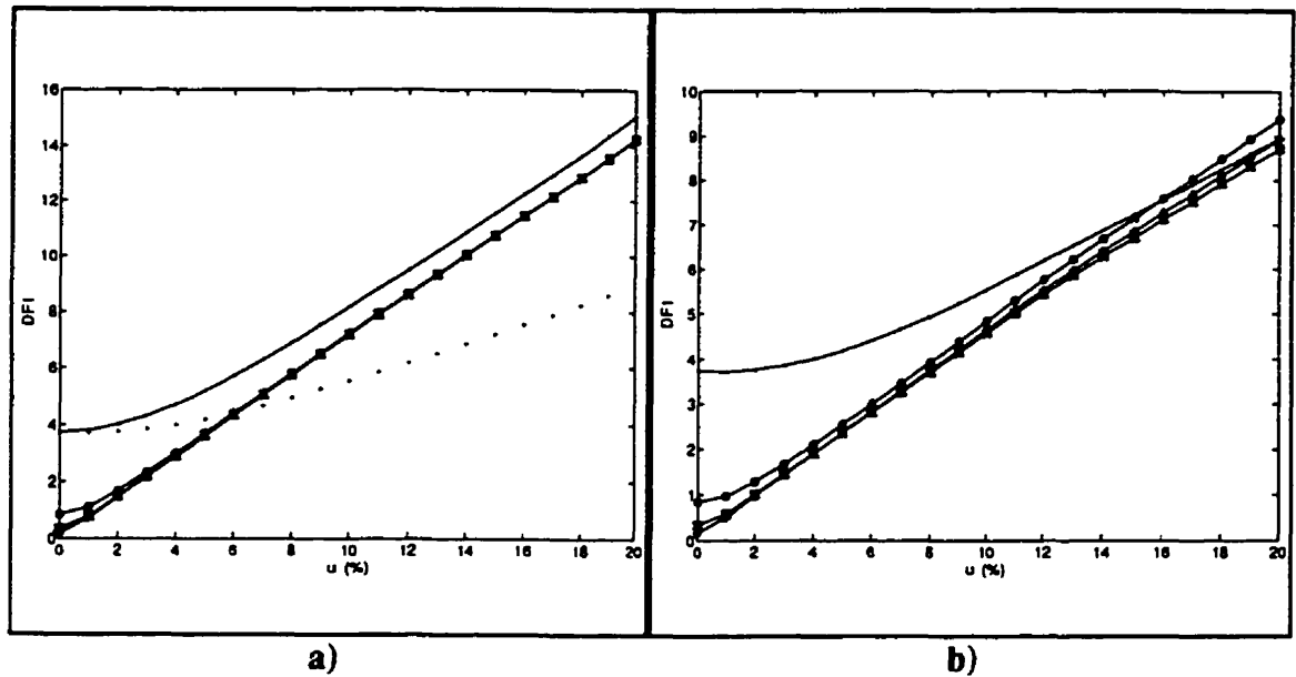
Figure 1.19 - DF_1 en fonction du taux de déséquilibre u avec \beta = 75^\circ et \alpha = 40^\circ ; convertisseurs: --- 6; --o-- 12; --*-- 18; --- 24 pulsations; a) commande individuelle; b) commande équidistante
