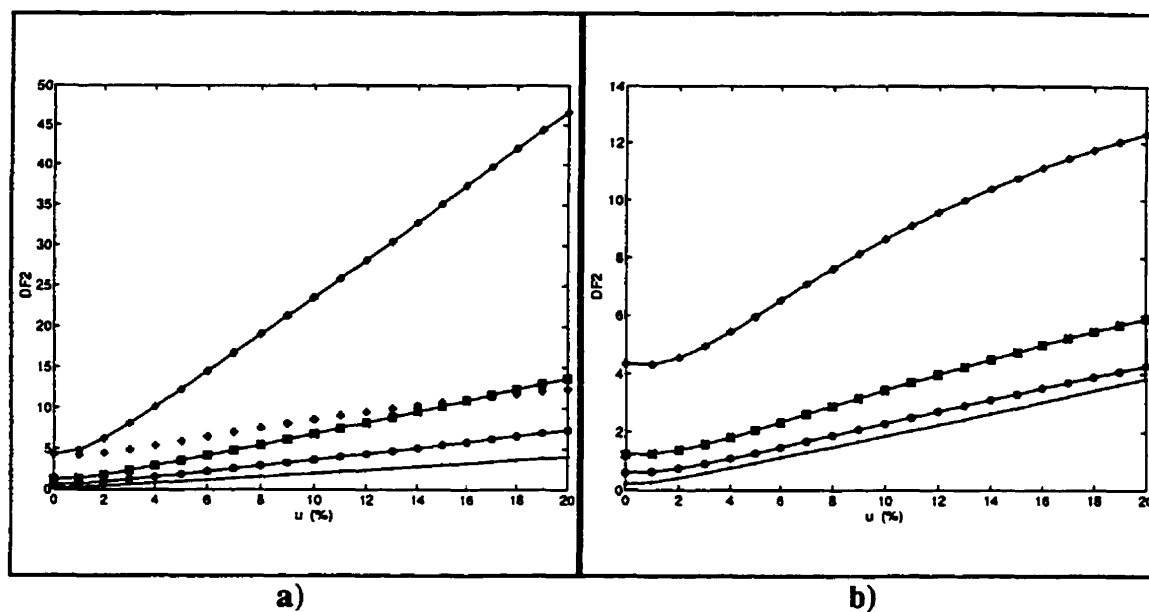
Figure 1.8 - DF_2 en fonction du taux de déséquilibre u avec \beta = 75^\circ ; \alpha : --- 10^\circ ; -o- 40^\circ ; -*-- 60^\circ ; ---+-- 80^\circ ; a) commande individuelle; b) commande équidistante
