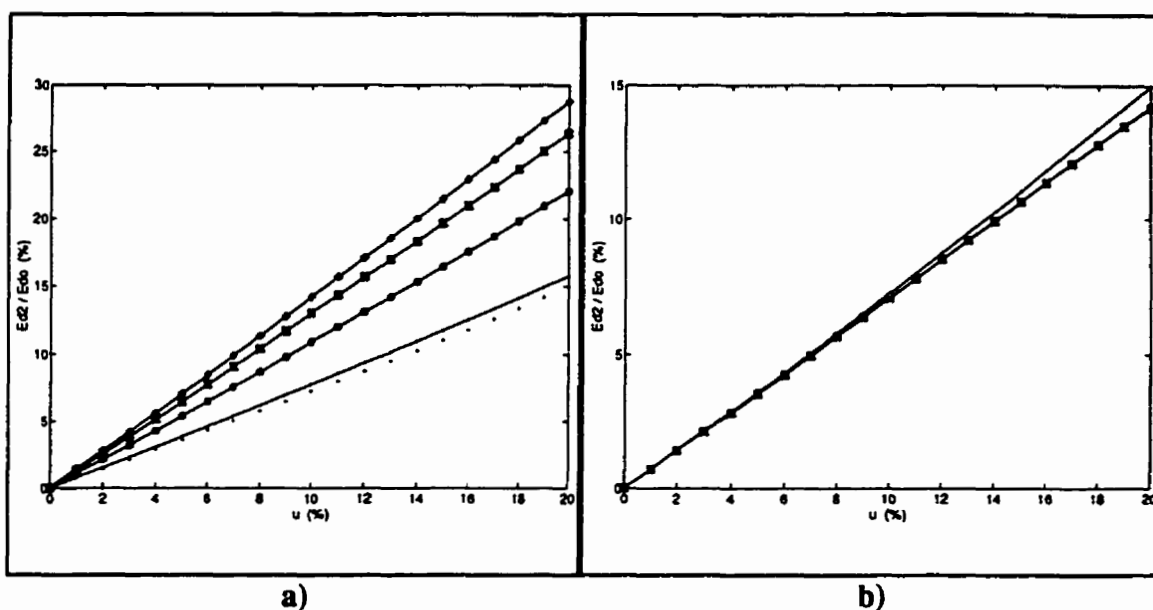
Figure 1.4 - Valeur efficace du deuxième harmonique en fonction du taux de déséquilibre u avec \beta=75^\circ ; \alpha : --.. 10°; --o-- 40°; --*-- 60°; --+-- 80°; a) commande individuelle; b) commande équidistante
