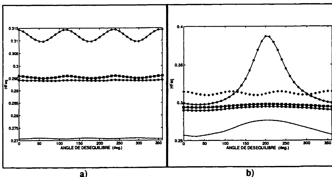
Figure 1.14 - Taux d'harmoniques équivalent en fonction de l'angle de déséquilibre \beta avec u=10\% ; \alpha : --- 10°; --o-- 40°; --*-- 60°; --+-- 80°; a) commande individuelle; b) commande équidistante
