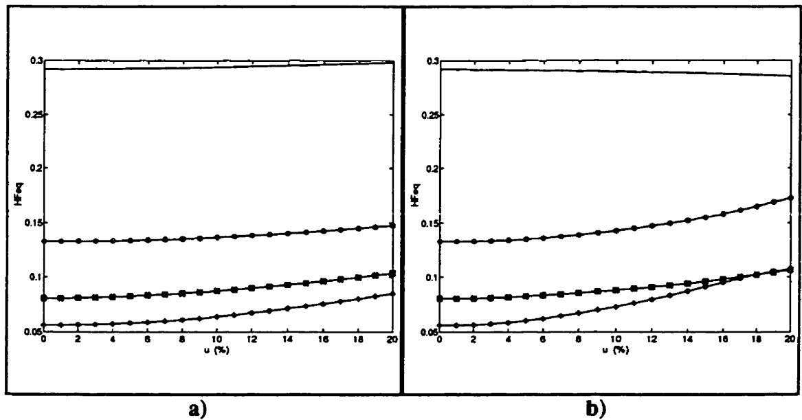
Figure 1.25 - Taux d'harmoniques de courants alternatifs en fonction du taux de déséquilibre u avec \beta = 75^\circ et \alpha = 40^\circ ; convertisseurs: -- 6; --o-- 12; --*-- 18; --+-- 24; a) commande individuelle; b) commande équidistante
