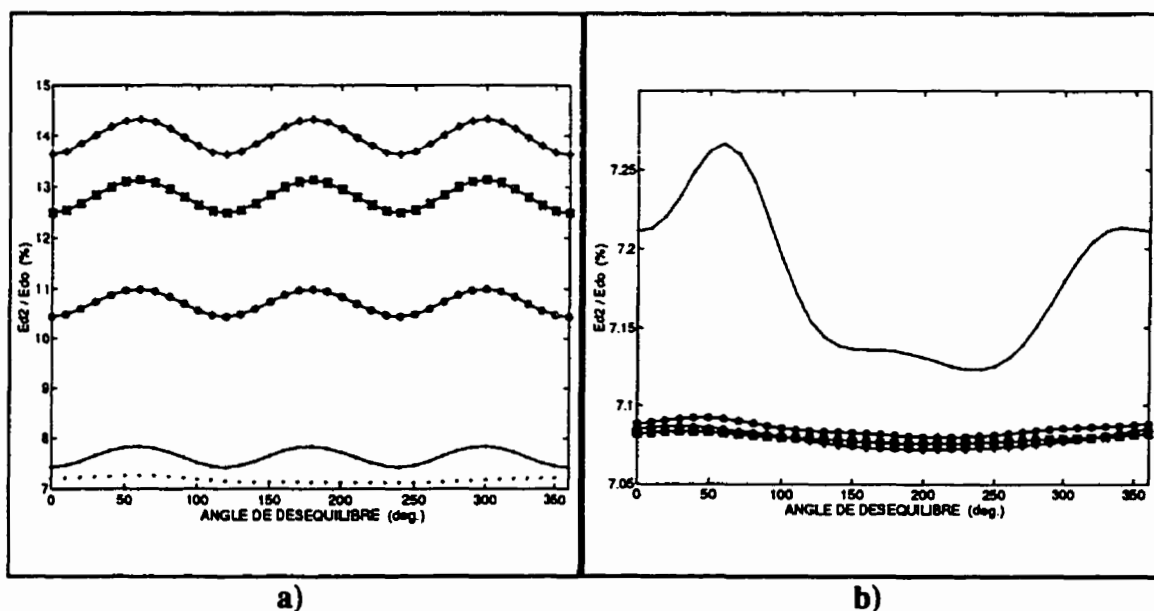
Figure 1.5 - Valeur efficace du deuxième harmonique en fonction de l'angle de déséquilibre \beta avec u=10\% ; \alpha : --.. 10°; --o-- 40°; --*-- 60°; --+-- 80°; a) commande individuelle; b) commande équidistante
