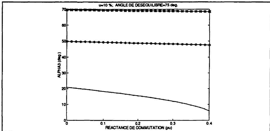
Figure 2.2-c - Variations de \alpha_3 avec X_c (---.--- \alpha=30^\circ ; ---o--- \alpha=60^\circ ; ---*--- \alpha=80^\circ )
