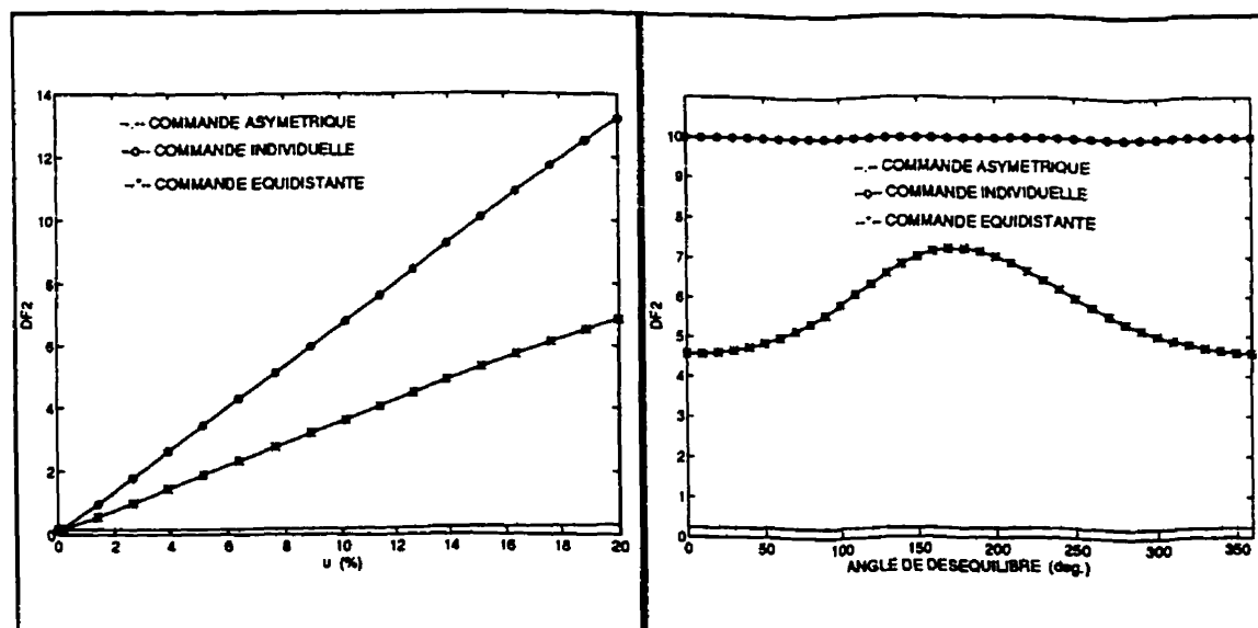
Figure 2.7 - Convertisseur dodécaphasé: taux de distorsion DF_2 en fonction du taux de déséquilibre u ( \beta=75^\circ ; \alpha=60^\circ )
