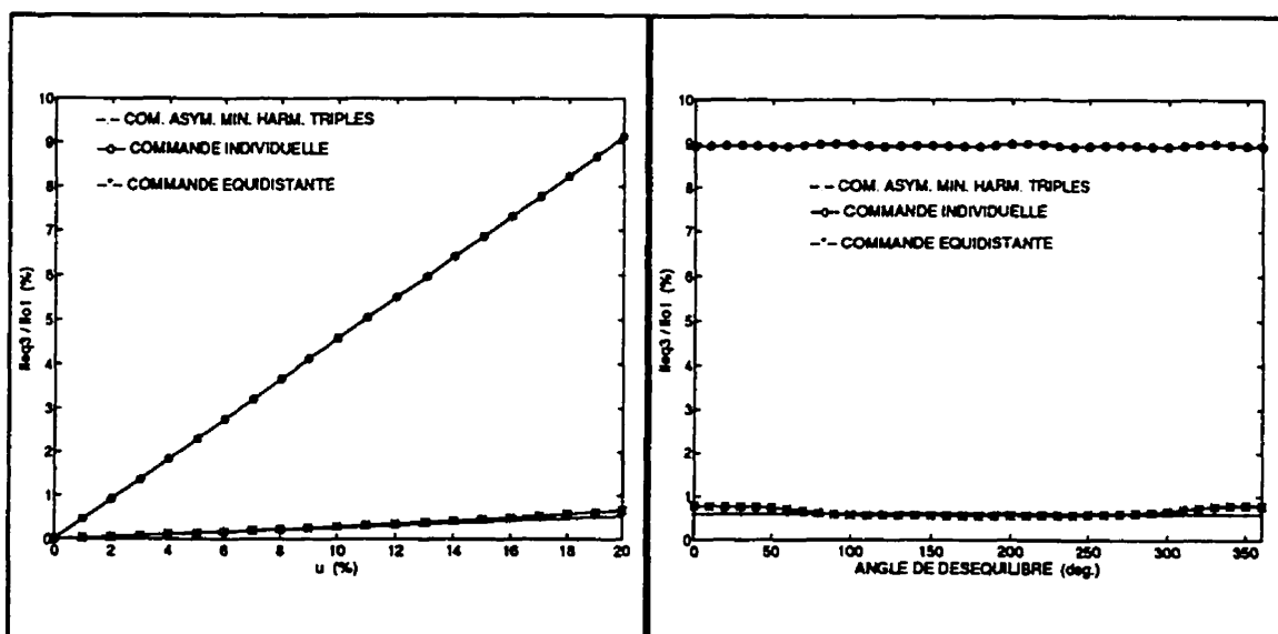
Figure 5.7 - Convertisseur dodécaphasé: 3 ème harmonique équivalent de courant ca en fonction du taux de déséquilibre u ( \beta=60^\circ ; \alpha=65^\circ )
