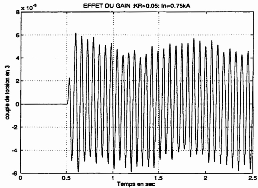
Fig. 4.11: Couple de torsion ( 10^{-6} Nm) en S_3 vs Temps (s)
