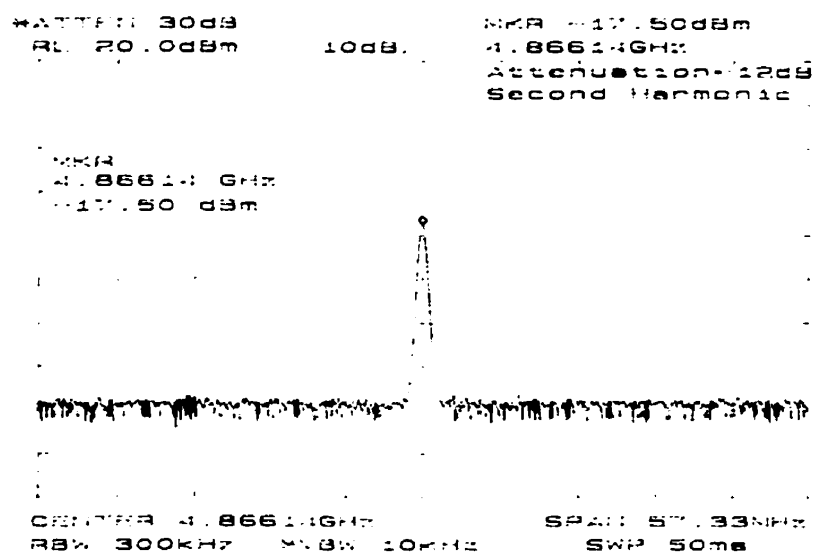
Figure 5.17: Deuxième harmonique.
