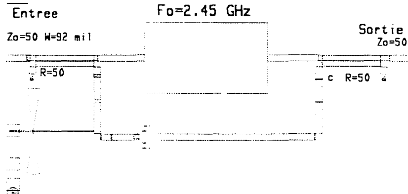
Figure 4.10: Résonateur actif utilisant l'amplificateur monolithique ERA5
