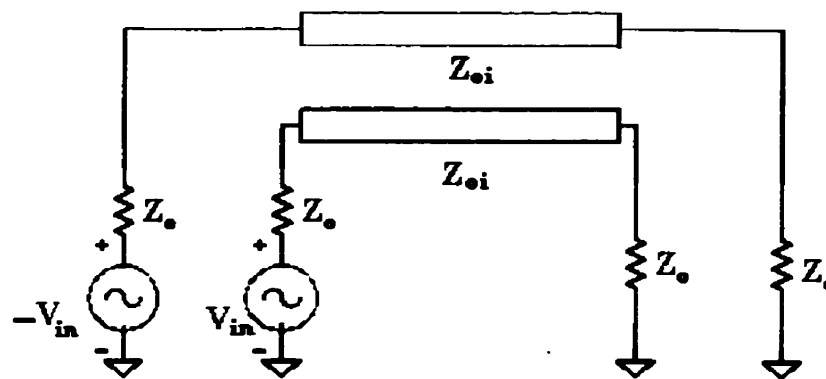
Figure 3.3: Circuit Équivalent pour mode impair
