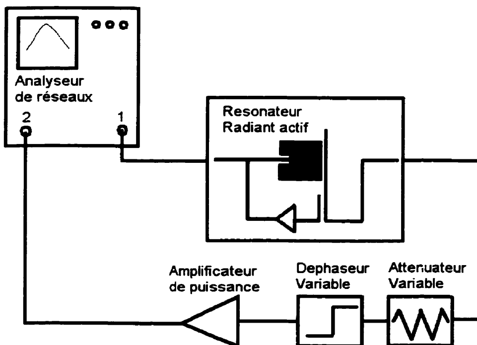
Figure 5.6: Montage utilisé pour le mesure du circuit d'oscillateur à boucle ouverte.
