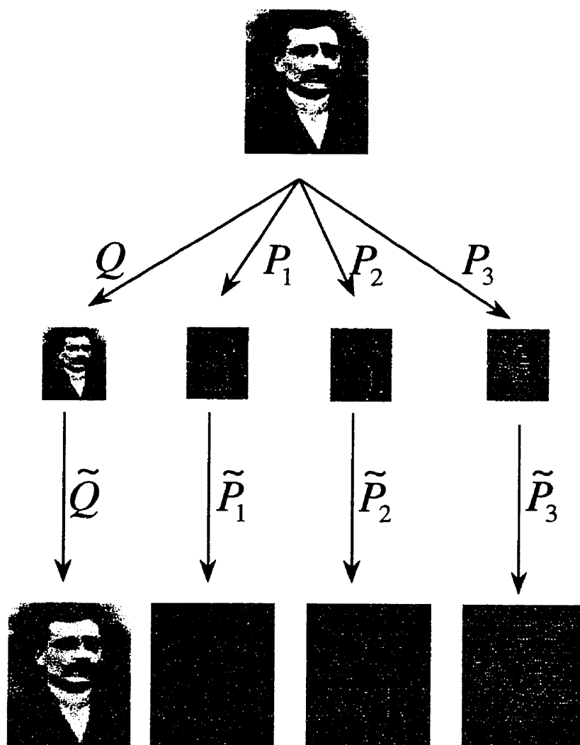
Figure 4.3: Illustration d'une décomposition par ondelettes
