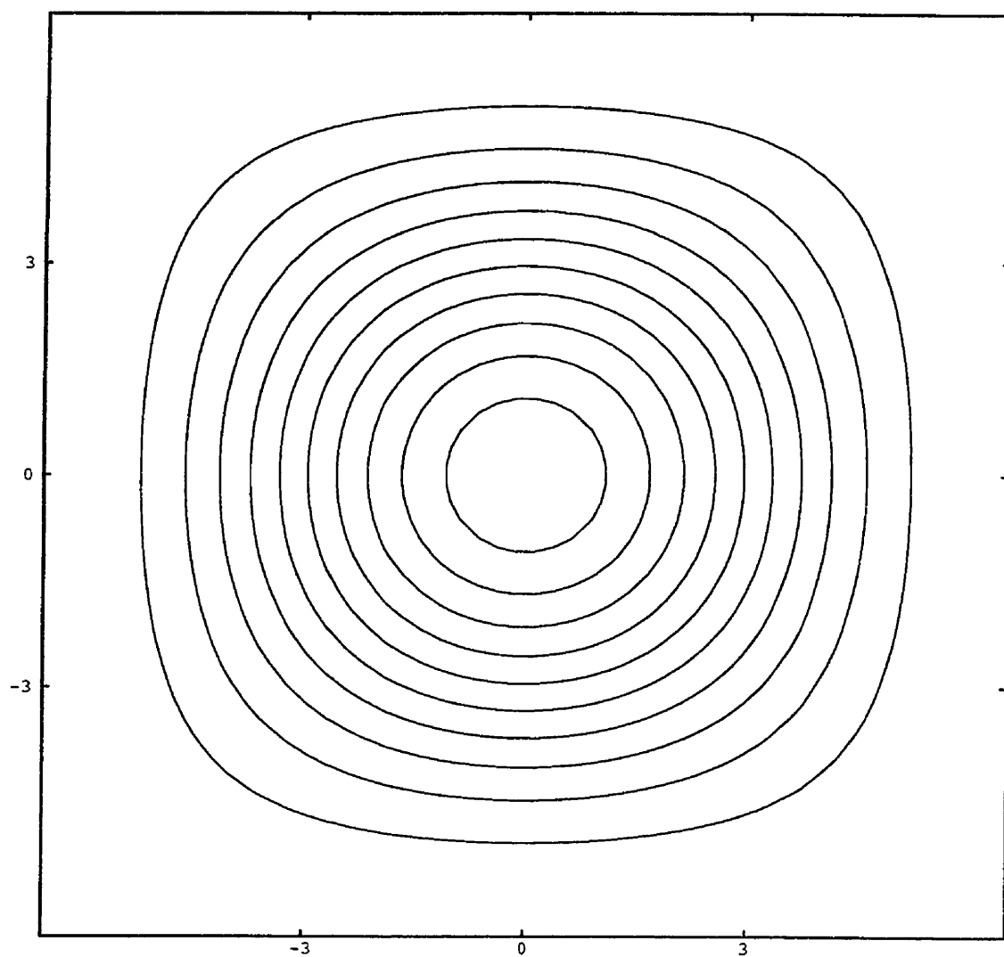
Figure 4.1: Contours du polynôme caractéristique de la fonction d'échelle primaire (\phi)
