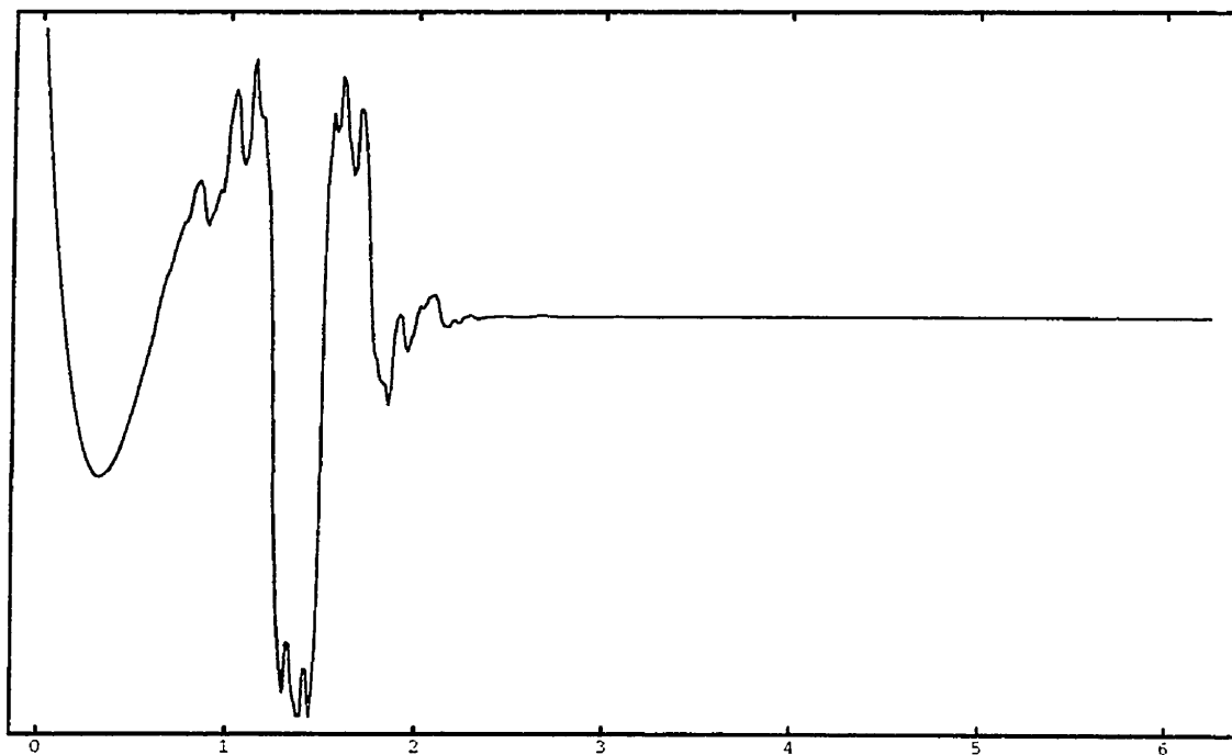
Figure 3.1: Ondelette duale _{3.5}\hat{\psi}_{j,0} pour j quelconque
