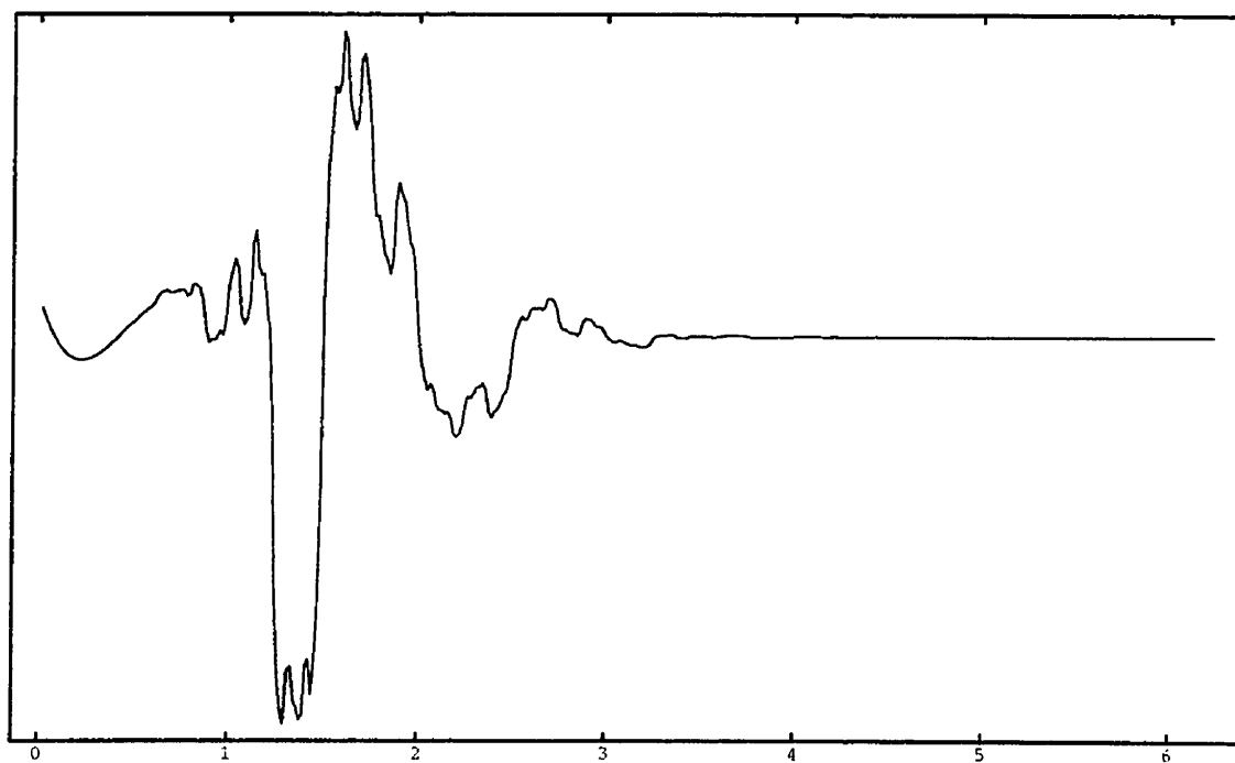
Figure 3.2: Ondelette duale _{3.5}\hat{\psi}_{j,1} pour j quelconque
