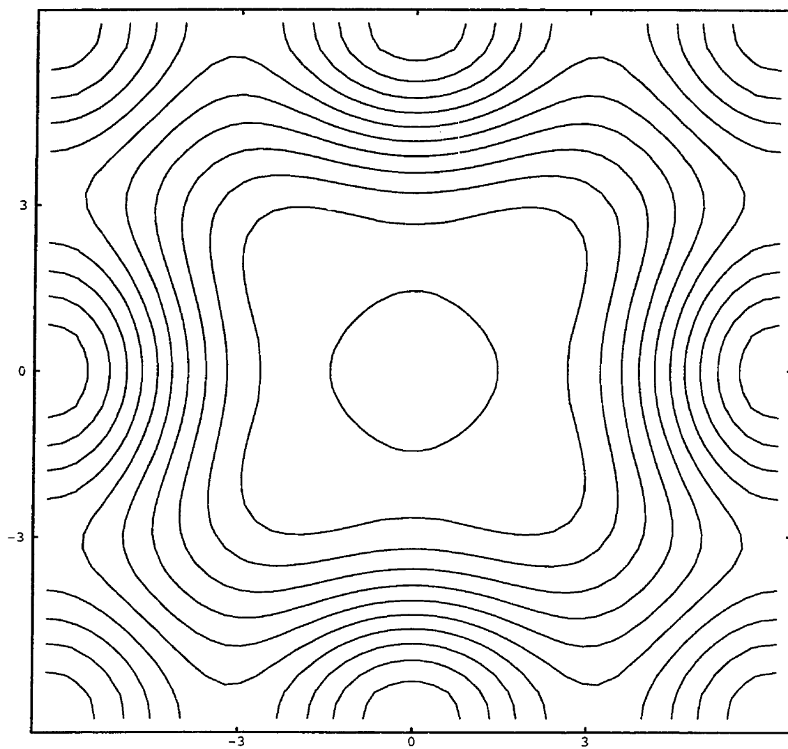
Figure 4.2: Contours du polynôme caractéristique de la fonction d'échelle duale ( \tilde{\phi} )
