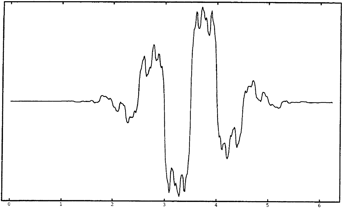
Figure 3.4: Ondelette duale {}_{3,5}\tilde{\psi}_{j,3} pour j quelconque (correspond à l'ondelette de Cohen Daubechies Feauveau)
