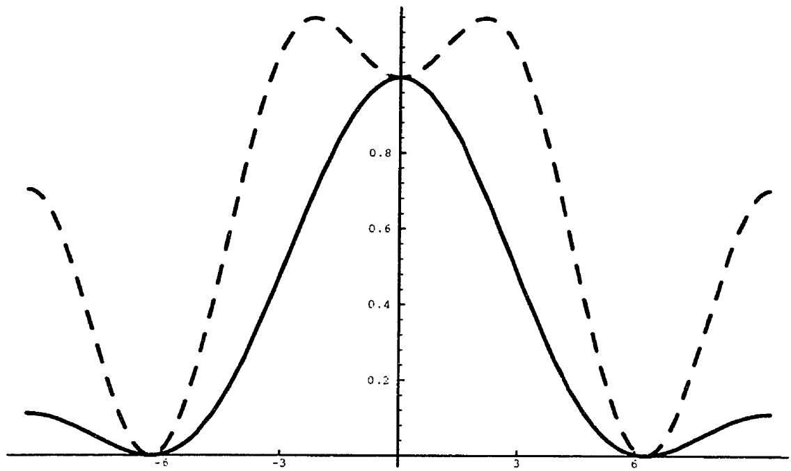
Figure 2.5: Polynômes caractéristiques des fonctions d'échelles pour N = \tilde{N} = 2 (le polynôme dual est en pointillé et l'ordonnée est en \xi )
