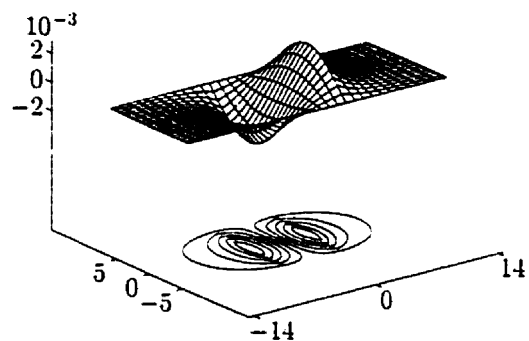
(d) H_y
