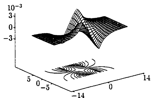
(f) H_z
