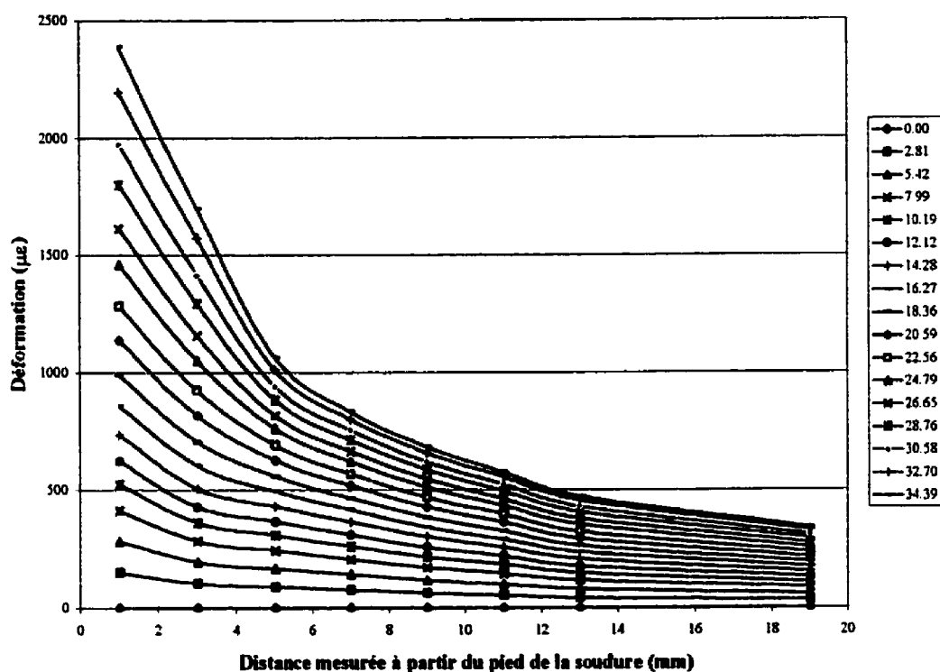
Figure 5-9 : Déformations mesurées selon la charge appliquée
