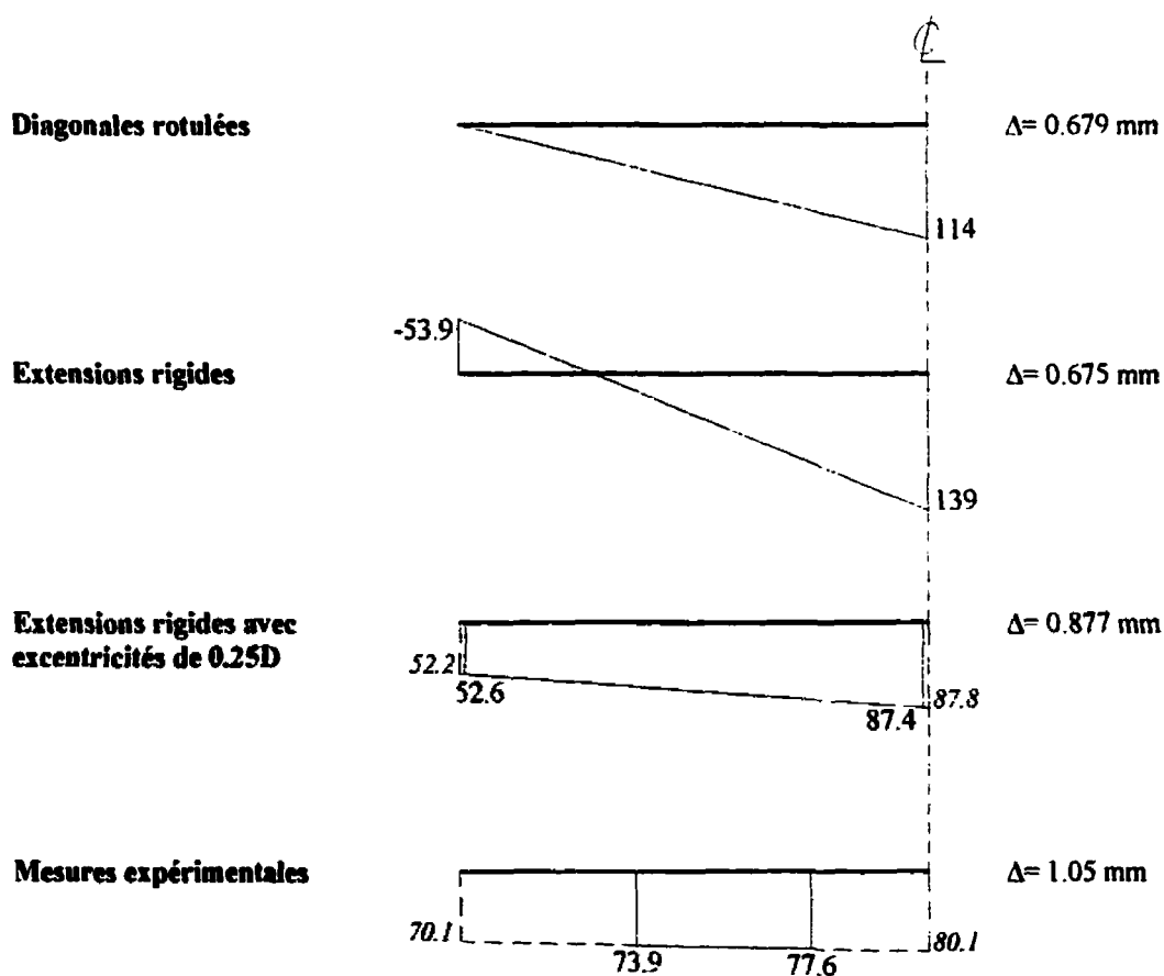
Figure 5-7 : Distribution des moments dans le longeron supérieur ( P=10.19 \text{ kN} )
