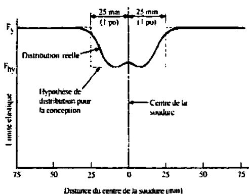
Figure 2-1 : Distribution des propriétés mécaniques de l'aluminium dans la ZAT
