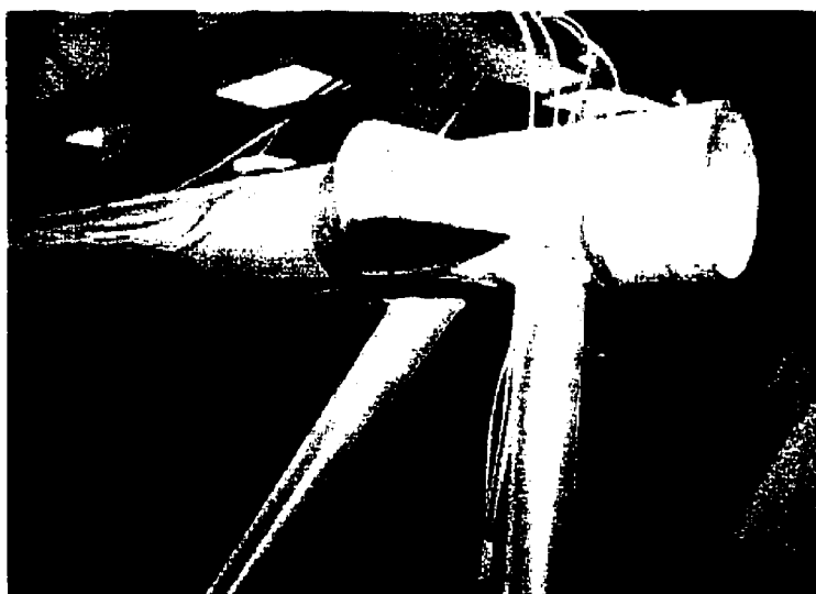
Figure 5-8 : Rupture de la diagonale lors de l'essai statique
