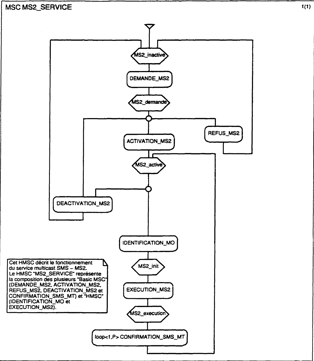
Figure B.2 : Le diagramme HMSC MS2_SERVICE
