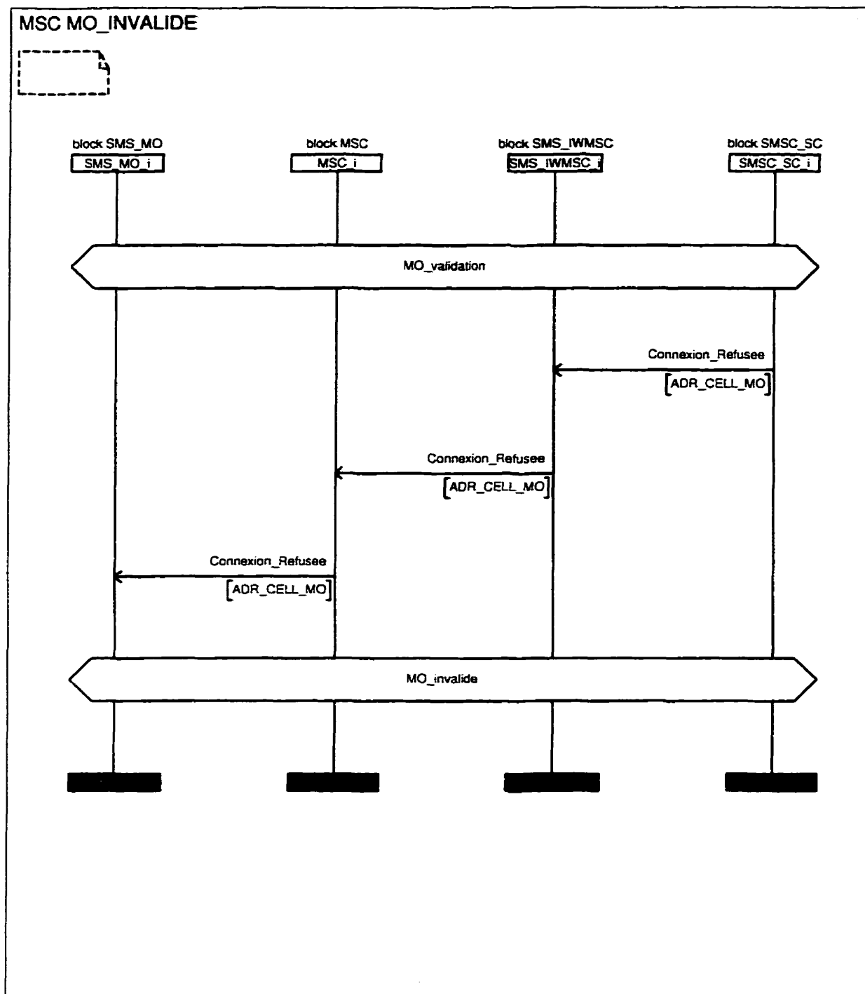
Figure B.10 : Le diagramme MSC MO_INVALIDE
