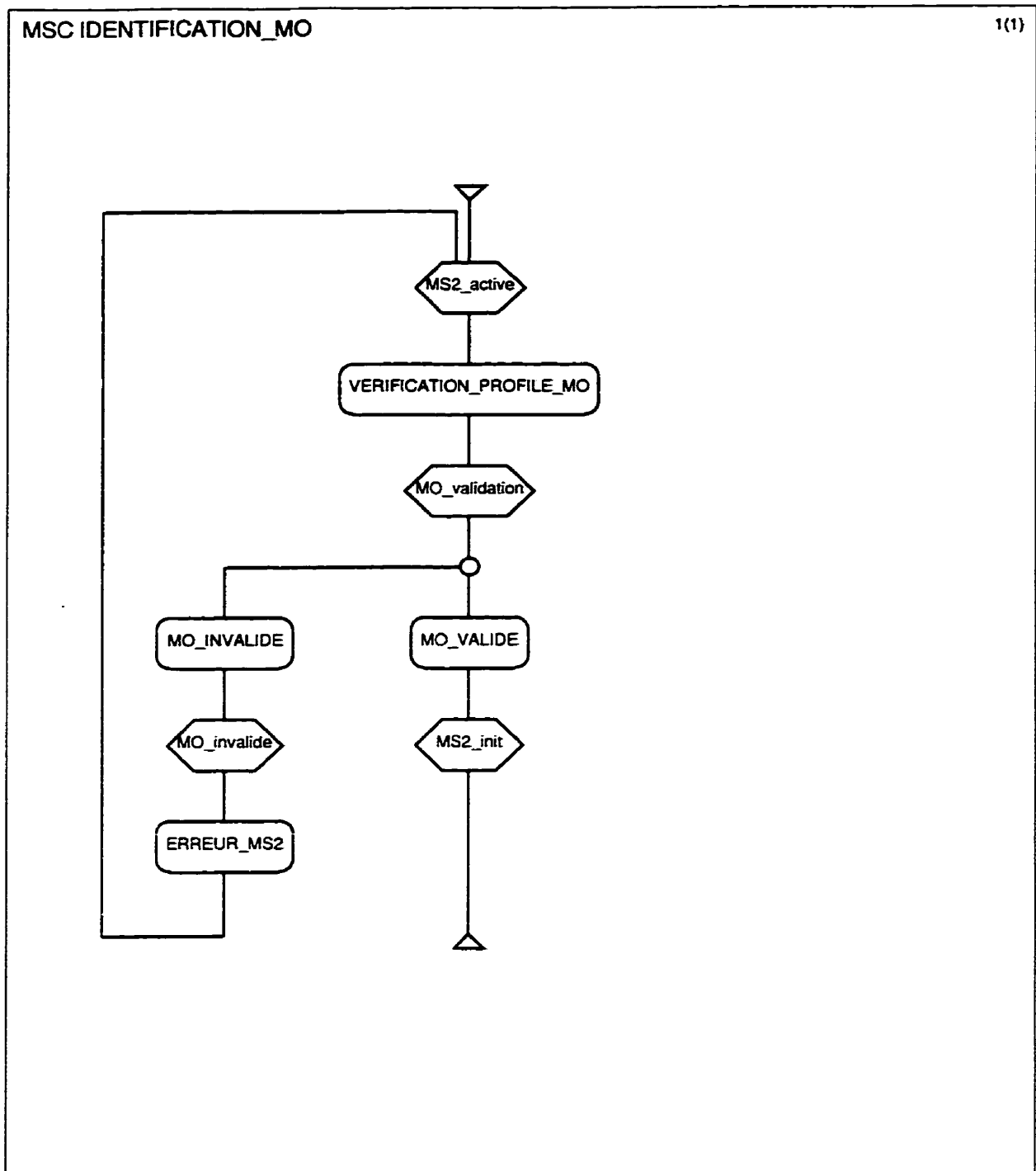
Figure B.7 : Le diagramme HMSC IDENTIFICATION_MO
