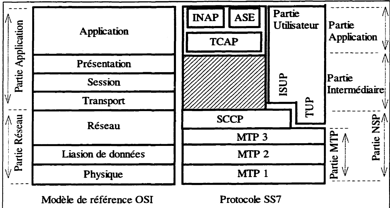
Figure 2.2 : La comparaison entre le modèle OSI et l'architecture du protocole SS7
