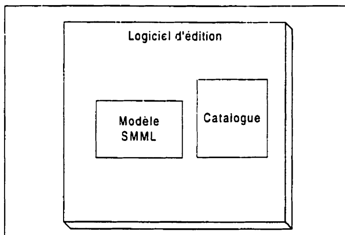
Figure 4.7 – Structure d'un logiciel implantant le modèle SMML avec le catalogue
