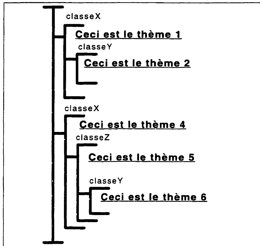
Figure 5.2 – Présentation de la structure d'un document SMML
