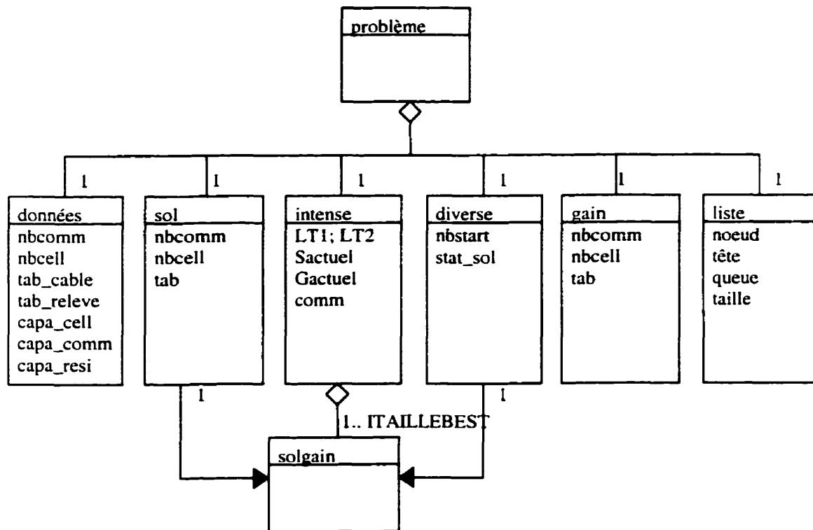
Figure 4.7 Diagramme des principales classes
