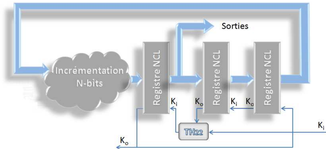
Figure A4-9. Circuit d'incrément N-bits en logique NCL
