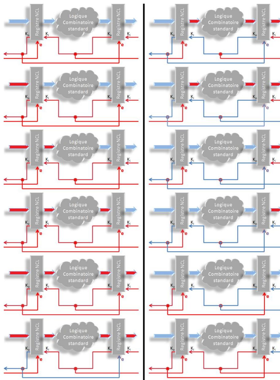
Figure 4-18. Exemple de protocole SHF-NCL cas n°2
