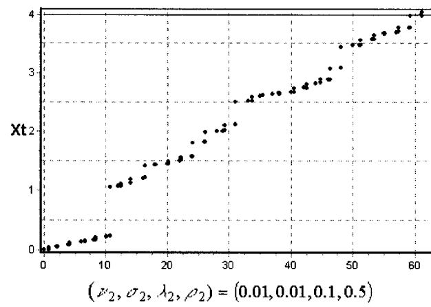
Figure 4.9: Graphique de la dégradation pour le client 2.
