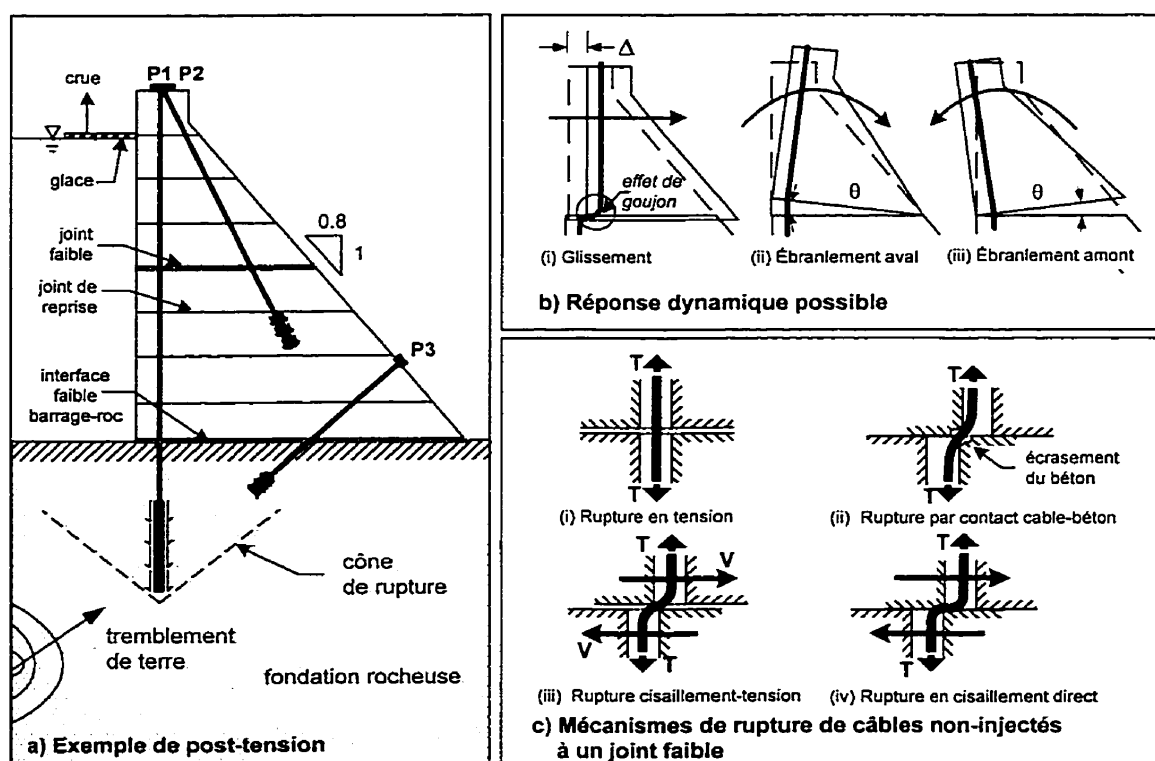
Figure I.1 Réponse sismique d'un barrage-poids post-tensionné.
