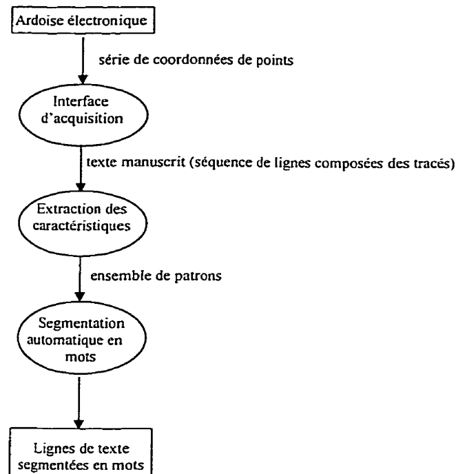
Figure 1.8. Diagramme des différents blocs du mode de segmentation automatique en mots.
