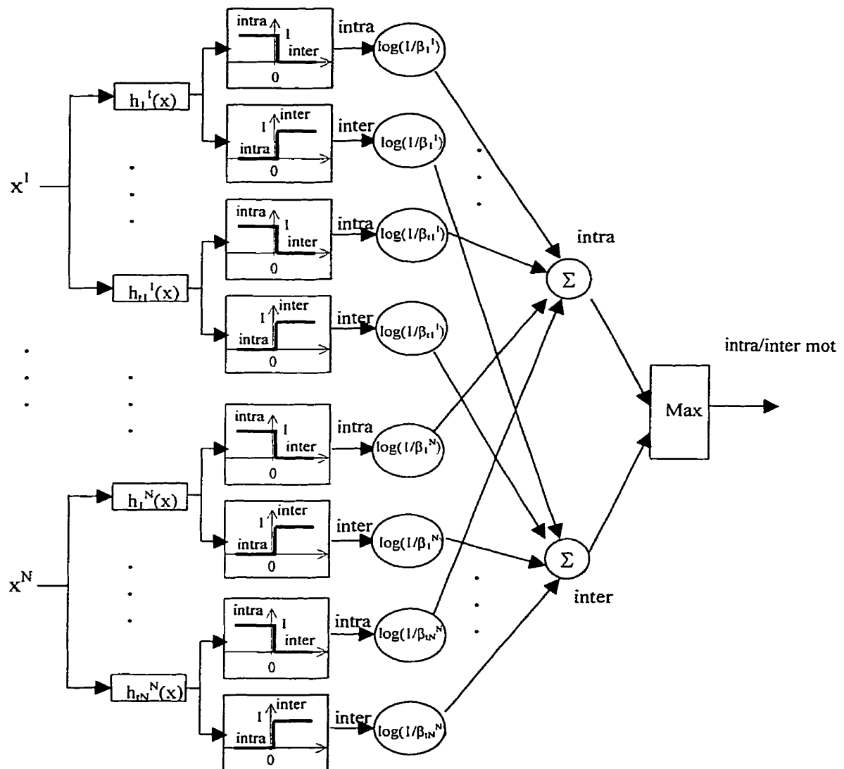
Figure 5.3. Structure générique des classificateurs basés sur la version initiale d'AdaBoost.
