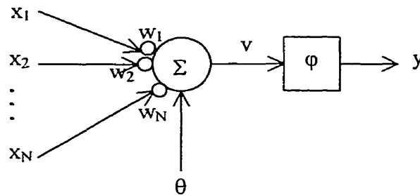
Figure 4.1. Modèle d'un neurone artificiel.
