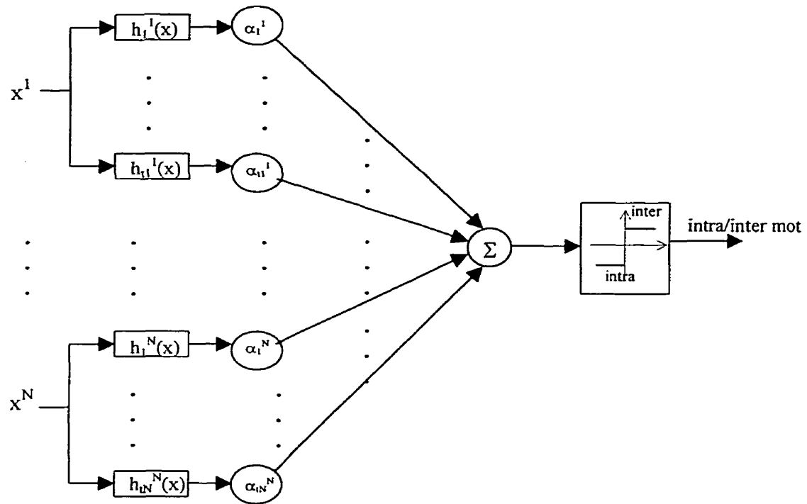
Figure 5.8. Structure générique des classificateurs AdaBoost.Z implantés.
