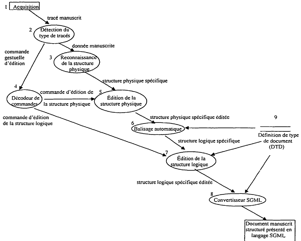
Figure 1.1. Diagramme de flux de données du système complet de traitement de documents manuscrits structurés, présenté dans (Moin, 1997).
