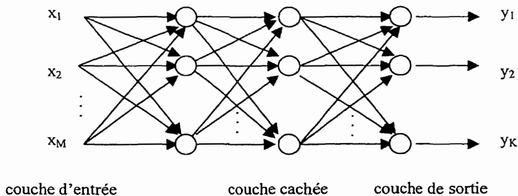
Figure 4.3. Structure d'un Perceptron multicouche
