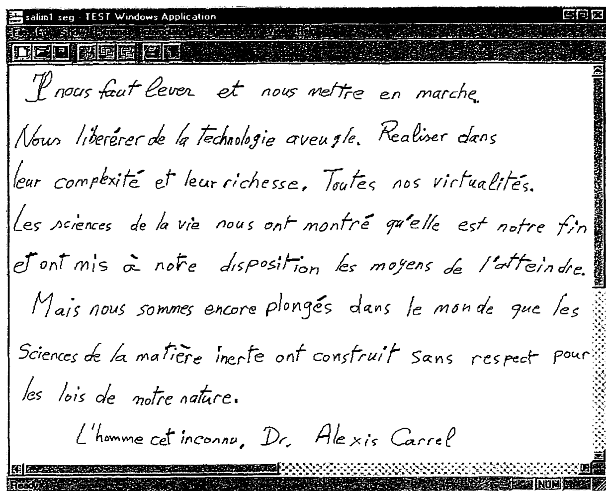
Figure 3.21. Résultat de l'application de l'algorithme de reconnaissance des Accent_Point_TBar sur un texte manuscrit. Les Accent_Point_TBars sont montrés plus épais que les autres tracés.
