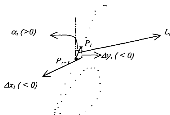
Figure 3.11. Un segment descendant du tracé 'b' et ses paramètres.
