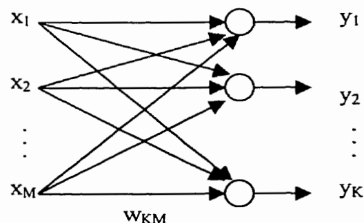
Figure 4.2. Structure d'un Perceptron à une couche.
