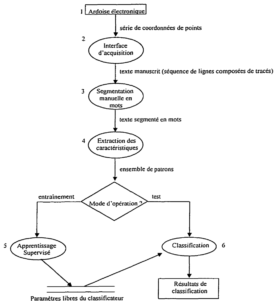
Figure 1.7. Schéma général du système de segmentation de textes manuscrits en mots, modes d'opération d'entraînement et de test.
