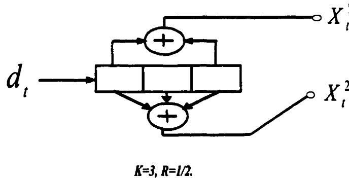
Figure 2.2: Codeur Convolutionnel non récursif et non systématique de matrice génératrice G(D) = [1 + D^2 \quad 1 + D + D^2]
