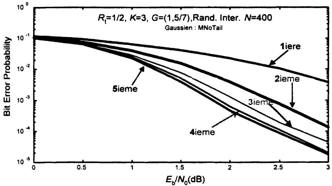
Figure 4.8: BER, K = 3 , R_t = 1/2 , N = 400 , Entrel. Aléatoire, Canal AWGN, Terminaison : MNoTail.
