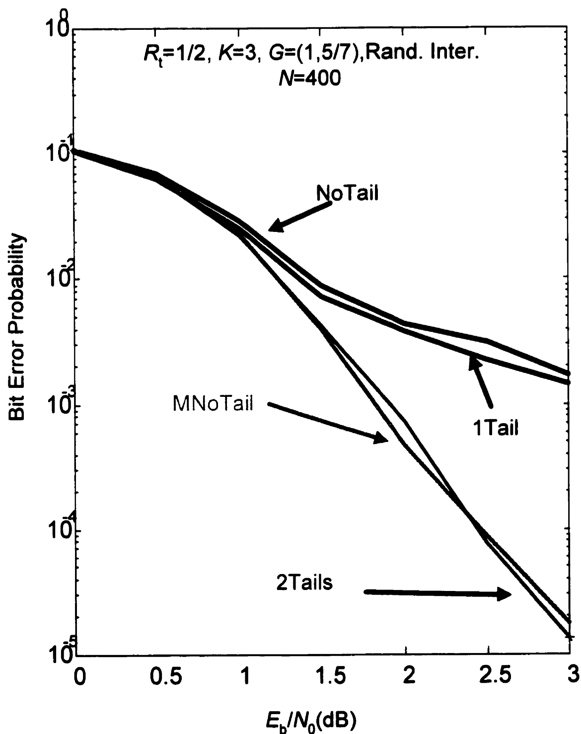
Figure 5.5: Comparaison des quatres alternatives 2Tails , 1Tail , NoTail et MNoTail dans un canal AWGN, pour K = 3 , R_t = 1/2 , N = 400 , Entr. Aléatoire.
