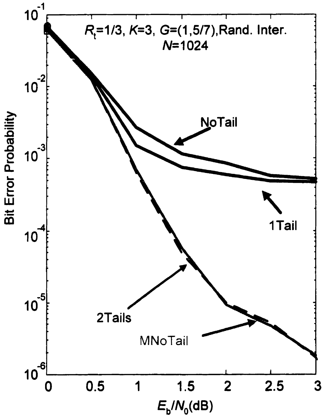
Figure 5.2: Comparaison des quatres alternatives 2Tails , 1Tail , NoTail et MNoTail dans un canal AWGN, pour K = 3 , R_t = 1/3 , N = 1024 , Entr. Aléatoire.
