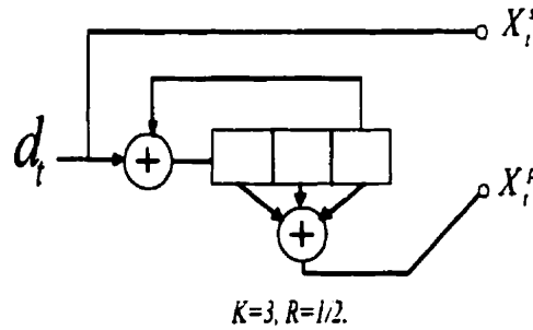
Figure 2.3: Codeur Systématique et Récursif (RSC) de matrice génératrice G(D) = \begin{bmatrix} 1 & \frac{1+D+D^2}{1+D^2} \end{bmatrix}
