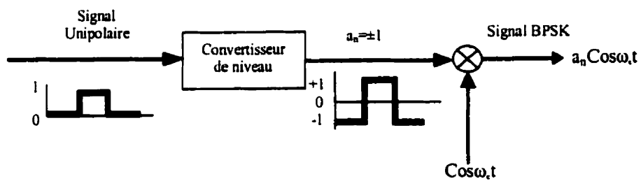
Figure 2.10: Modulateur BPSK
