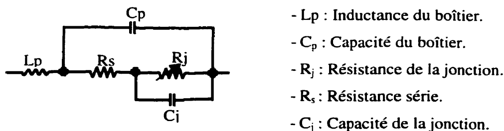
Figure 4.4: Circuit équivalent de la diode schottky.
