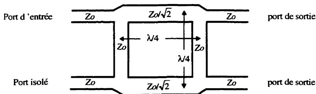
Figure 5.12 : Géométrie du coupleur hybride quadratique.
