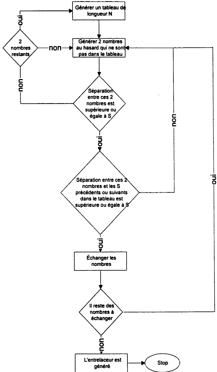
Figure 5.13 – Algorithme de l'entrelaceur symétrique S
