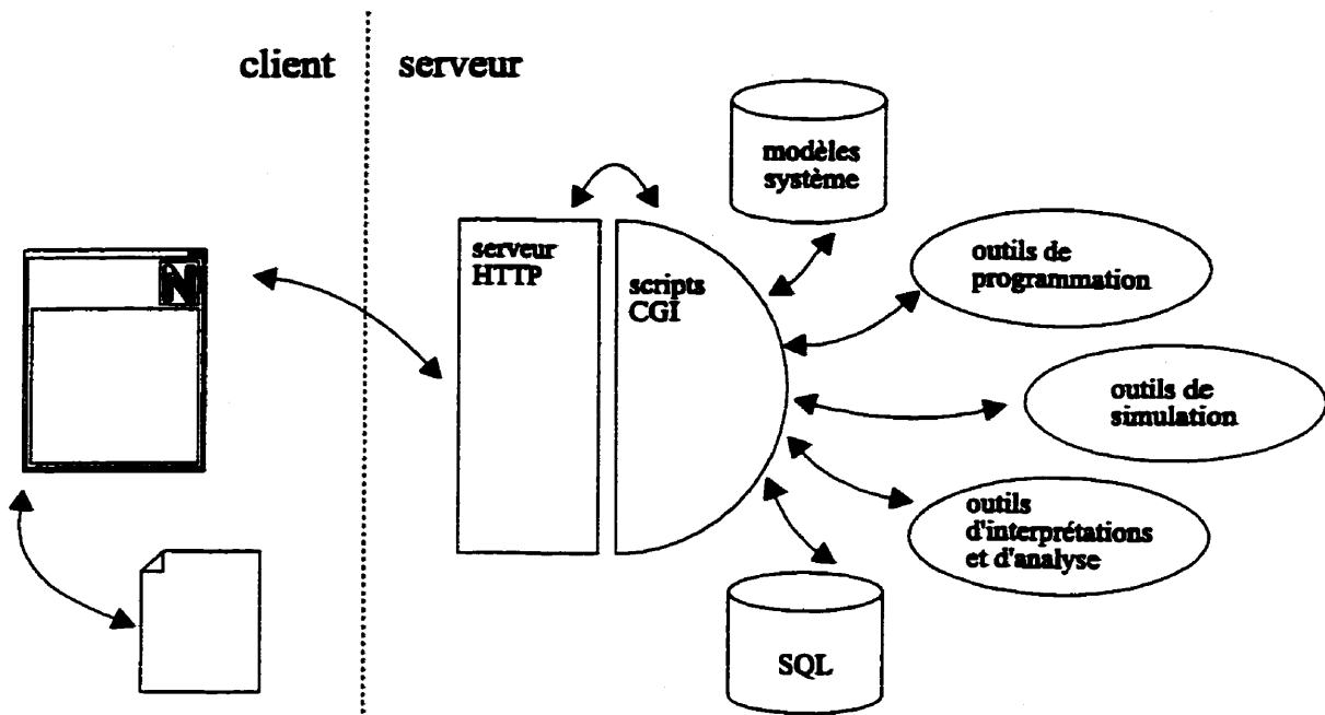
Figure 3.3: Modèle de fonctionnement du SimPULSE-CGI
