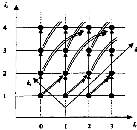
Figure 2.1: Domaine d'itération du filtre IIR 1D
