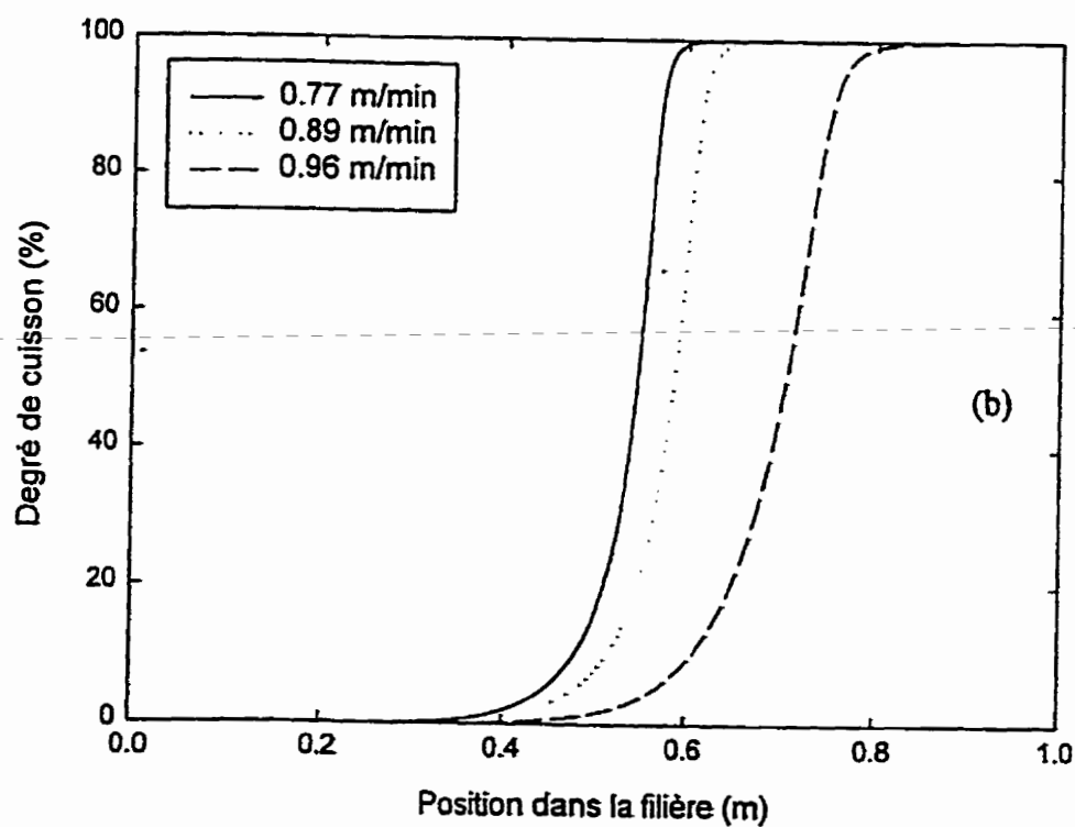
Figure 4.12: Effet de la vitesse sur le degré de conversion simulé au centre du profilé (a) Polyester, (b) Epoxy
