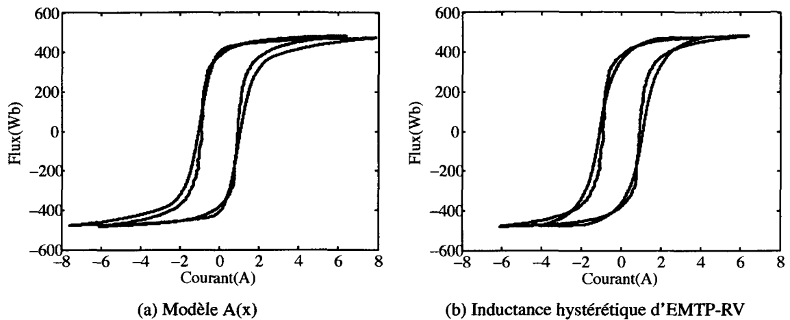
Figure 6.3 Résultats pour le régime permanent à 1,0 pu
