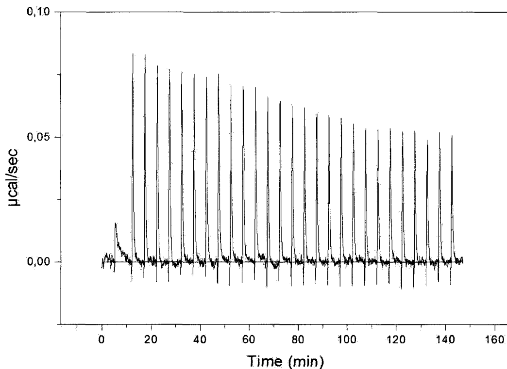
Figure 22. Pics de dégagement de chaleur pour la dilution du chitosane 326,4 \mu\text{g/ml} dans du tampon MES pH 6.0.
