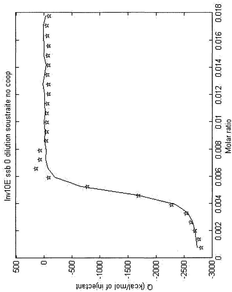
Figure 7. Interpolations par le modèle Mc Gee Van Hippel non coopératif des isothermes obtenus avec le peptide 10E non marqué 0.018 mM (1er essai). Les étoiles rouges représentent les données expérimentales et le trait bleu l'interpolation
