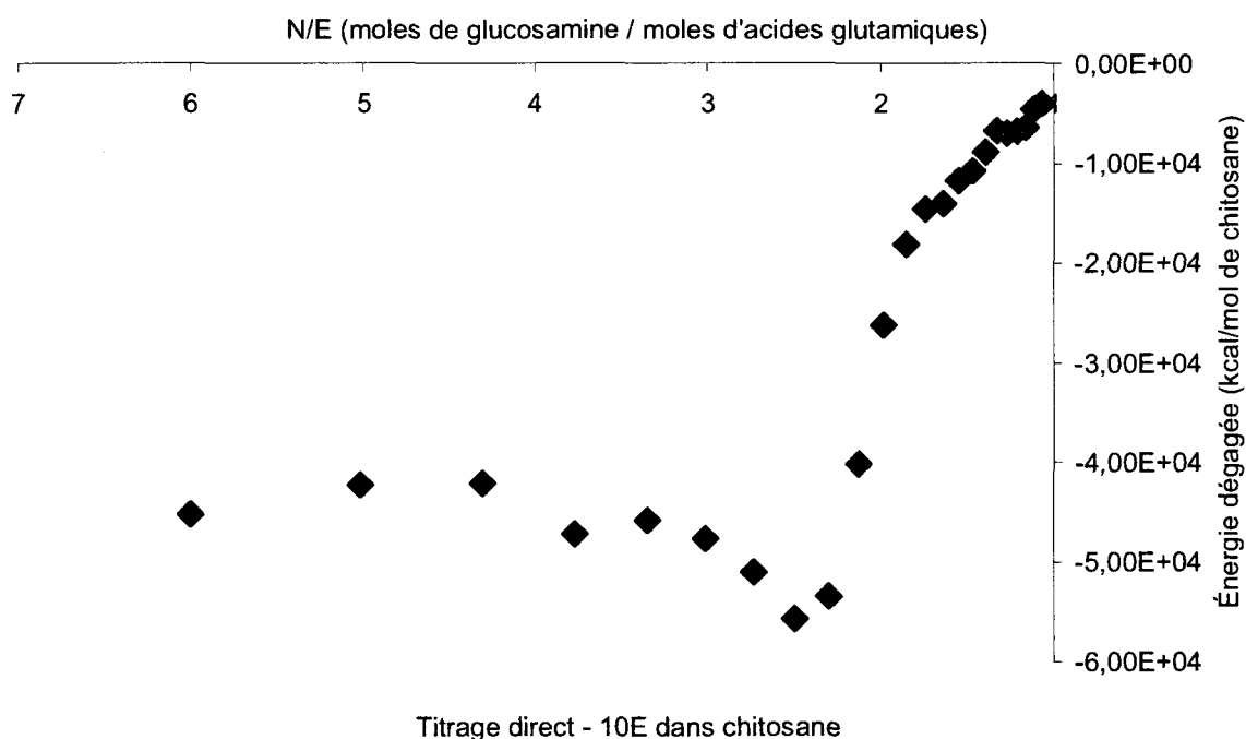
Figure 20. Isotherme de l'injection de peptide 10E 35 \mu\text{g/ml} dans une solution de chitosane concentrée 20.4 \mu\text{g/ml} . Le tampon utilisé était du MES pH 6.0.
