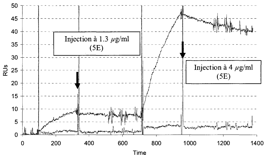
Figure 19. Comparaison des injections sur une surface de chitosane de concentrations 1.3 \mu\text{g/ml} et 4 \mu\text{g/ml} de peptide 5E (courbe rouge supérieure) et de 0.7 \mu\text{g/ml} et 2 \mu\text{g/ml} pour le peptide témoin (courbe verte inférieure). La surface référence était laissée nue. Les flèches bleues désignent la fin de l'injection (phase d'association) et le début d'injection de tampon (phase de dissociation).
