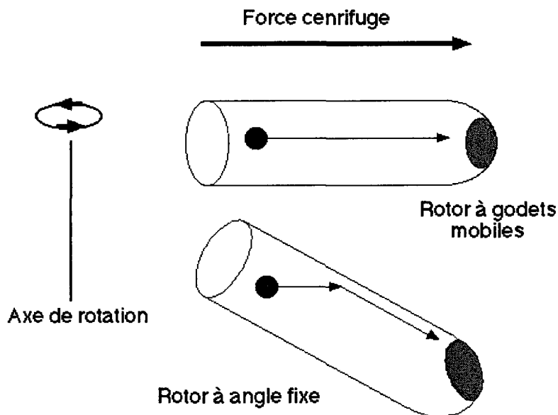
Figure 42. Distribution de particules dans une ultracentrifugation rotor fixe / mobile
