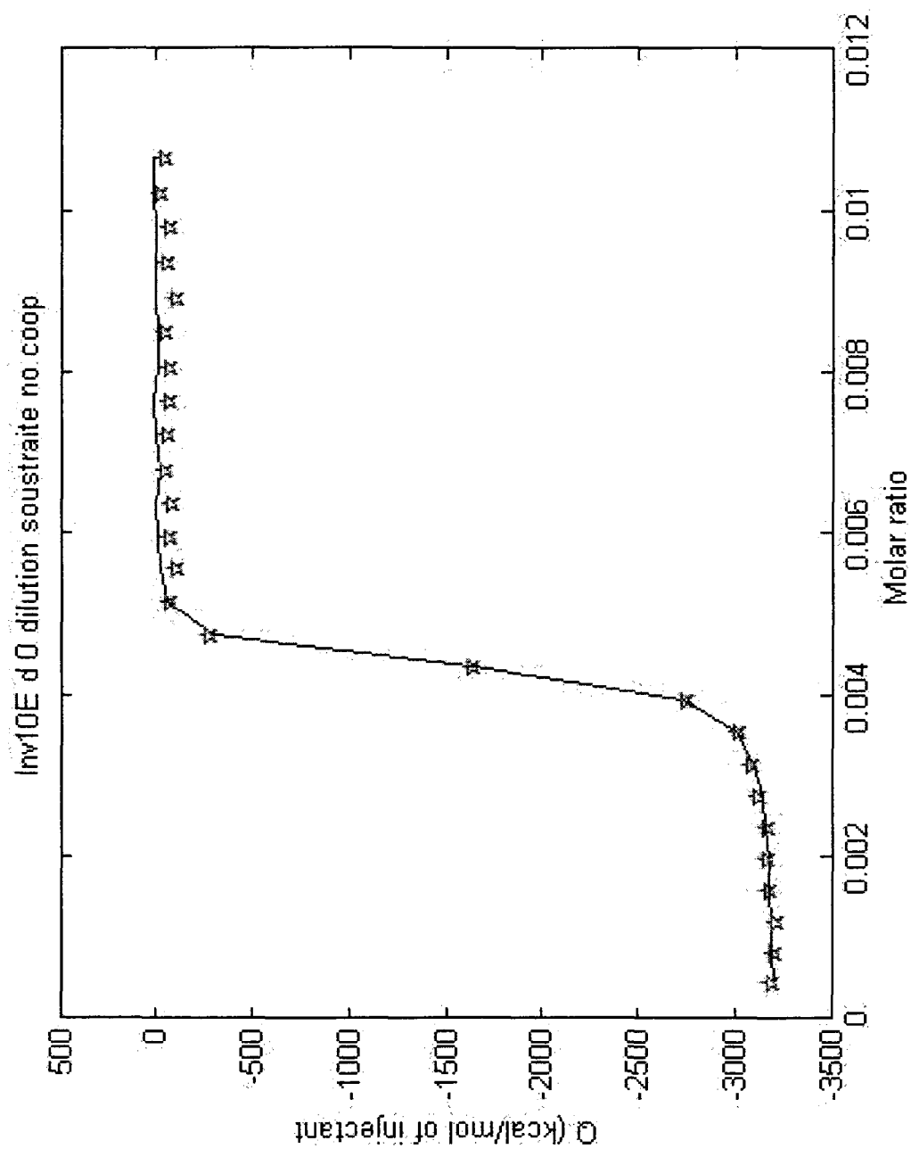
Figure 5. Interpolations des isothermes obtenus avec le modèle Mc Gee Van Hippel pour le peptide 10E 0.03 mM (2ème essai). Les étoiles rouges représentent les données expérimentales et le trait bleu l'interpolation..
