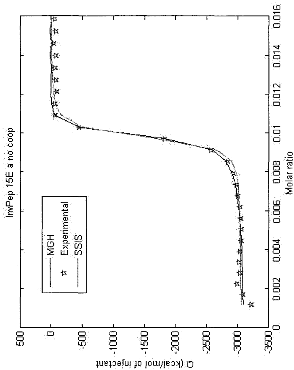
Figure 11. Interpolations par le modèle Mc Gee Van Hippel non coopératif des isothermes obtenus avec le peptide 15E non marqué 0.021 mM. L'interpolation par le modèle SSIS est ajoutée pour comparaison
