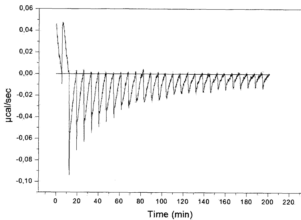
Figure 21. Pics de dégagement de chaleur obtenus pour la dilution du peptide 10E 35 \mu\text{g/ml} dans du MES pH 6.0
