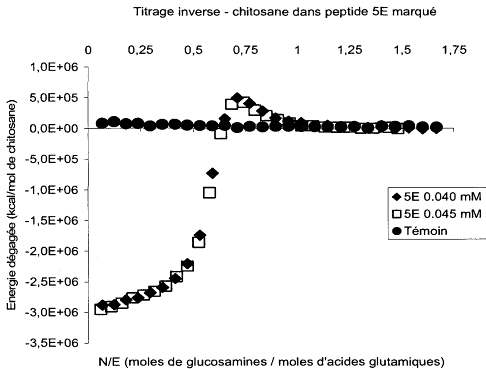
Figure 23. Isothermes du peptide 5E étiqueté. Les concentrations étaient de 0.040 mM (losanges) et de 0.045 mM (carrés) dans le MES à pH 6.0 qui servait également de référence. Le témoin avait pour concentration 0.040 mM (ronds).
