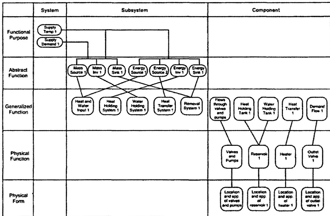
Figure 4.3 – Application de la hiérarchie d'abstraction et de décomposition au contrôle d'un processus thermo-hydraulique (Vicente 1999a, p. 175).
