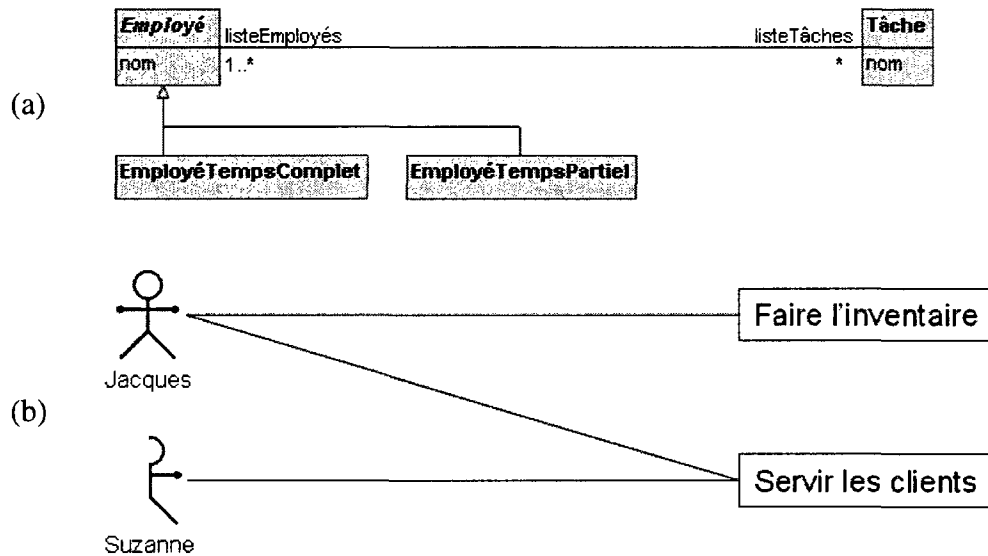
Figure 2.7 – Nouveau langage de modélisation pour l'assignation de tâches : (a) la syntaxe abstraite et (b) la syntaxe concrète.
