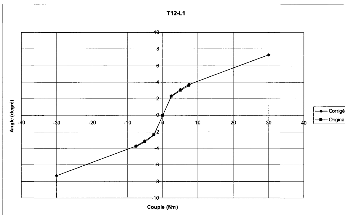
Figure B-9 Courbe expérimentale en inflexion latérale T11-T12
