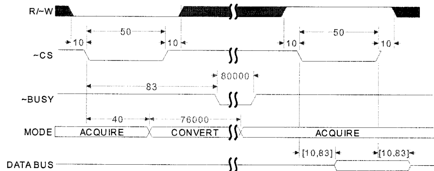
Figure 3.7 Chronogramme d'une lecture de l'ADC (temps en ns )
