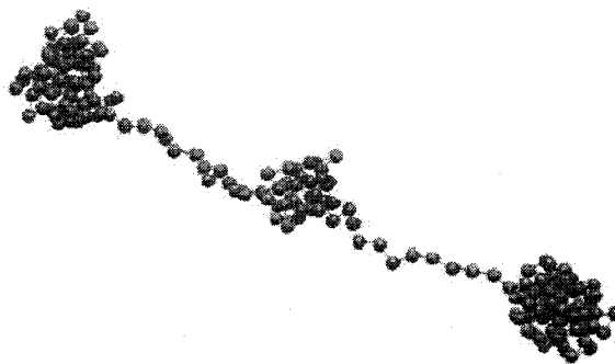
Figure 2.14 Représentation schématique d'une conformation de type collier caractéristique d'un polyelectrolyte solubilisé dans un mauvais solvant (Dobrynin et al., 1996).
