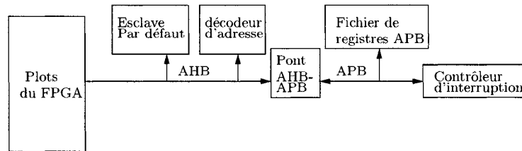
Figure 2.12: Configuration intérieure AHB du FPGA
