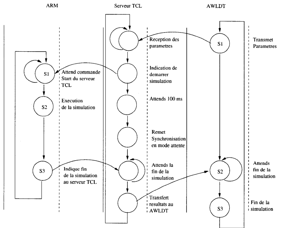
Figure 4.3: Diagramme du communication entre les différents paliers de la plateforme matérielle-logicielle
