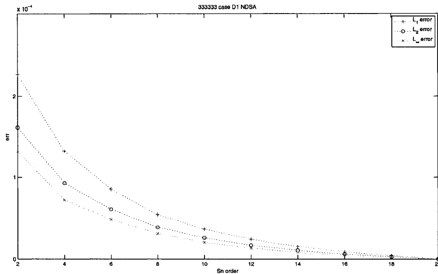
FIG. 3.14 Cas 333333 : évolution de l'erreur en fonction du raffinement angulaire pour les flux surfaciques
