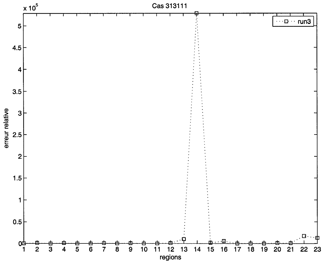
FIG. 3.27 Erreur relative : cas 313111
