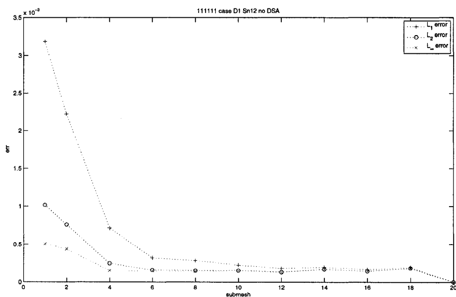
FIG. 3.7 Cas 111111 : évolution de l'erreur en fonction du raffinement spatial pour les flux scalaires
