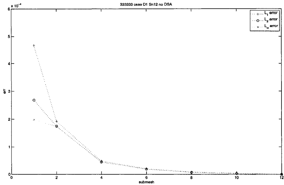
FIG. 3.11 Cas 333333 : évolution de l'erreur en fonction du raffinement spatial pour les flux scalaires
