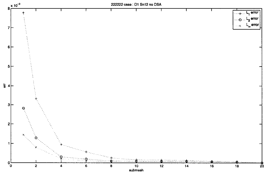
FIG. 3.3 Cas 222222 : évolution de l'erreur en fonction du raffinement spatial pour les flux scalaires
