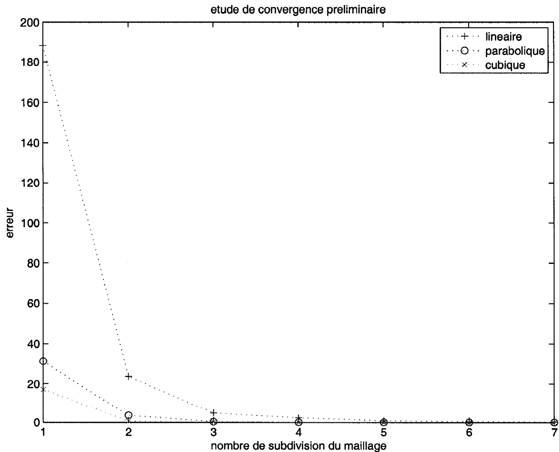
FIG. I.1 Etude de convergence monotonique
