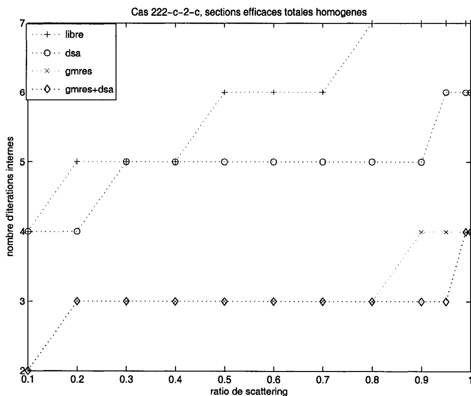
FIG. 2.5 Test GMRES et DSA : cas 222-c-2-c
