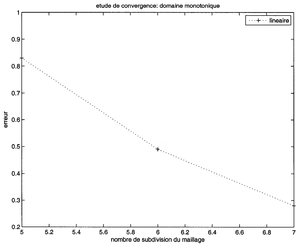
FIG. I.2 Erreur relative pour le cas linéaire
