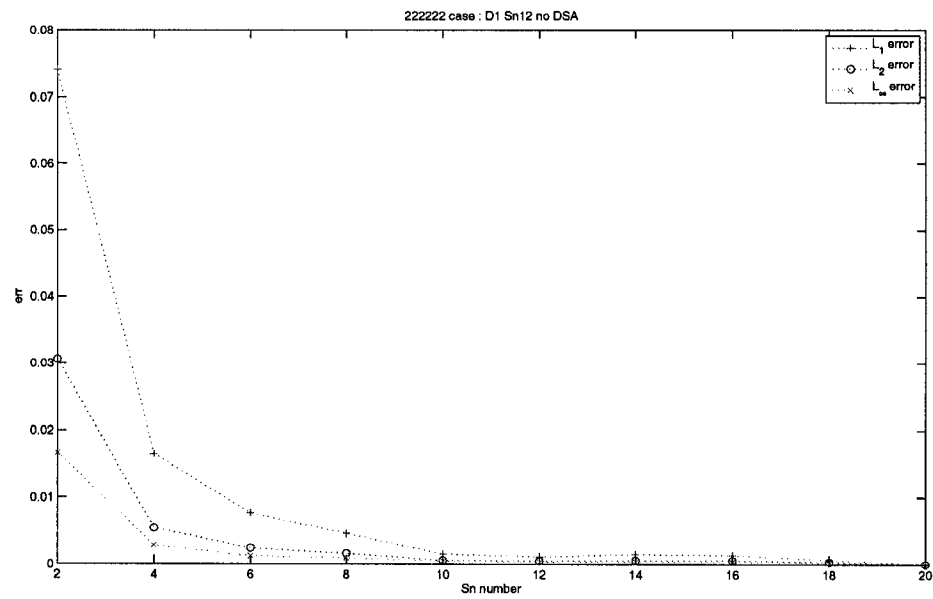
FIG. 3.4 Cas 222222 : évolution de l'erreur en fonction du raffinement angulaire pour les flux scalaires
