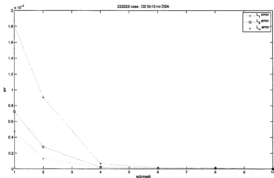
FIG. 3.15 Cas 222222 : évolution de l'erreur en fonction du raffinement spatial pour les flux scalaires
