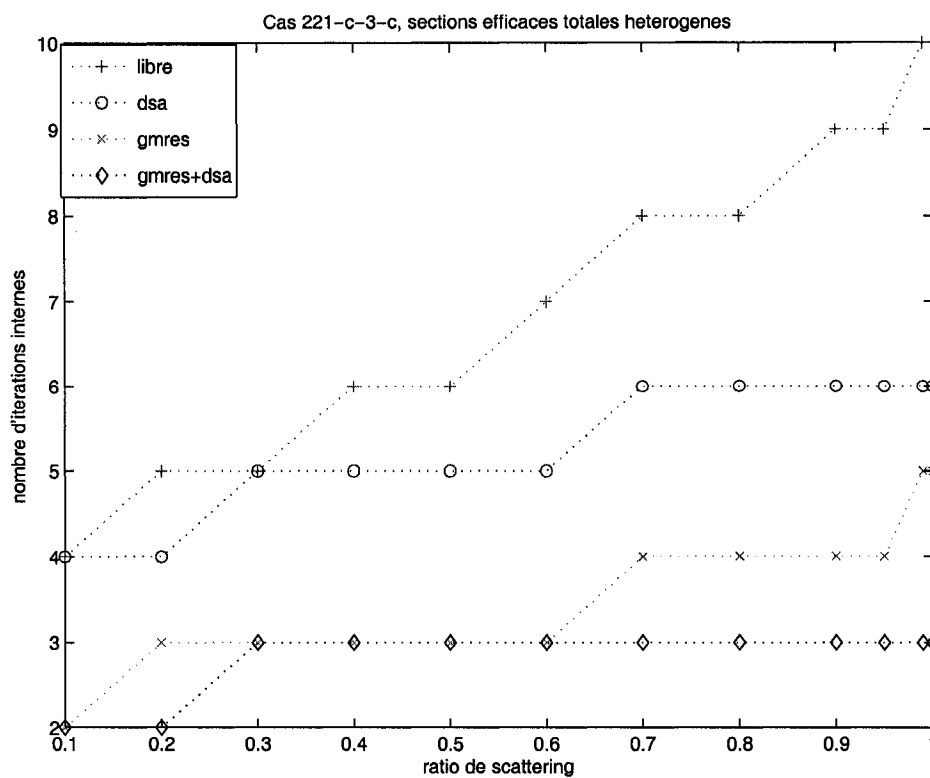
FIG. 2.6 Test GMRES et DSA : cas 221-c-3-c
