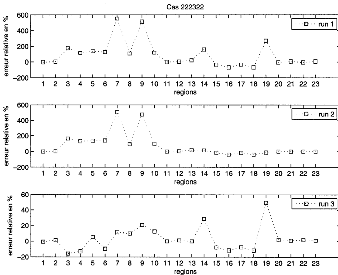
FIG. 3.21 Erreur relative pour le cas 222322
