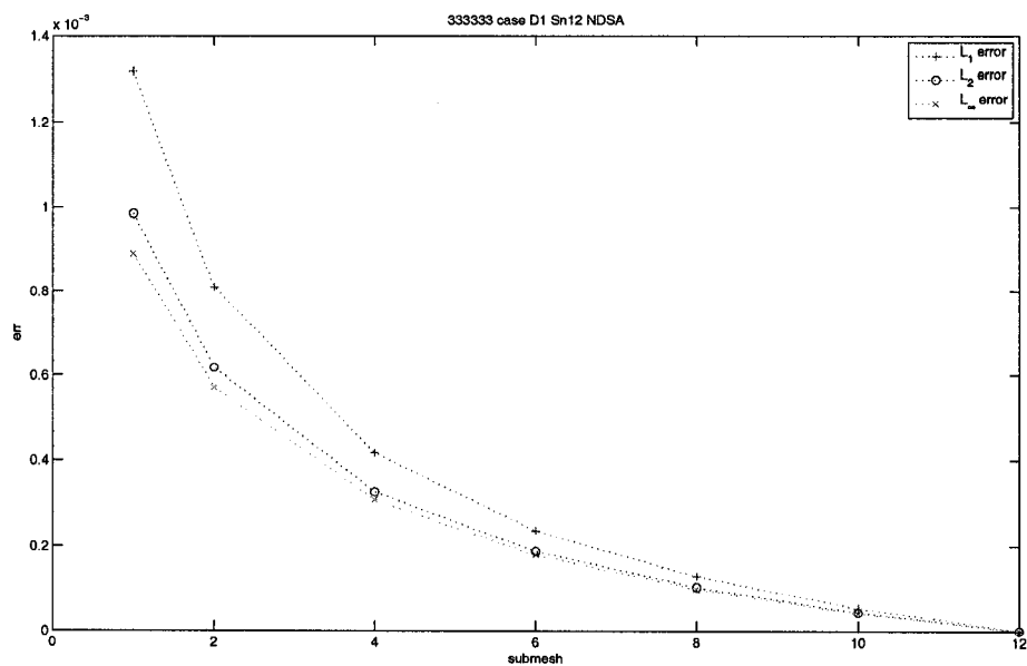
FIG. 3.13 Cas 333333 : évolution de l'erreur en fonction du raffinement spatial pour les flux surfaciques
