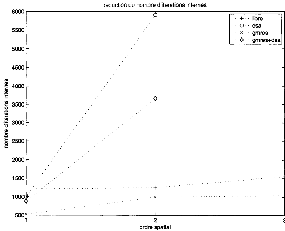
FIG. 2.7 Test GMRES et DSA pour les différents ordres spatiaux : benchmark IAEA3D
