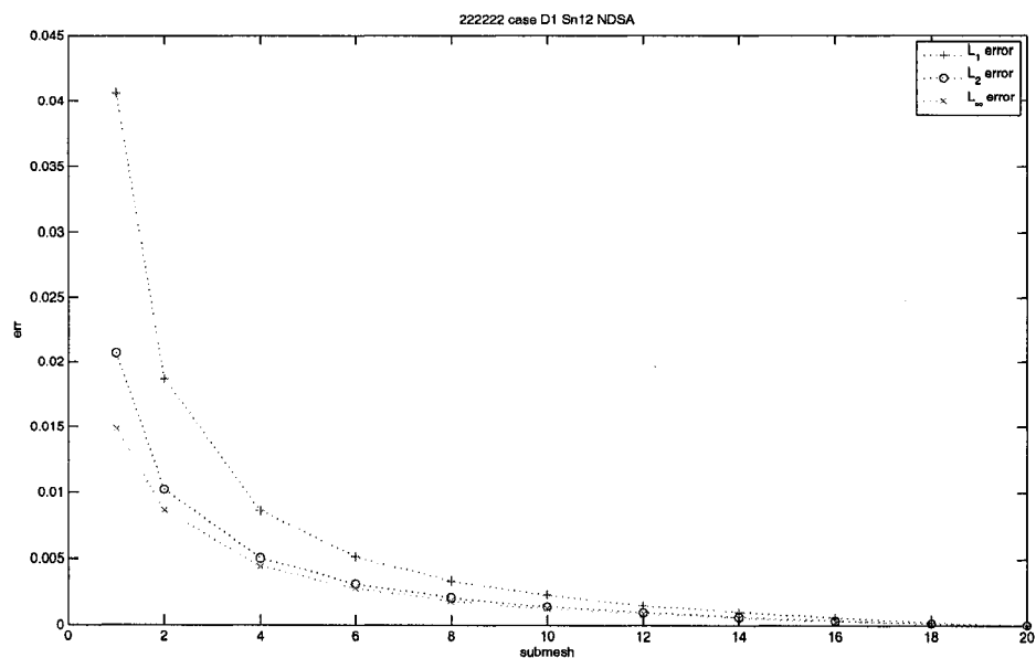
FIG. 3.5 Cas 22222 : évolution de l'erreur en fonction du raffinement spatial pour les flux surfaciques
