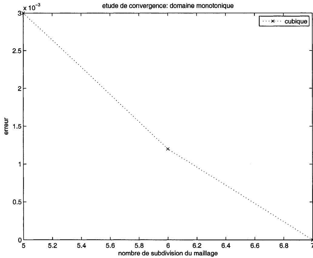
FIG. I.6 Erreur relative pour le cas cubique
