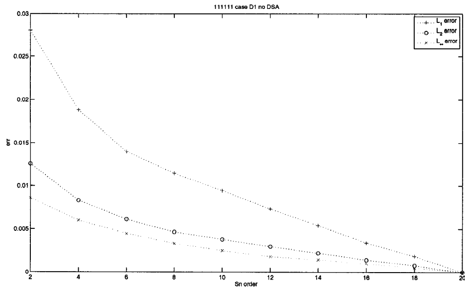
FIG. 3.10 Cas 111111 : évolution de l'erreur en fonction du raffinement angulaire pour les flux surfaciques
