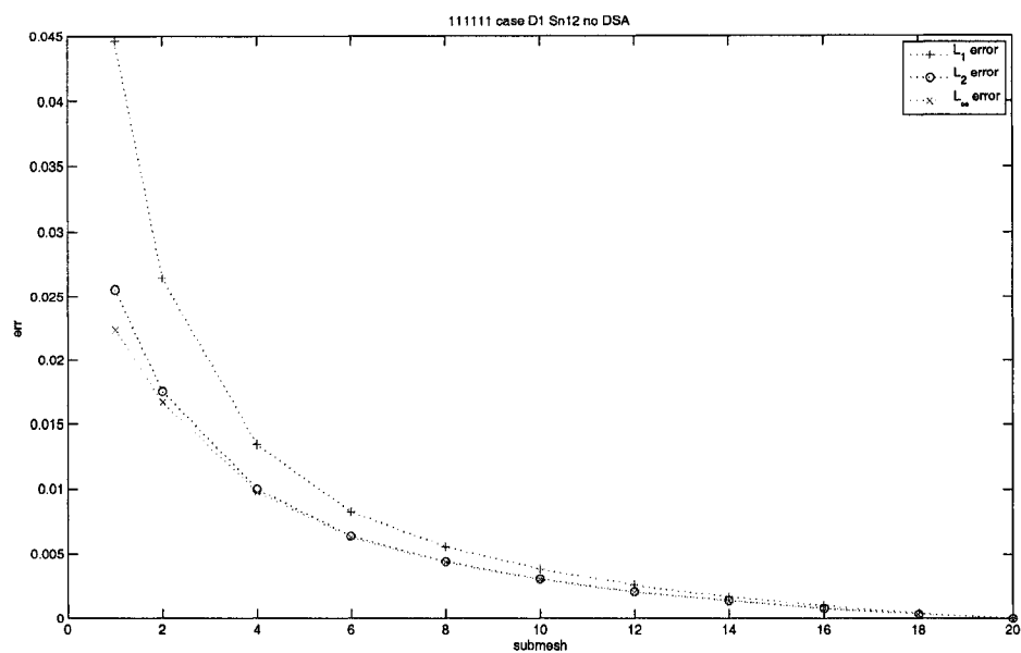
FIG. 3.9 Cas 111111 : évolution de l'erreur en fonction du raffinement spatial pour les flux surfaciques
