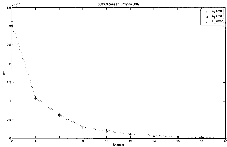
FIG. 3.12 Cas 333333 : évolution de l'erreur en fonction du raffinement angulaire pour les flux scalaires
