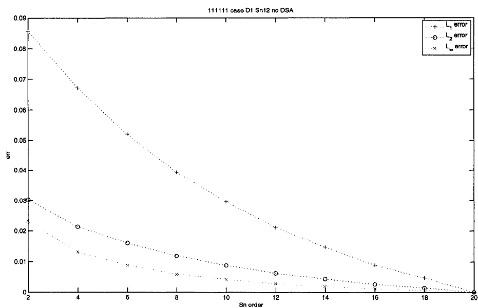
FIG. 3.8 Cas 111111 : évolution de l'erreur en fonction du raffinement angulaire pour les flux scalaires
