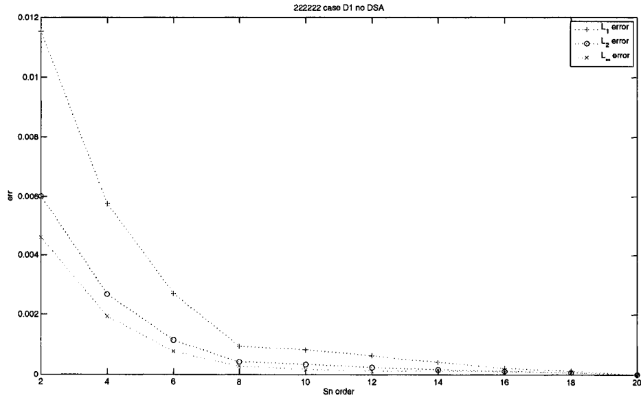
FIG. 3.6 Cas 222222 : évolution de l'erreur en fonction du raffinement angulaire pour les flux surfaciques
