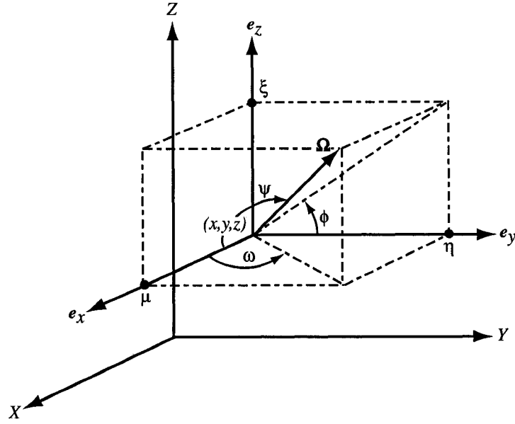
FIG. 1.2 Système de coordonnées 3D cartésien
