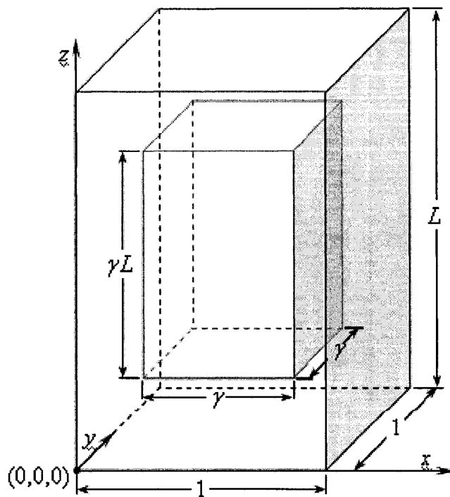
FIG. 3.1 Géométrie du Benchmark NEA 3D
