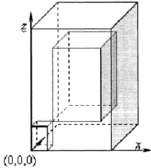
FIG. 3.2 Position de la source unitaire
