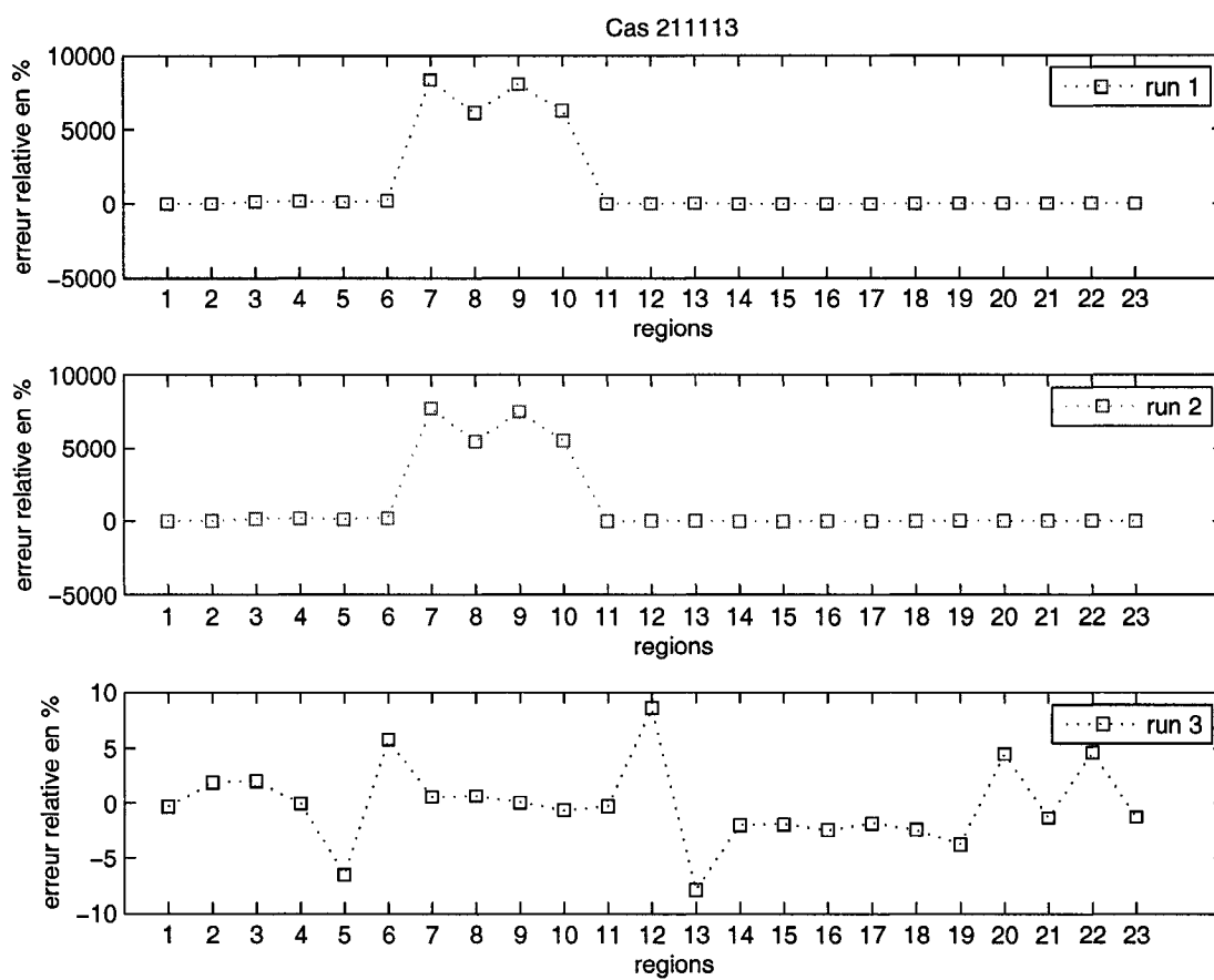
FIG. 3.18 Erreur relative pour le cas 211113
