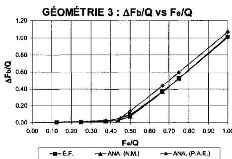
Figure E.5 – Supplément de force relatif à la précontrainte (géométrie 3)
