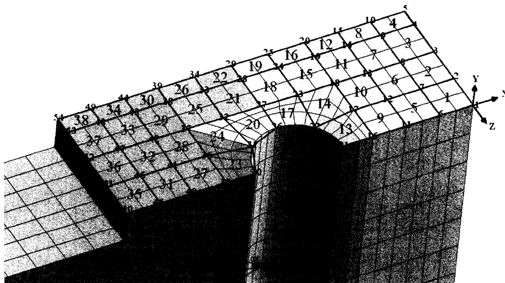
Figure C.2 – Numérotation des noeuds et des éléments au contact
