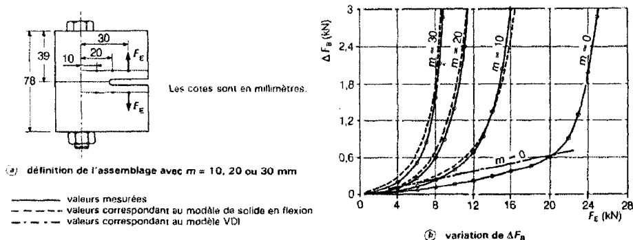
Figure 1.4 – Influence de l'excentration sur le supplément d'effort dans le boulon
