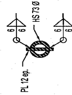
COUPE 1 1:10
