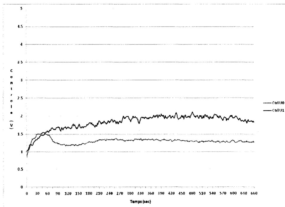
Figure A.5.6 : évolution de la commande pour l'expérience 7
