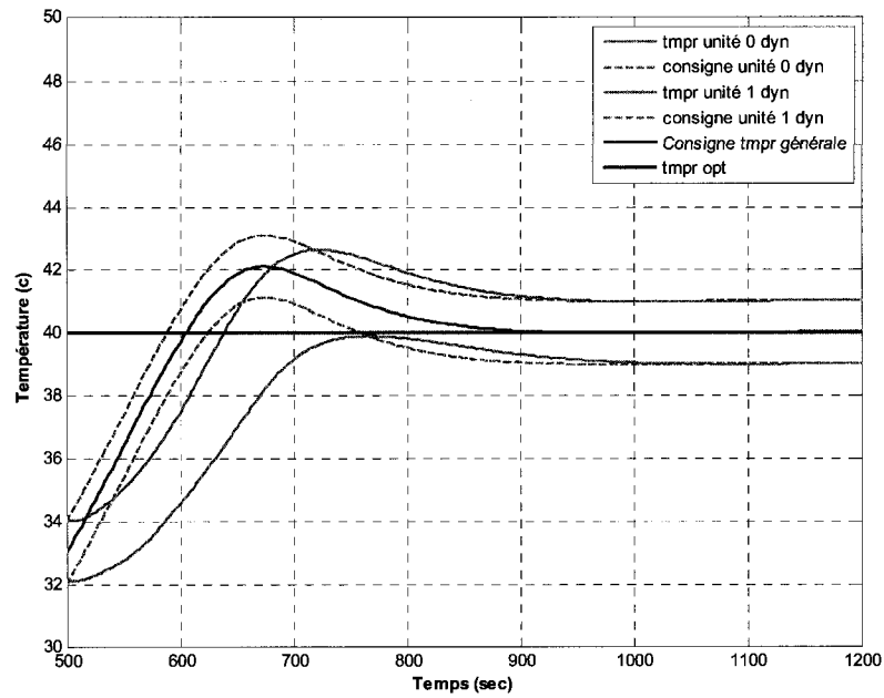
Figure 5.7 : évolution de la température pour la simulation 4
