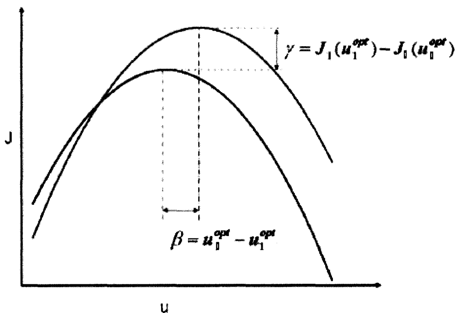
Figure 2.6 : courbe statique non identique entre les unités
