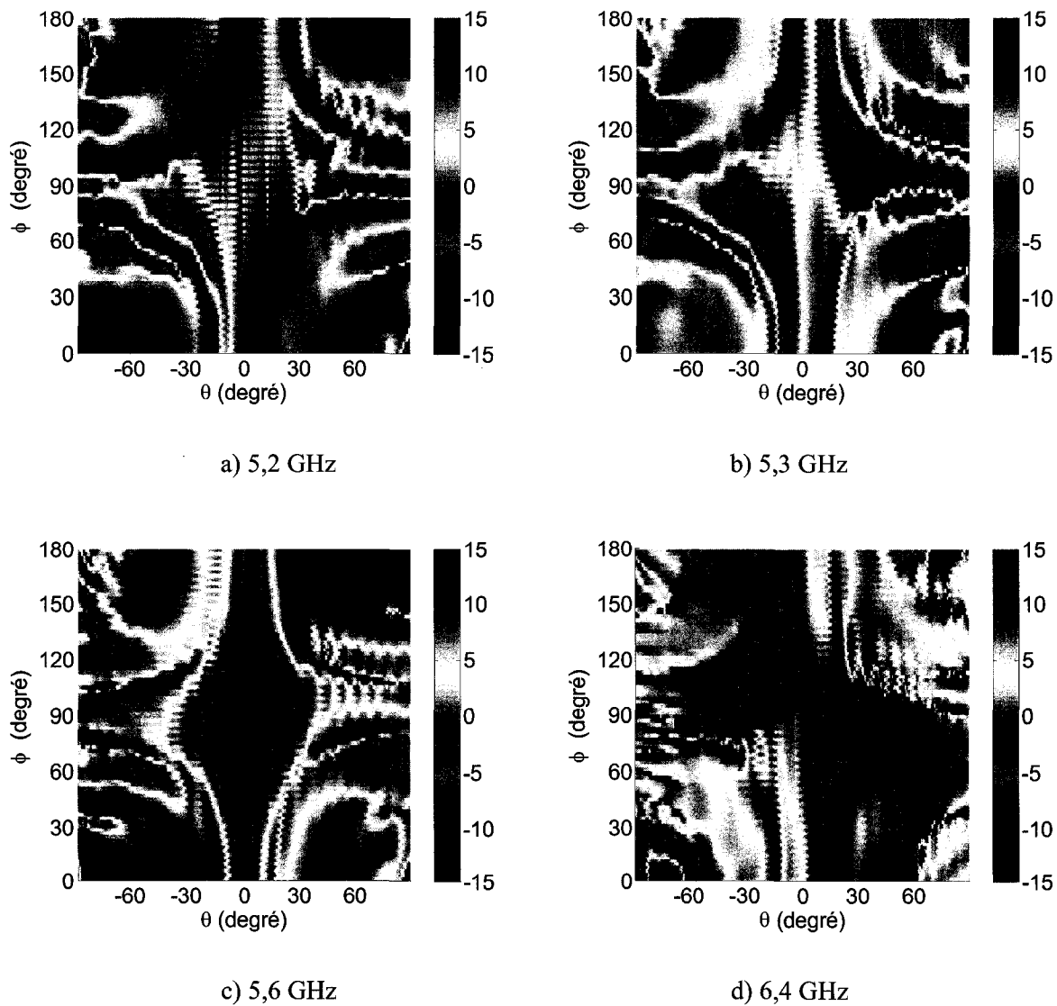
Figure 4-32 Variations de l'amplitude entre l'état ON et OFF en co-polarisation
