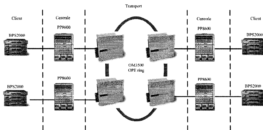
FIGURE 4.3 Connectivité : Nortel
