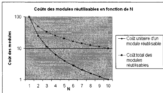
FIGURE 4.30 Coût des modules réutilisables en fonction du nombre de modules
