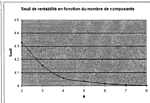
FIGURE 4.60 Coût de réutilisation en fonction du nombre de composants FIGURE 4.61 Seuil en fonction du nombre de composants
