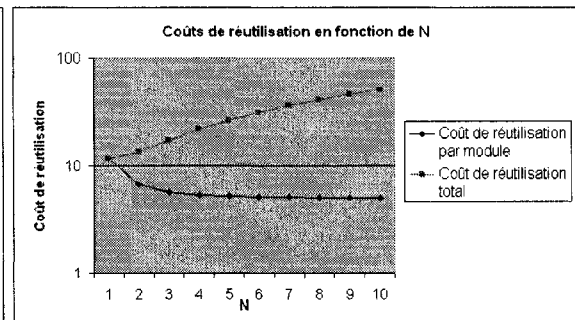
FIGURE 4.30 Coût des modules réutilisables en fonction du nombre de modules
