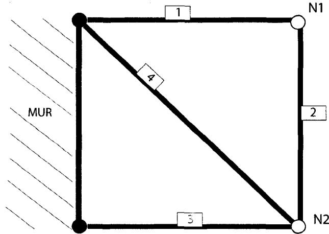
Figure 1.14 – Treillis initial à 5 barres (diamètres = 50)
