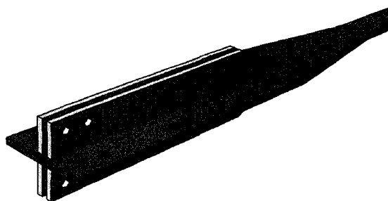
Figure 9.2: Détail des raidisseurs d'extrémité du noyau
