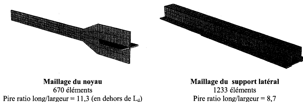
Figure 5.33 : Maillage des éléments du modèle
