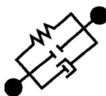
Figure 5.23 : Lien de modélisation des boulons
