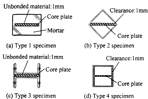
Figure 3.5: Systèmes comparés par Iwata et al. (2000)
