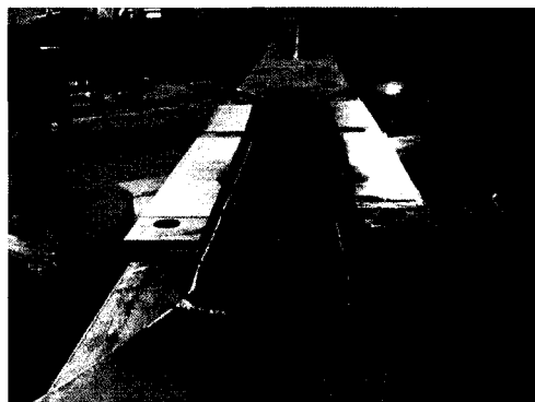
Figure 3.9: État du noyau du spécimen S2-1 à la fin du test (Bolduc et Tremblay 2003)
