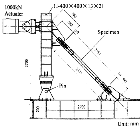
Figure 3.6: Banc d'essais de Iwata et al. (2000)
