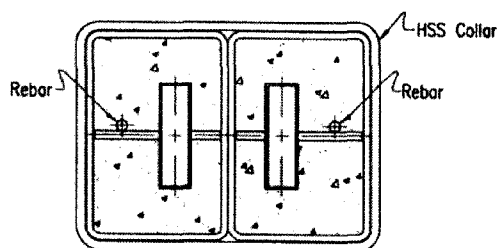
Figure 3.23: Combinaison de deux diagonales Star Seismic (Merritt 2003)
