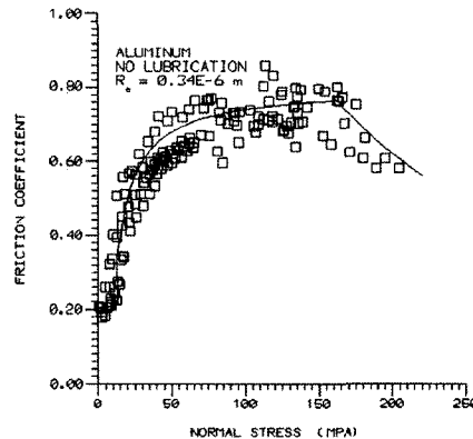
Figure 5.26 : Coefficient de friction aluminium-acier selon la pression (tiré de Javadi 2006)
