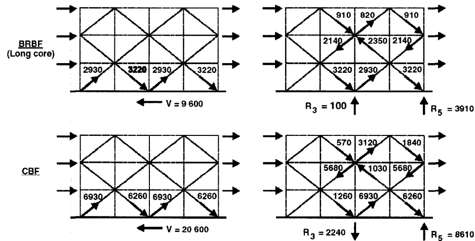
Figure 2.2: Calcul par capacité partiel pour DDC et cadres concentriques (Tremblay et al. (2004))
