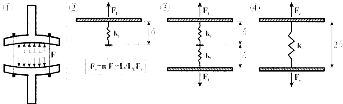
Figure 7.2: Schéma explicatif pour la rigidité équivalente
