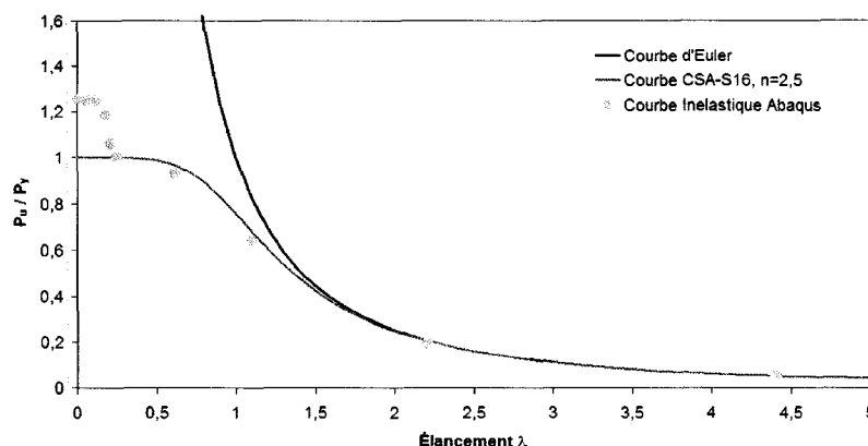
Figure C.2: Courbes de flambement
