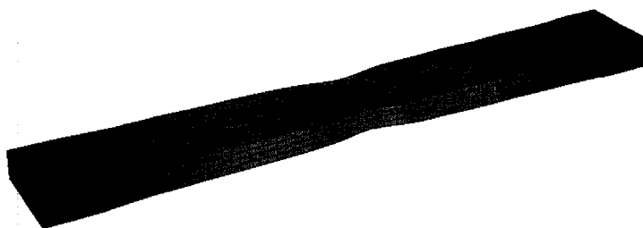
Figure 5.5 : Striction du coupon numérique – maillage cubique à interpolation linéaire
