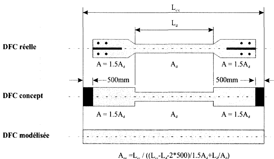
Figure A.2: DDC et aires équivalentes
