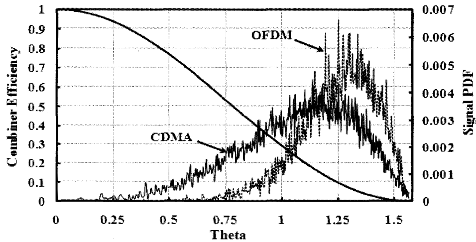
Figure 5: L'efficacité du Combineur hybride et PDF pour signaux modulés OFDM et CDMA vs. l'angle de décomposition \theta .
