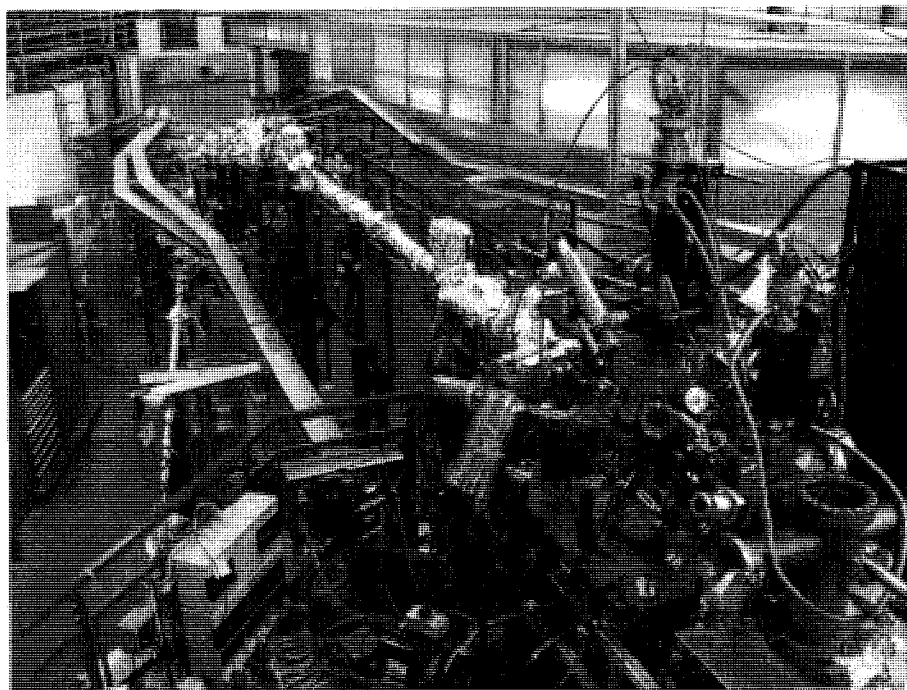
FIGURE 2.8 Montage expérimental pour le NEXAFS et sa ligne de faisceau. Synchrotron BESSY II à Berlin, Allemagne.
