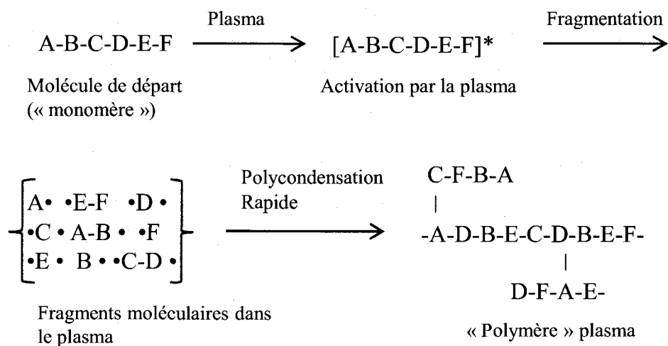
FIGURE 1.3 Concept général la formation des polymères plasma.
