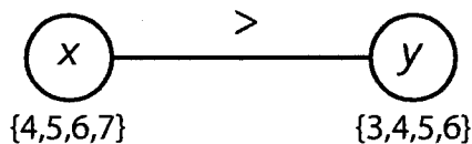
Figure 2.4 – Exemple d'une contrainte binaire arc-cohérente.
