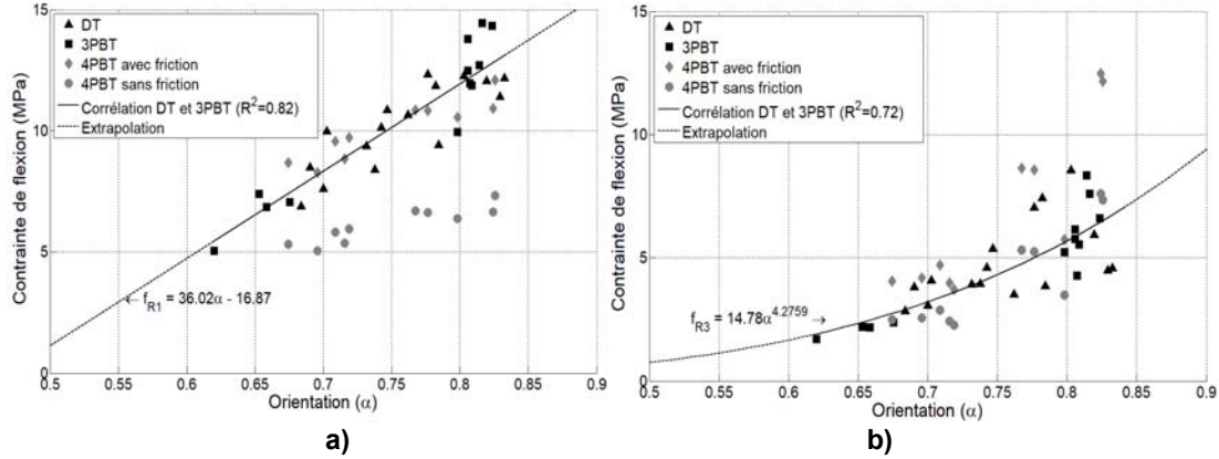
Figure 6. Impact de l'orientation des fibres sur les contraintes résiduelles, a) f_{R1} , b) f_{R3}
