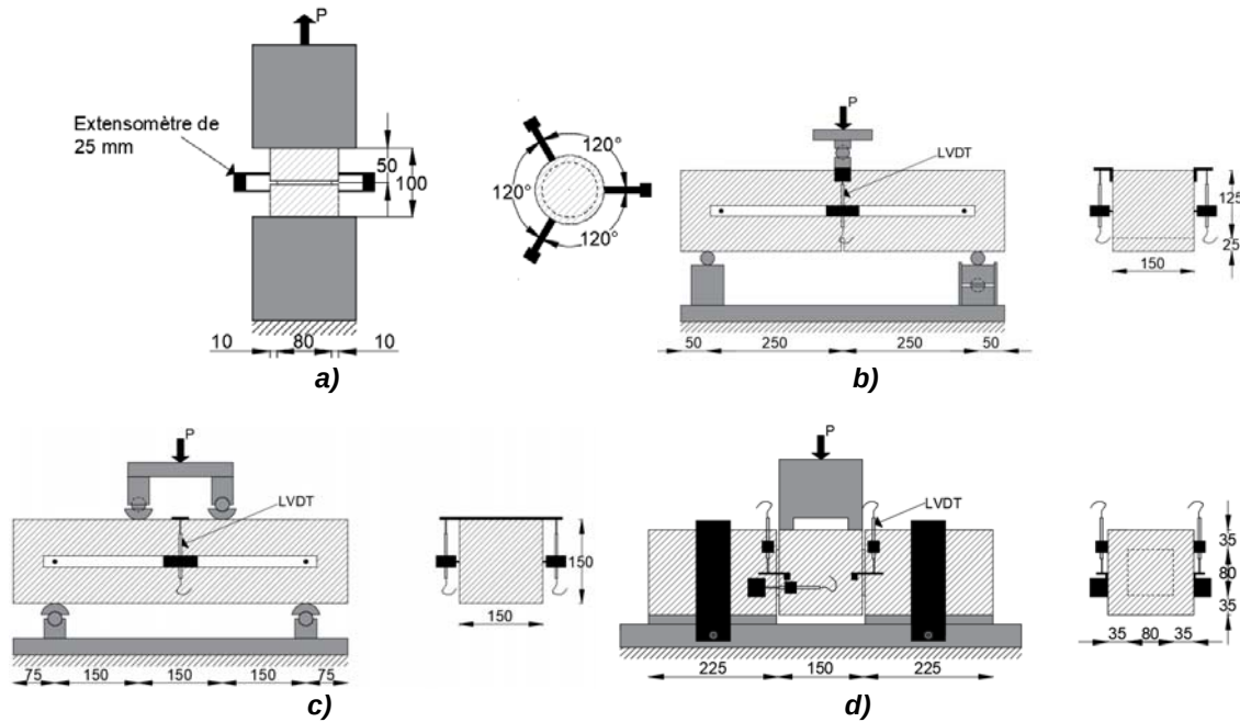
Figure 2. Montage et géométrie des essais, a) Essai de traction directe, b) Essai de flexion en trois points, c) Essai de flexion en quatre points, d) Essai de cisaillement
