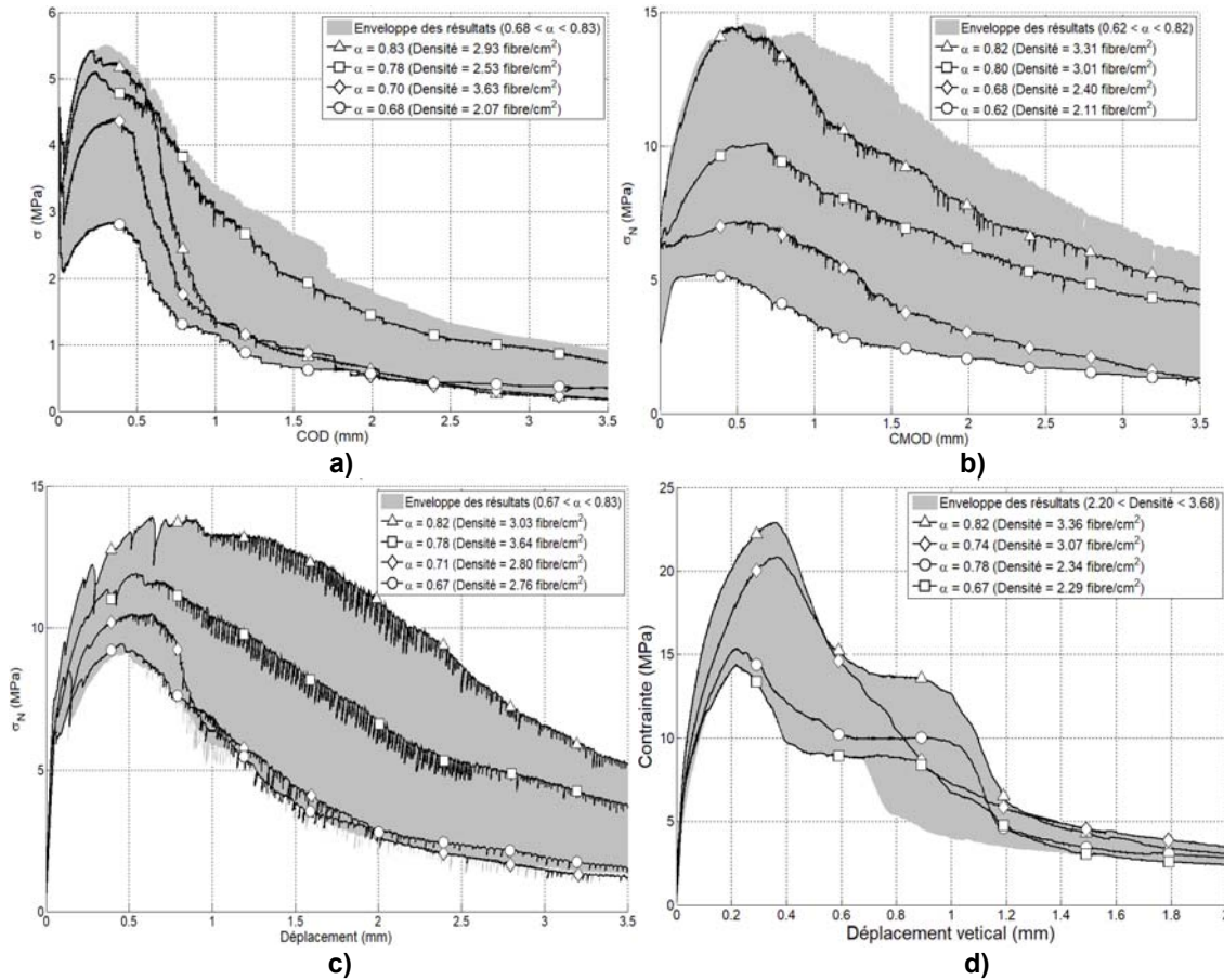
Figure 4. Résultats d'essais, a) traction directe (DT), b) flexion en trois points (3PBT), c) flexion en quatre points (4PBT), d) cisaillement
