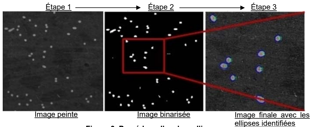
Figure 3. Procédure d'analyse d'image
