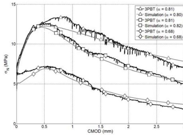
Figure 5. Comparaison entre les comportements simulés et expérimentaux de spécimens soumis à un essai de flexion en trois points
