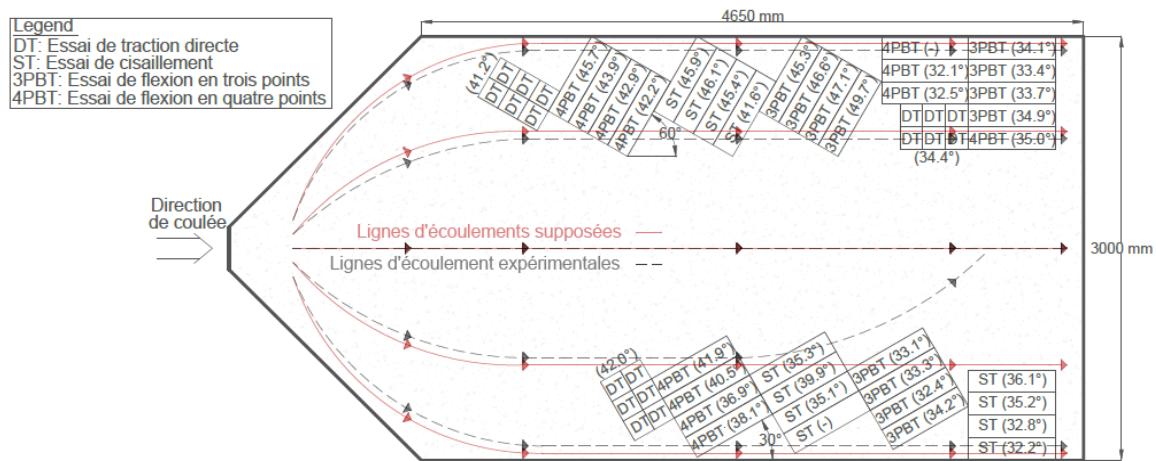
Figure 1. Vue en plan de la dalle expérimentale, localisation des spécimens et orientations des fibres
