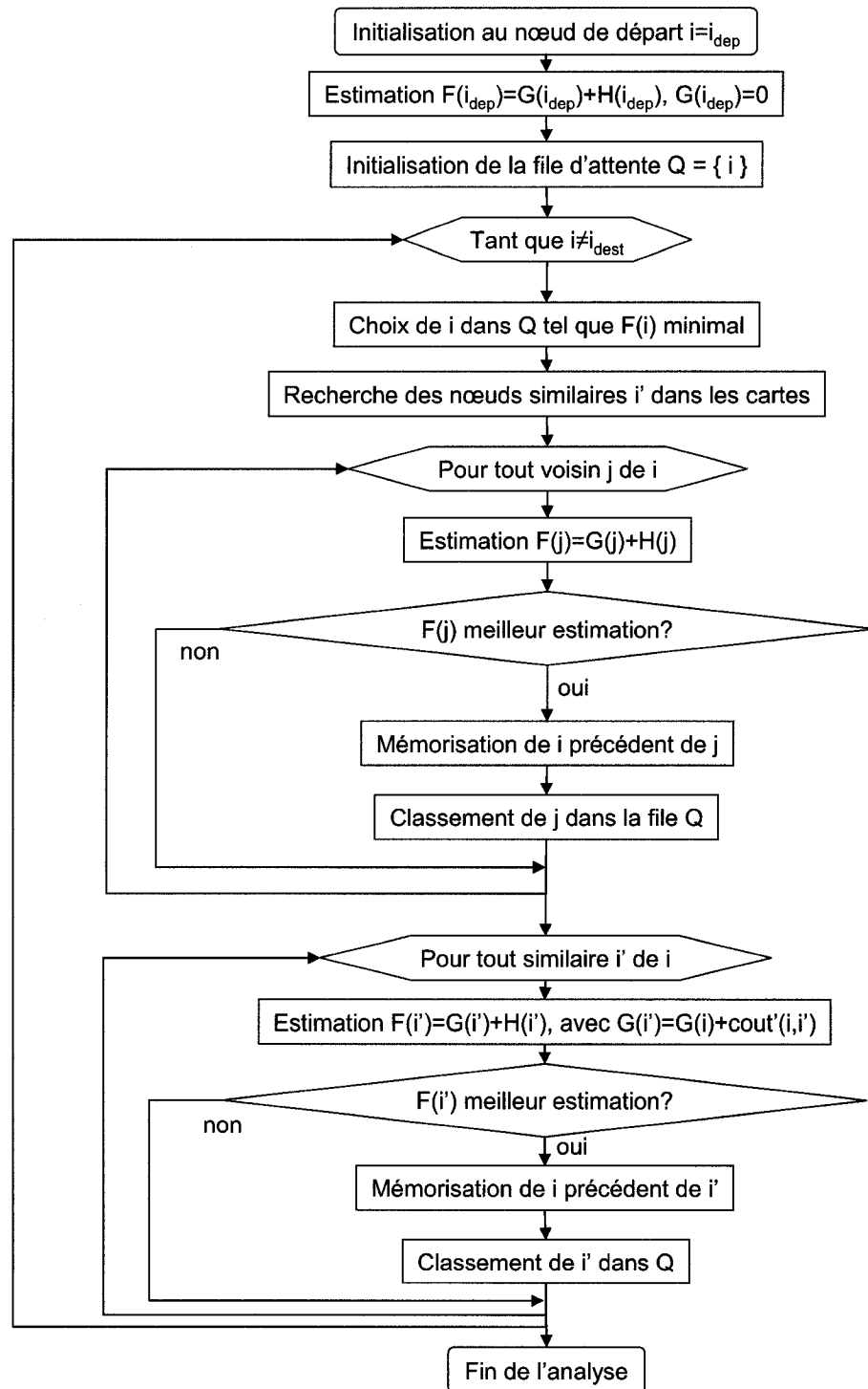
FIG. 2.8 Algorithme d'exploration du graphe
