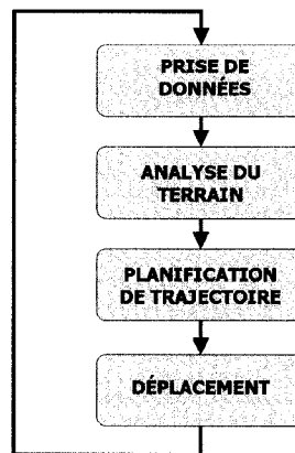
FIG. 2.1 Déroulement d'une séquence de navigation dans un terrain partiellement connu
