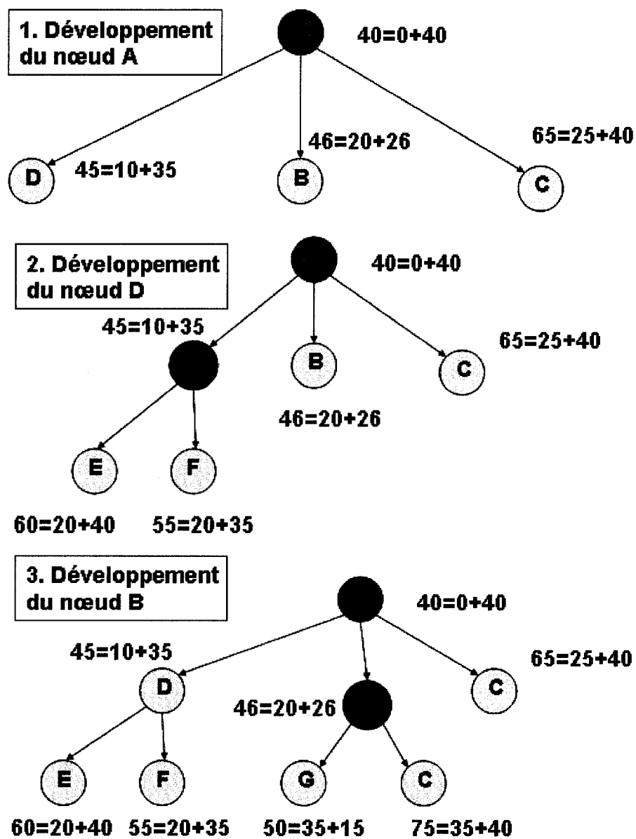
FIG. 2.3 Fonctionnement de l'algorithme A* (1)
