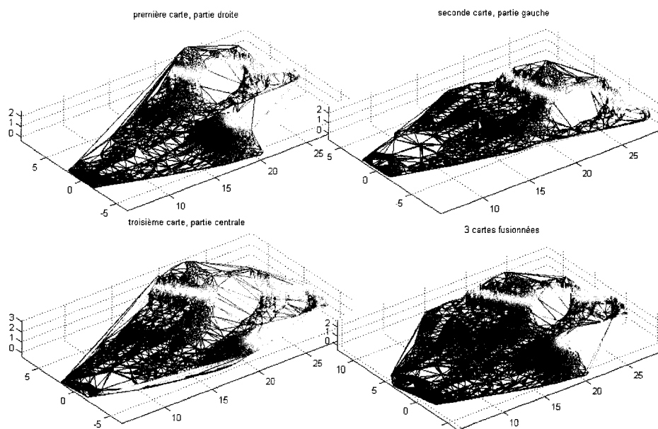
FIG. 1.7 Maillage triangulaire irrégulier, cartes obtenues par le robot
