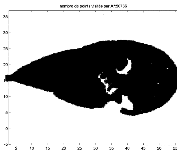
FIG. 2.12 Exemple de zone balayée par A* dans le cas d'un contournement sur une longue distance
