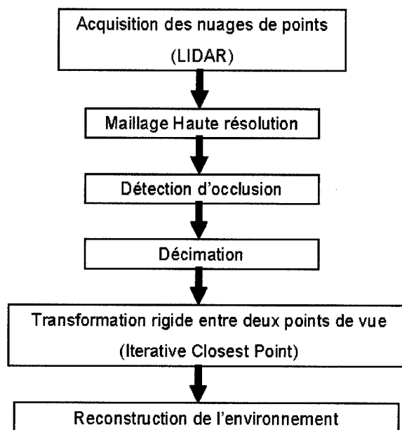
FIG. 1.4 Étapes de construction des cartes
