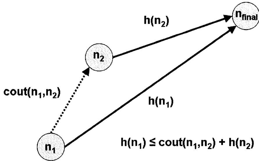
FIG. 2.6 Consistance de l'exploration A*
