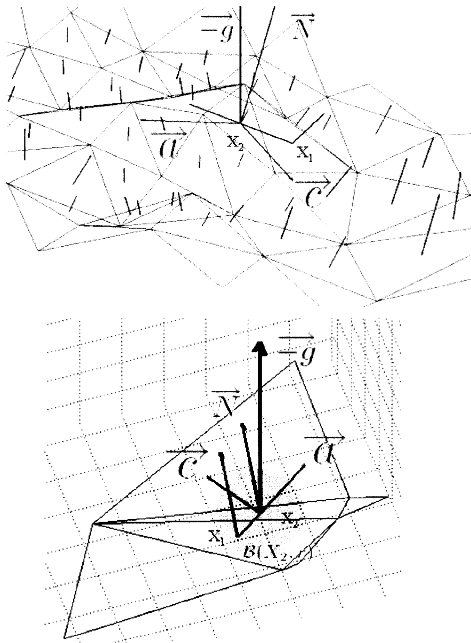
FIG. 3.21 Illustration des vecteurs et angles nécessaires dans le calcul de l'orientation
