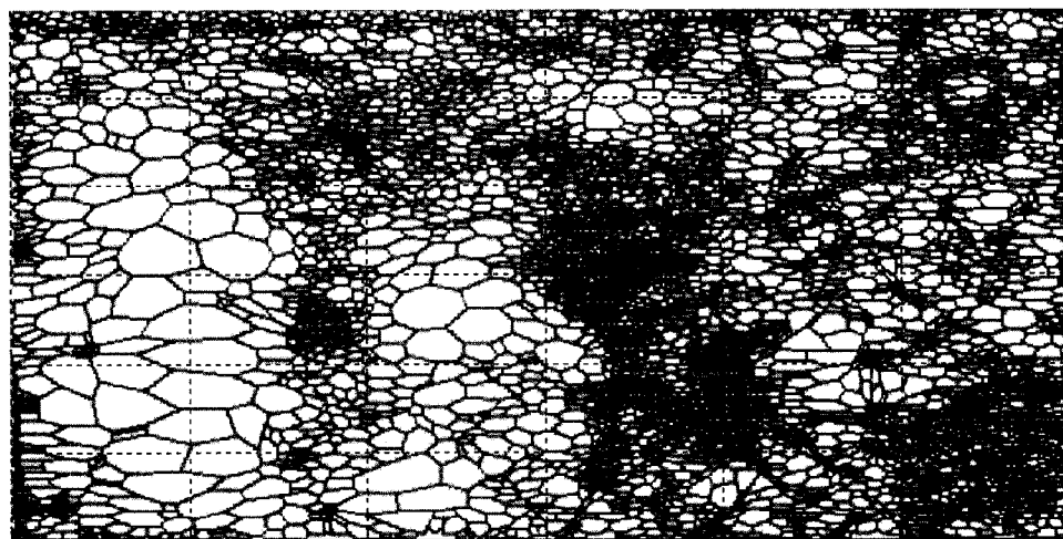
FIG. 3.23 Représentation des valeurs c_6 de la rugosité de plus de 20cm des liens du graphe
