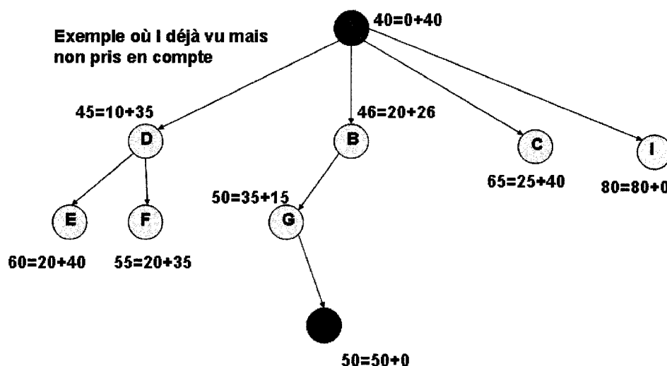
FIG. 2.7 Illustration de l'optimalité de A*
