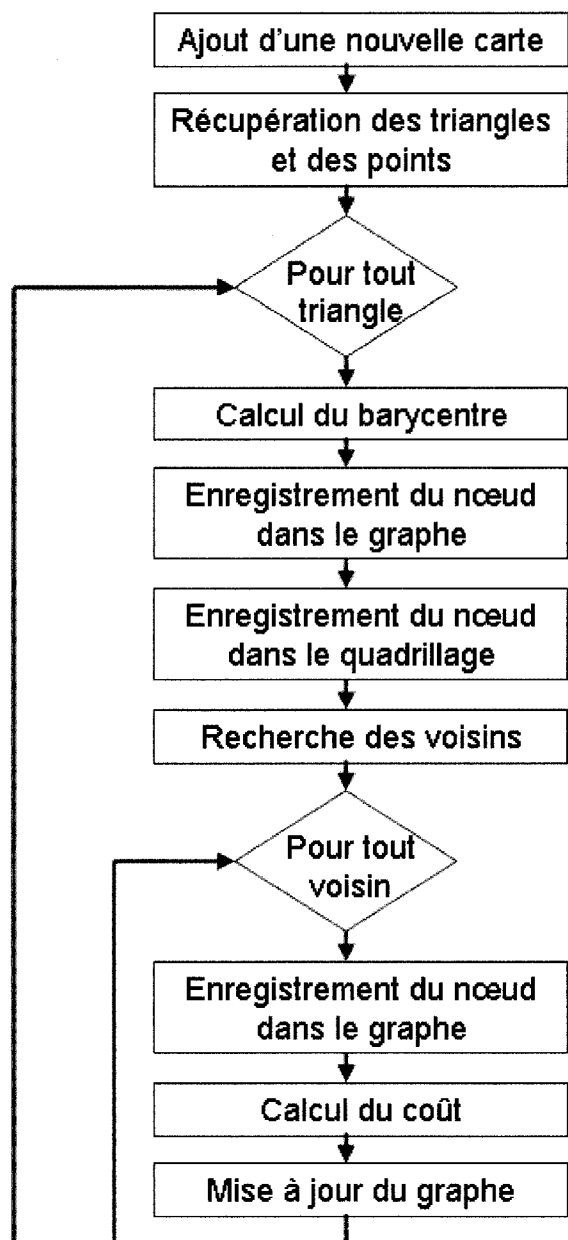
FIG. 2.2 Algorithme de réalisation du graphe
