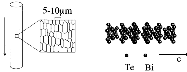
Figure 1.10: Procédé d'extrusion et structure cristalline du \text{Bi}_2\text{Te}_3 .
