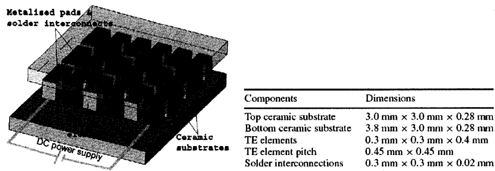
Figure 1.27 : Design et dimension du module étudié [18].
