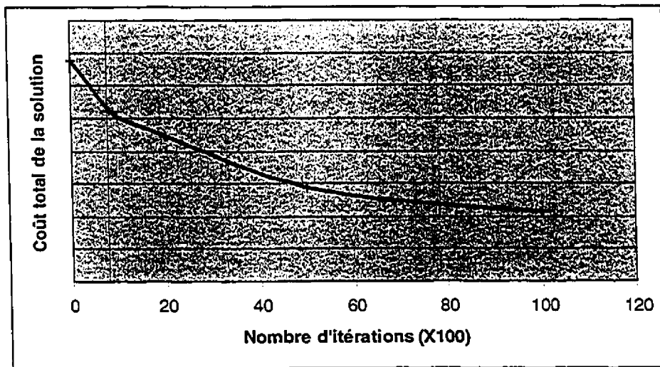
Figure 5.12 Impact du nombre d'itérations sur la qualité de la solution
