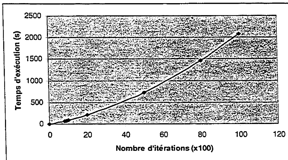
Figure 5.13 Temps de réponse et nombre d'itérations
