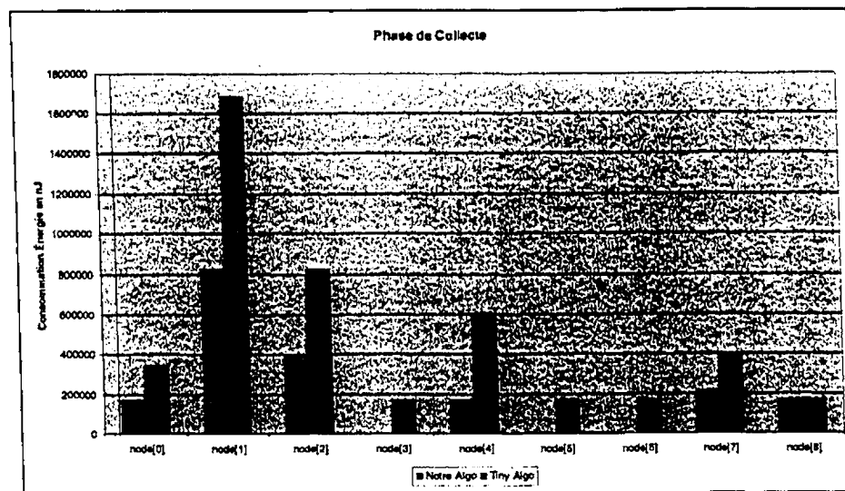
Figure 5.2 Consommation d'énergie : Phase de collecte
