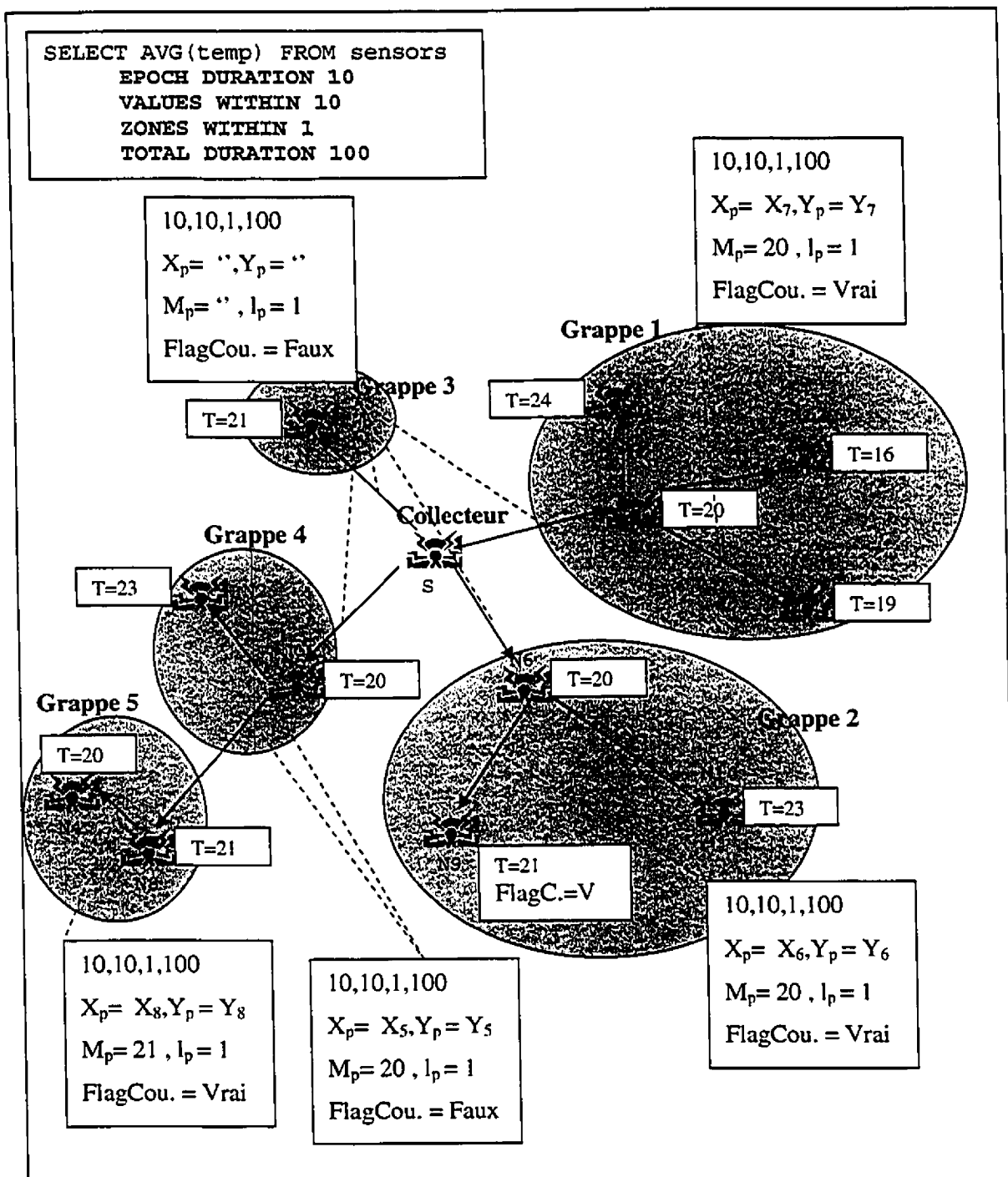
Figure 3.11 Exemple de formation de grappes
