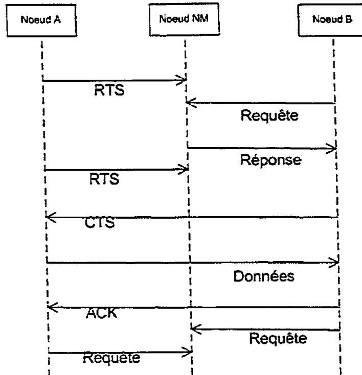
Figure 2.2 Échange de messages dans le protocole Nœud Médiateur
