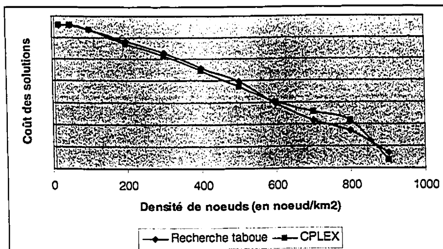
Figure 5.16 Comparaison des coûts des solutions recherche taboue et CPLEX : Topologie aléatoire
