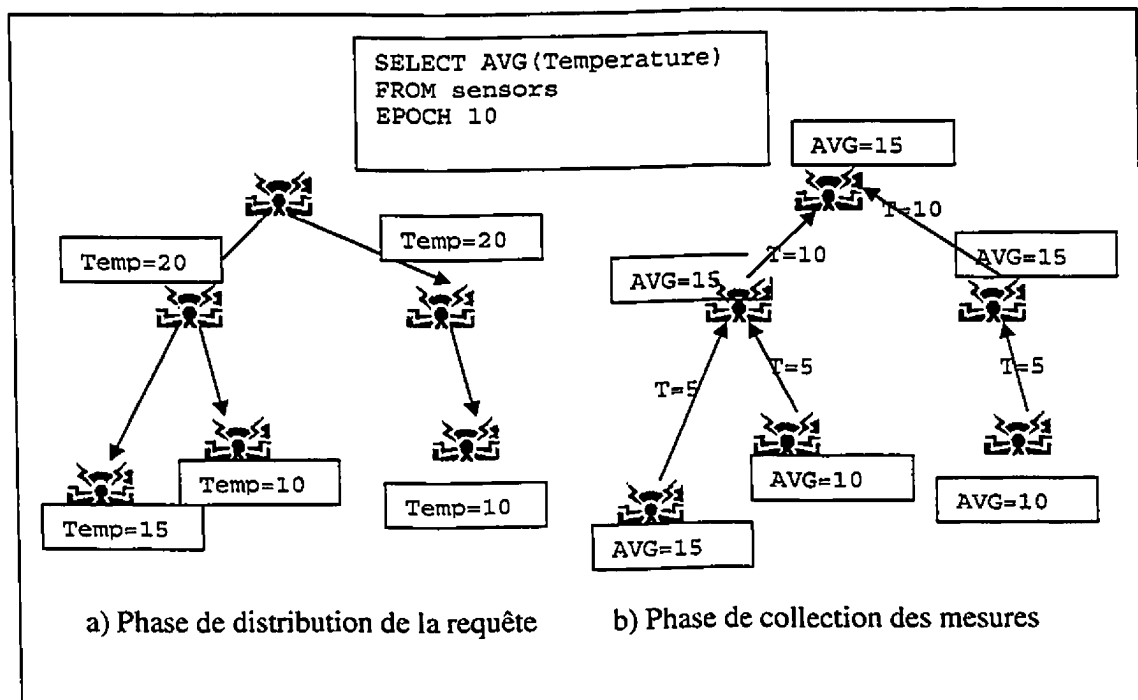
Figure 3.6 Phases de l'agrégation TAG
