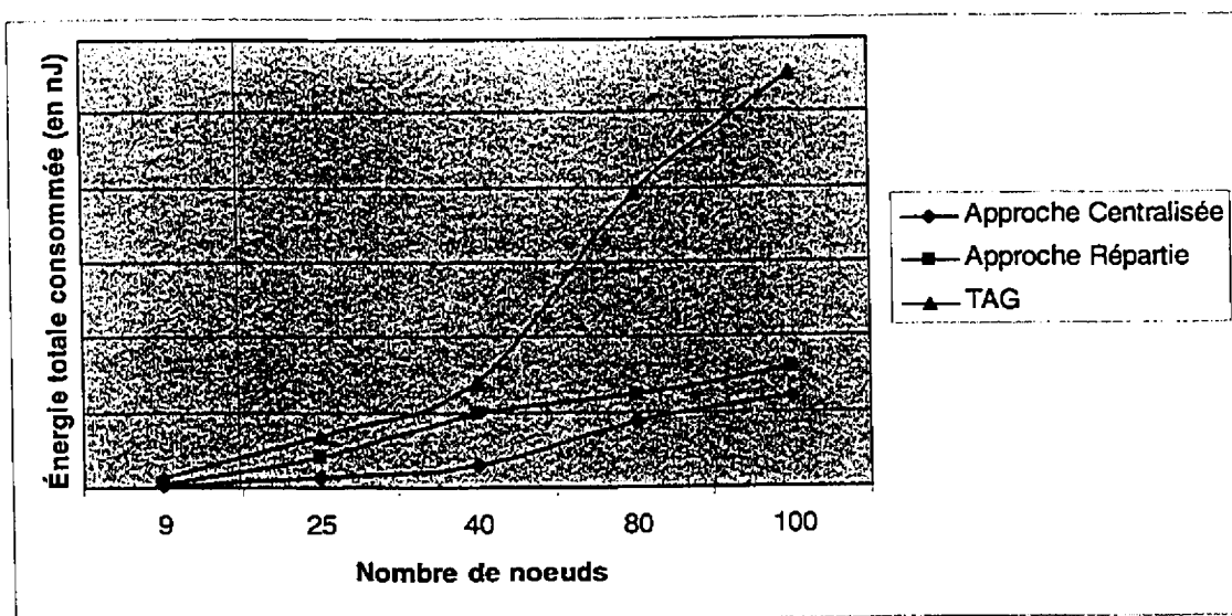
Figure 5.20 Comparaison des énergies totales consommées dans les deux approches
