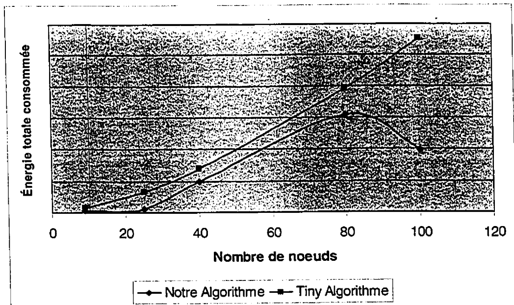
Figure 5.6 Impact du nombre de nœuds sur la consommation d'énergie
