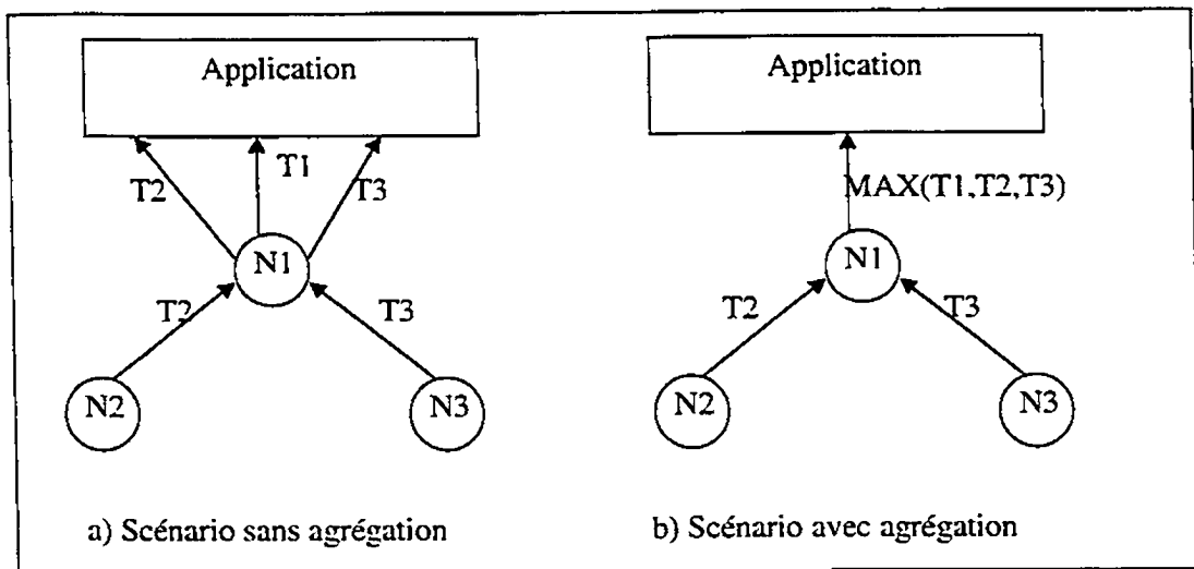
Figure 3.3 Principe de l'agrégation
