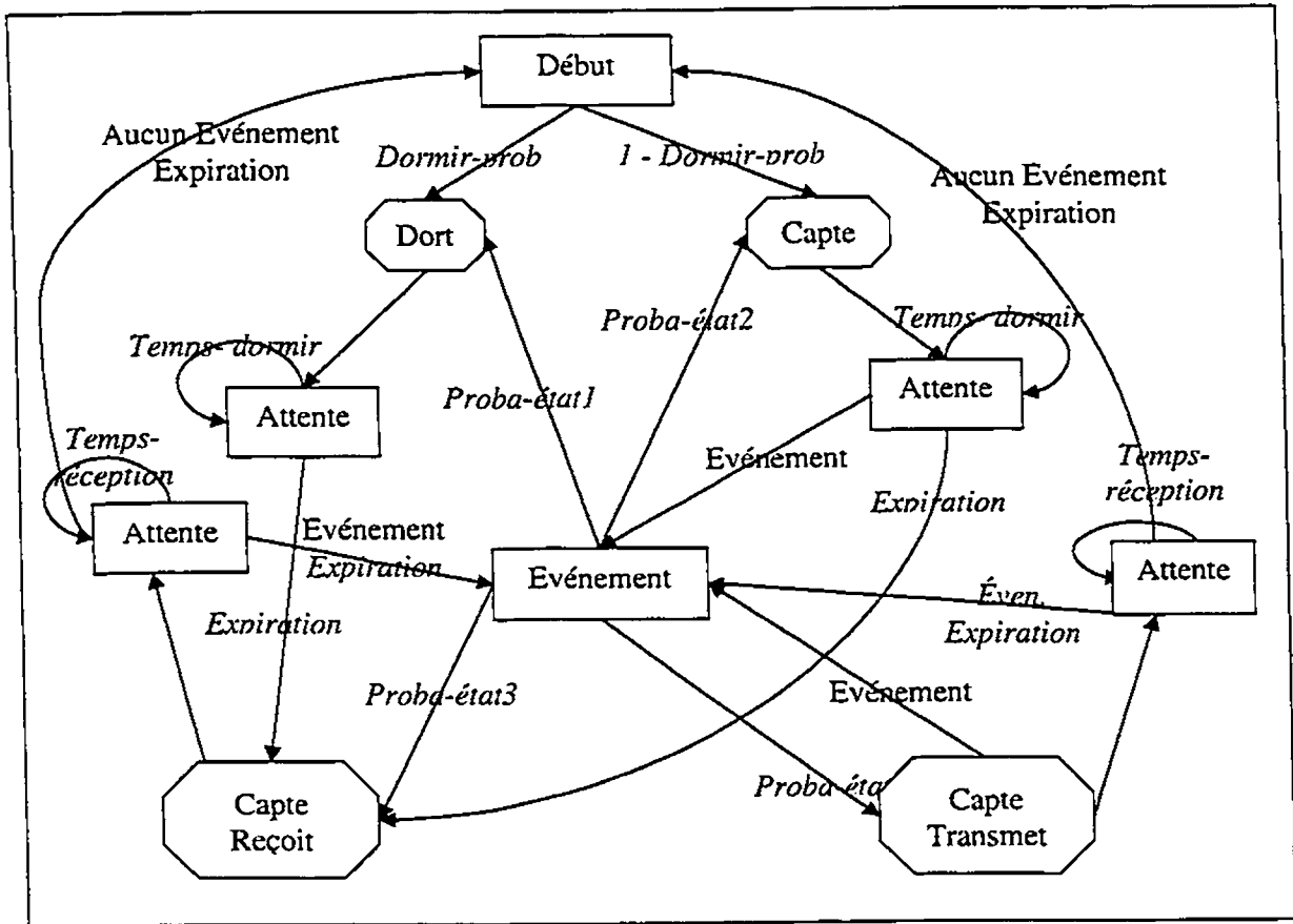
Figure 2.4. Modèle amélioré du comportement des nœuds
