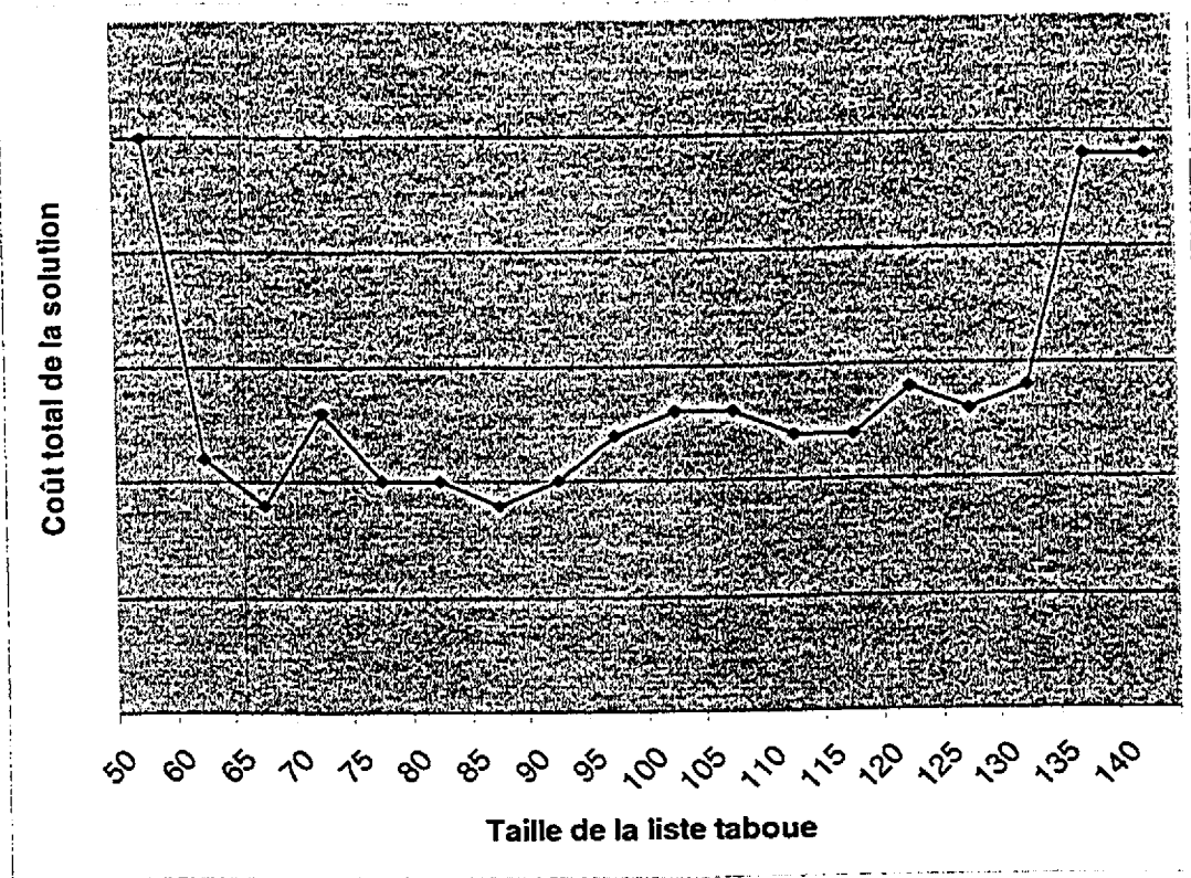
Figure 5.11 Impact de la taille de la liste taboue
