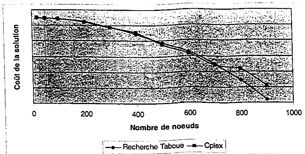
Figure 5.14 Comparaison des coûts des solutions recherche taboue et CPLEX : Topologie en carré
