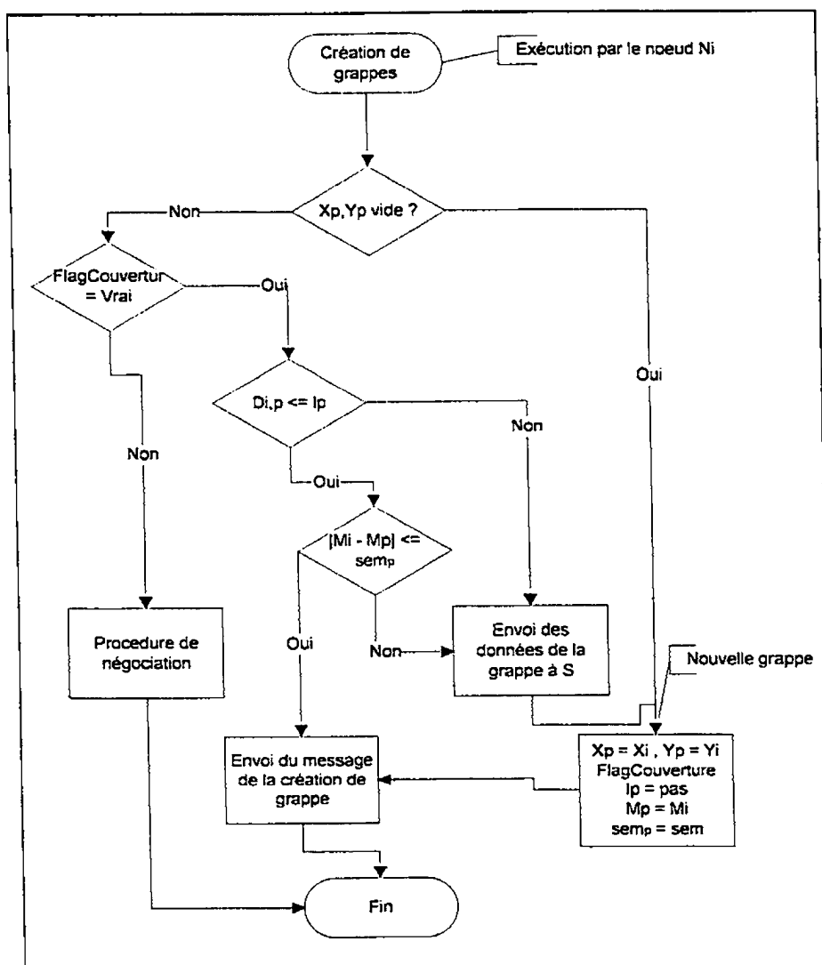
Figure 3.10 Organigramme de l'algorithme de création de grappes
