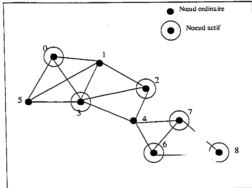
Figure 5.8 Graphe G' et solution initiale du réseau de validation
