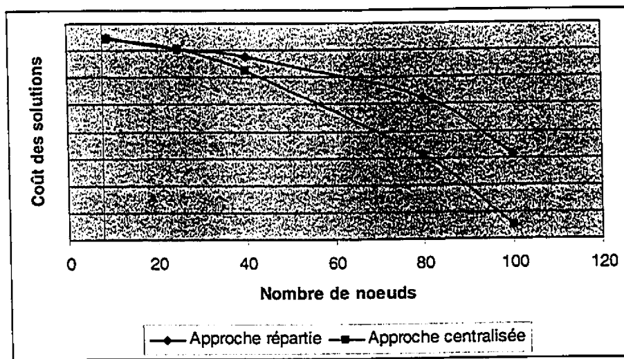
Figure 5.18 Coût des solutions pour les deux approches répartie et centralisée
