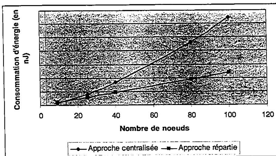
Figure 5.19 Comparaison des énergies consommées pour former les grappes dans les deux approches
