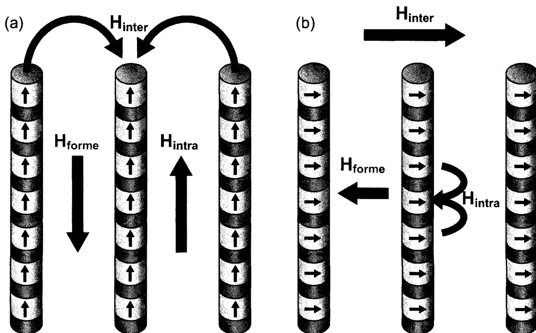
Figure 6.3 : Provenance des champs d'interaction dans les réseaux de nanofils multicouches. (a) Direction axiale (b) Direction transverse
