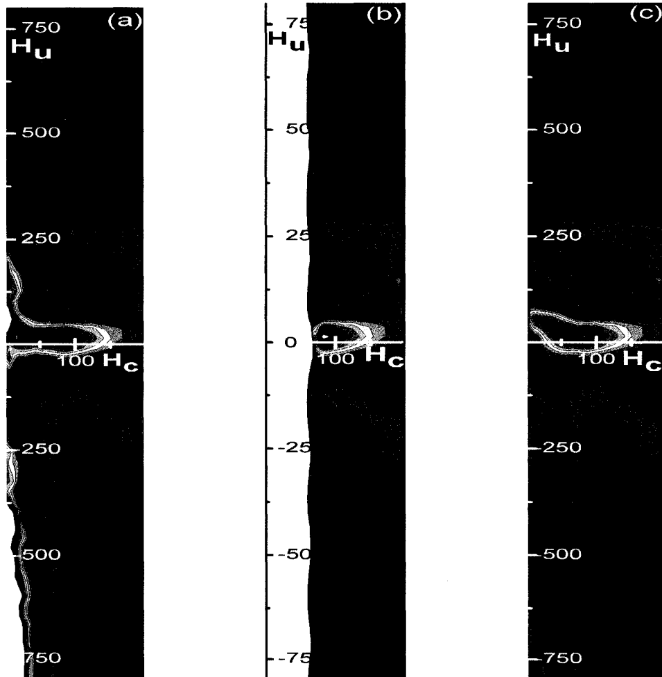
Figure 2.9 : Diagrammes FORC (a) tronqué (b) étendu et (c) extrapolé
