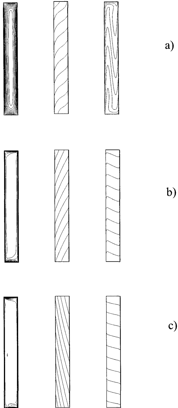
Figure 5.10 Lignes de courant(gauche), isothermature(milieu), isoconcentration(droite) (cas Neumann) pour R_T = 50 , Le = 10 , a = 1 , \eta = 0.5 et A = 8 ; a) N = 0 , b) N = 10 , et c) N = -10
