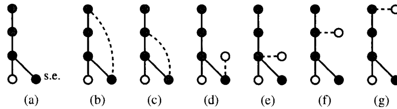
Figure 2.15 (a) Un graphe et (b)-(g) quelques uns des prolongements de ce graphe par GSPAN. Les sommets noircis forment le chemin extrêmeal se terminant par le sommet extrêmeal (s.e.). Les arêtes en pointillé représentent les prolongements du graphe.
