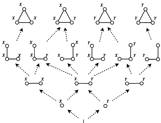
Figure 2.4 L'espace de recherche contenant tous les sous-graphes connexes d'au plus trois sommets et deux étiquettes de sommet.
