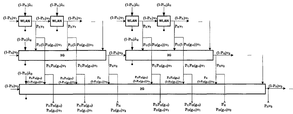
FIGURE 3.5 Trafic d'appels dans un RMHPG
