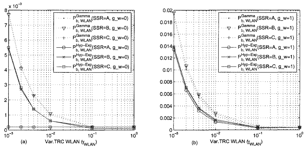
FIGURE 3.9 Probabilité de blocage WLAN en fonction de la variabilité du TRC
